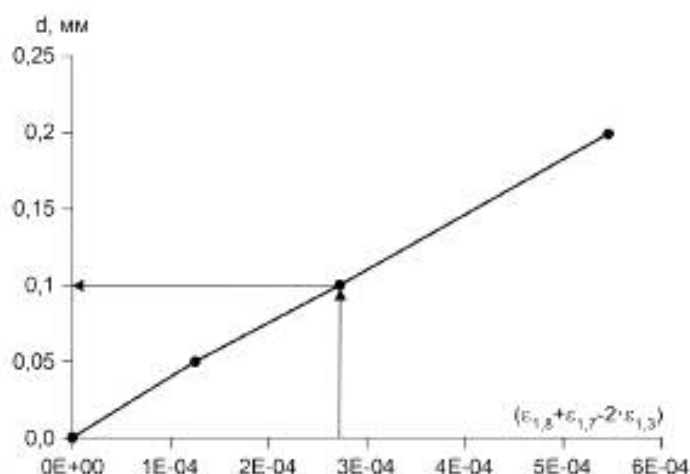
Рисунок 7 — График дефекта типа S
