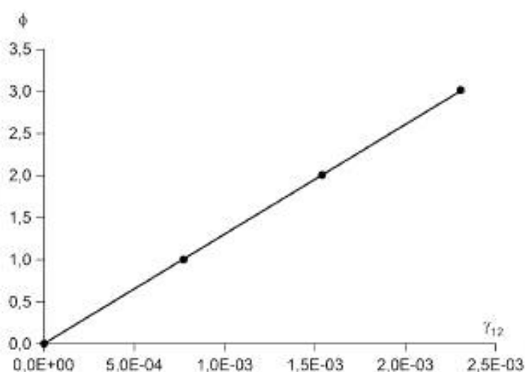
Рисунок 5 — Карта 1. Дефект скручивания
