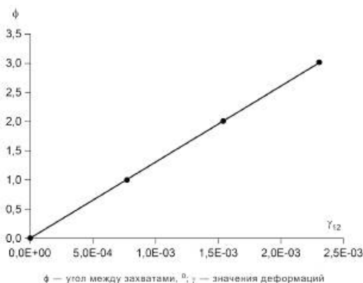
Рисунок 5 — График дефекта кручения
