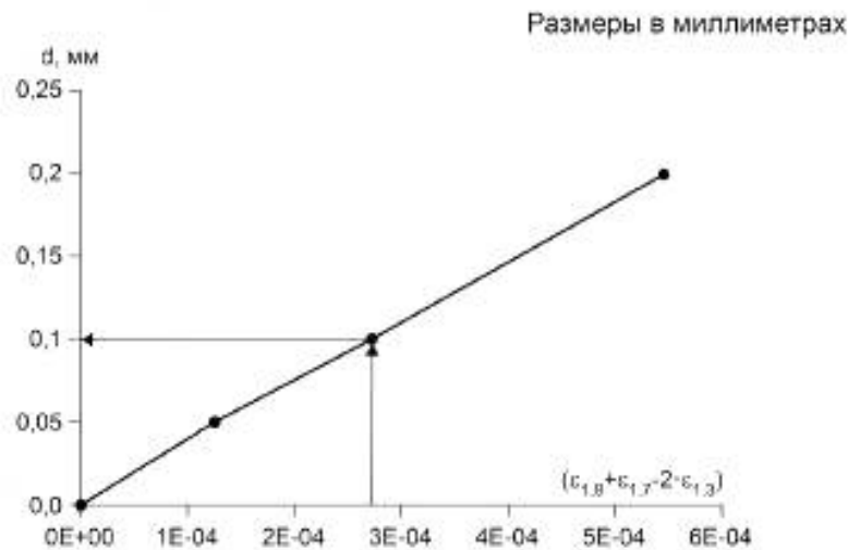
Рисунок 7 — Карта 3. S-дефект
