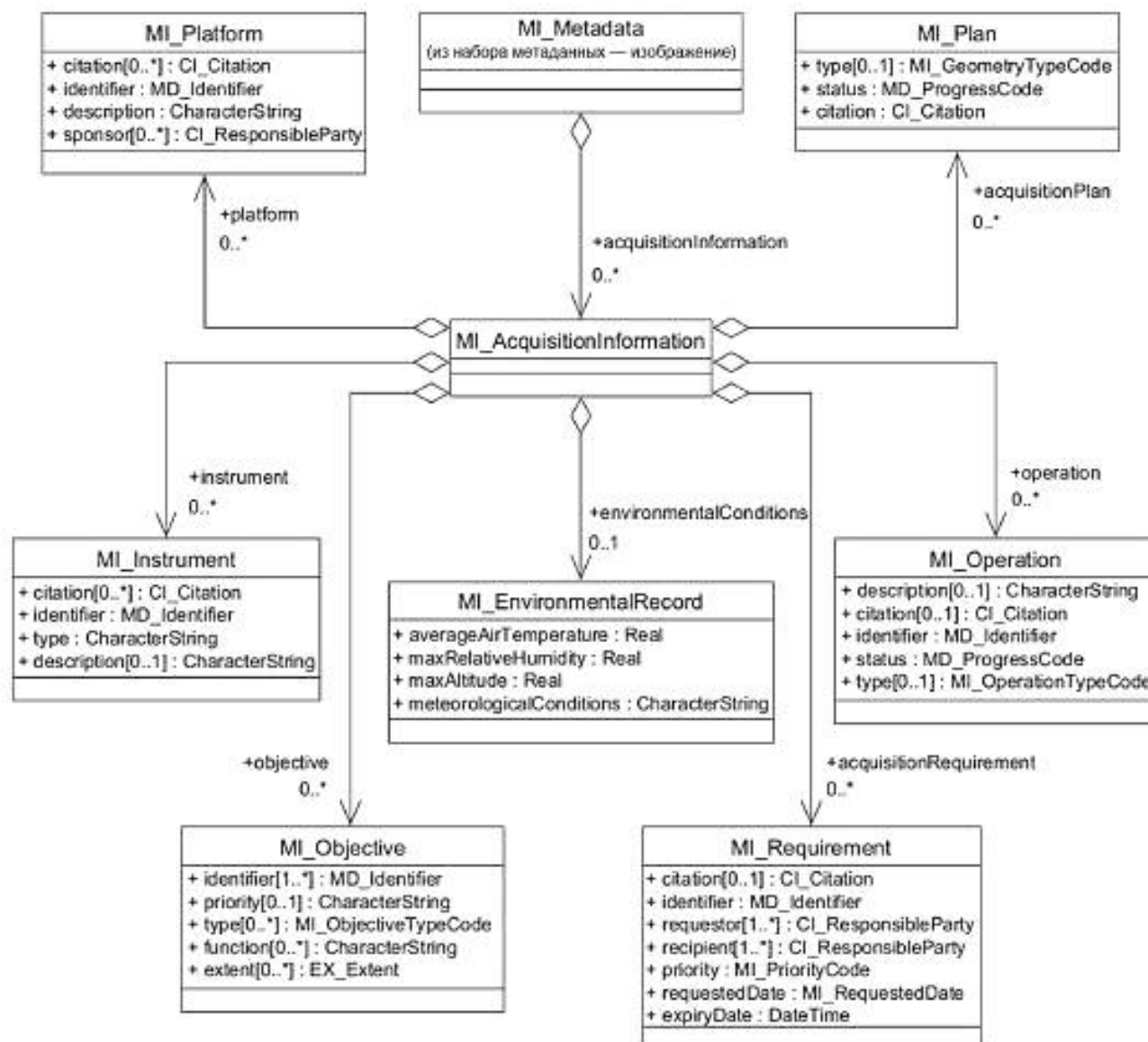
Рисунок A.8 — Обзор сбора
