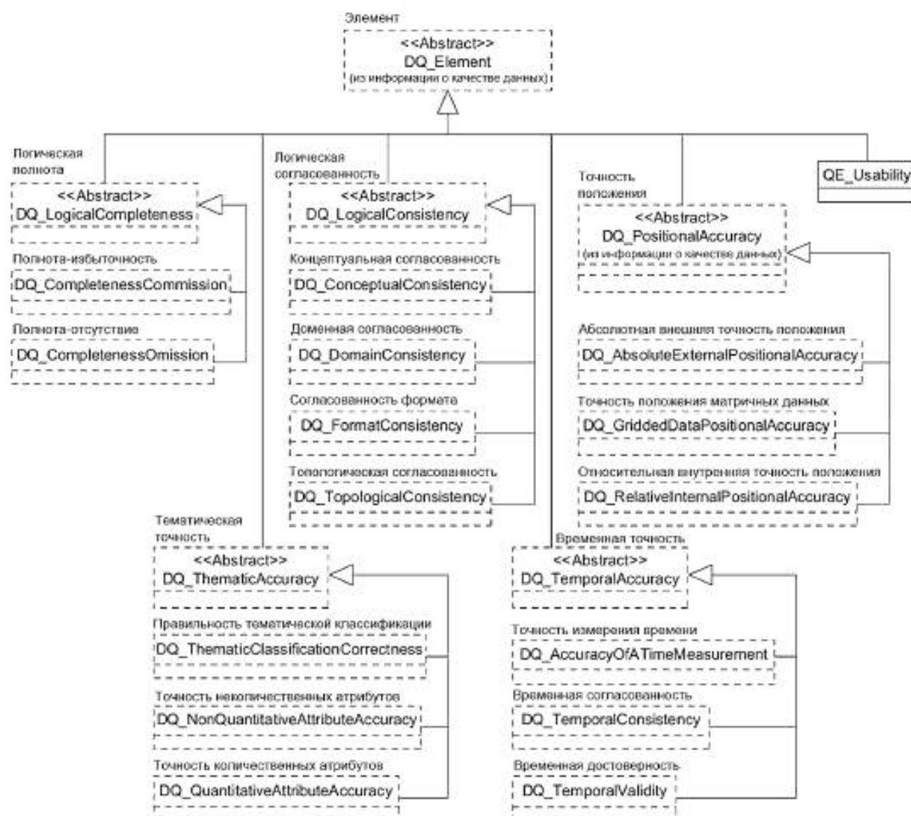
Рисунок A.4 — Расширение подклассов качества данных
