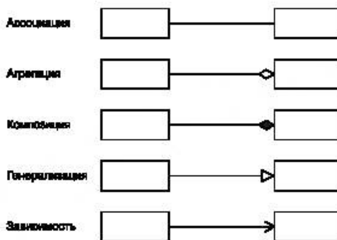
Рисунок 1 — Символика UML
