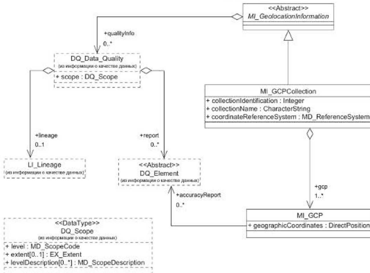
Рисунок A.6 — Качество опорных точек
