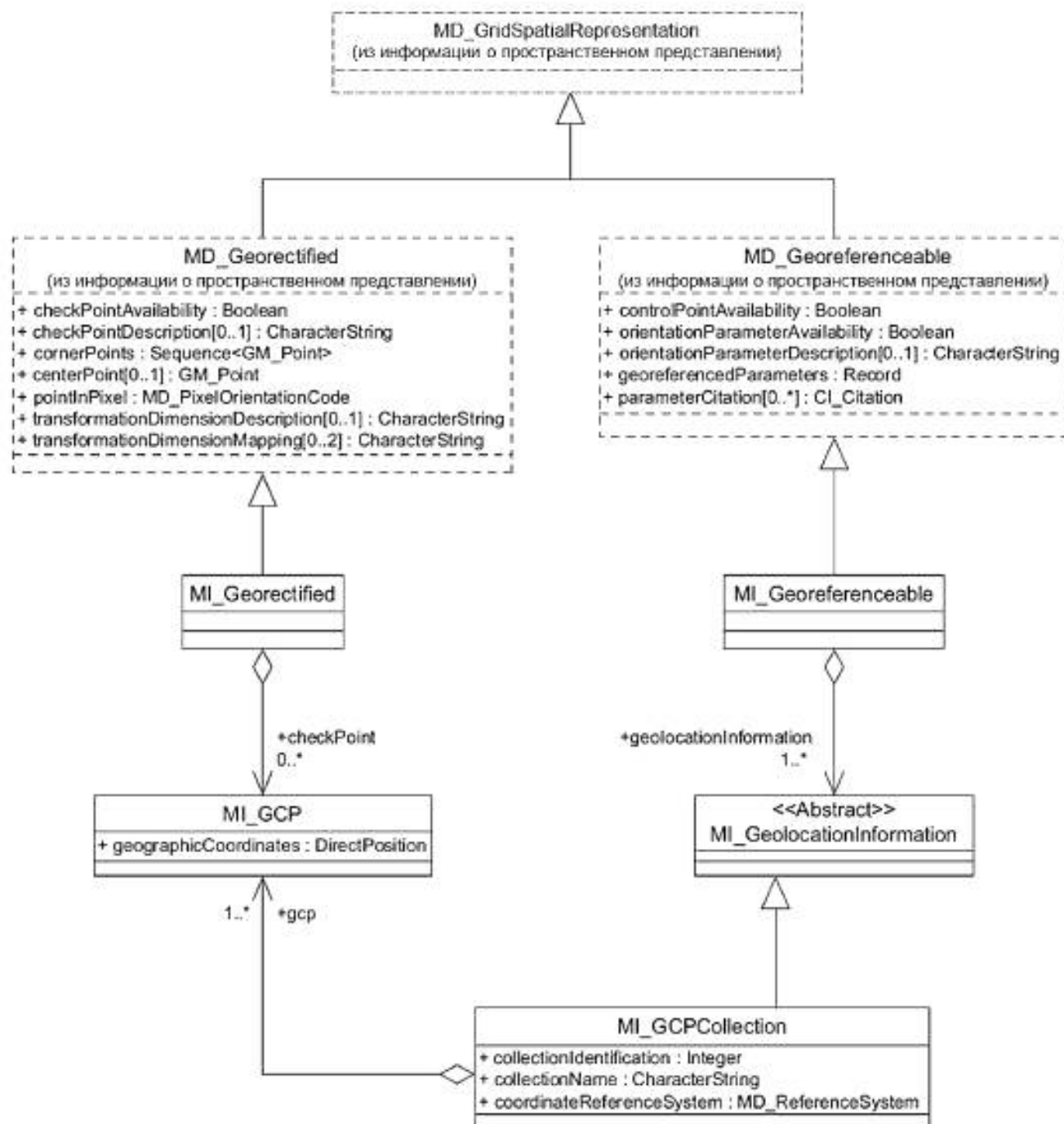
Рисунок A.5 — Информация о пространственном представлении
