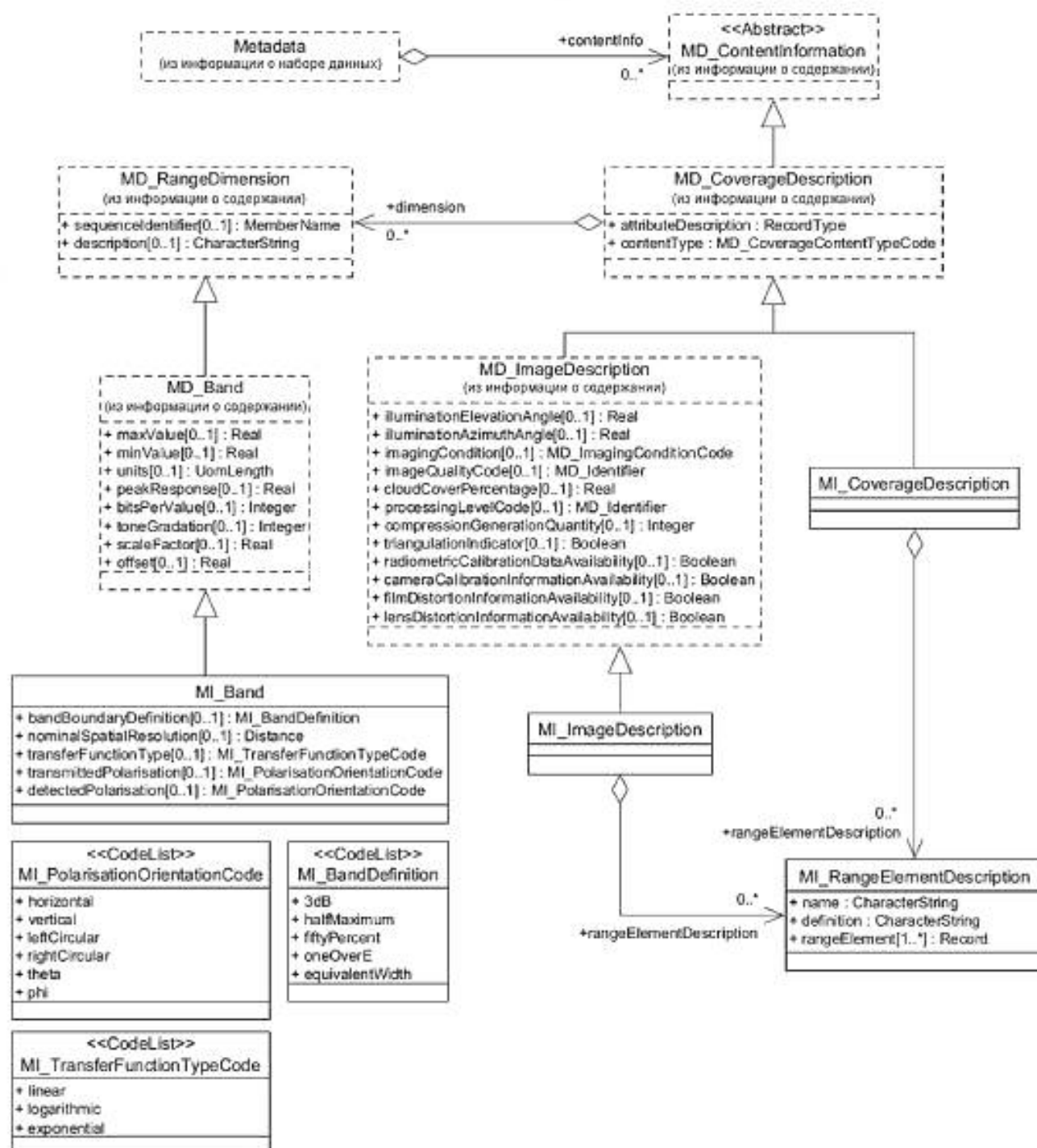
Рисунок А.7 — Информация о содержании 1)
