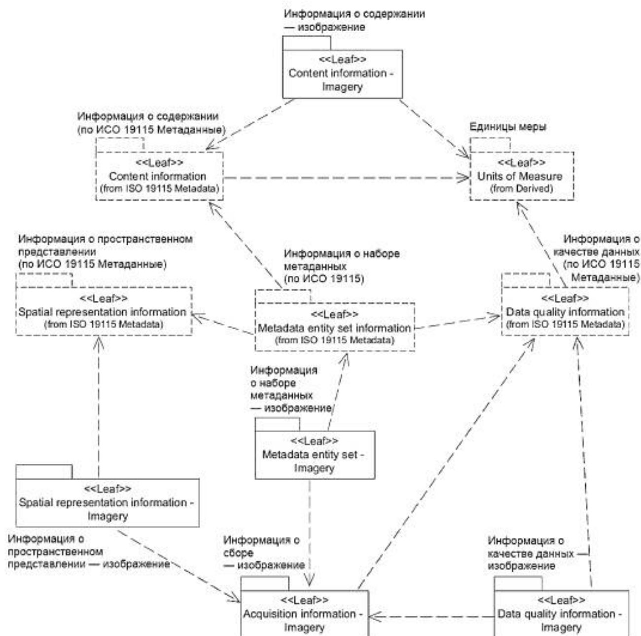
Рисунок 3 — Пакеты метаданных
