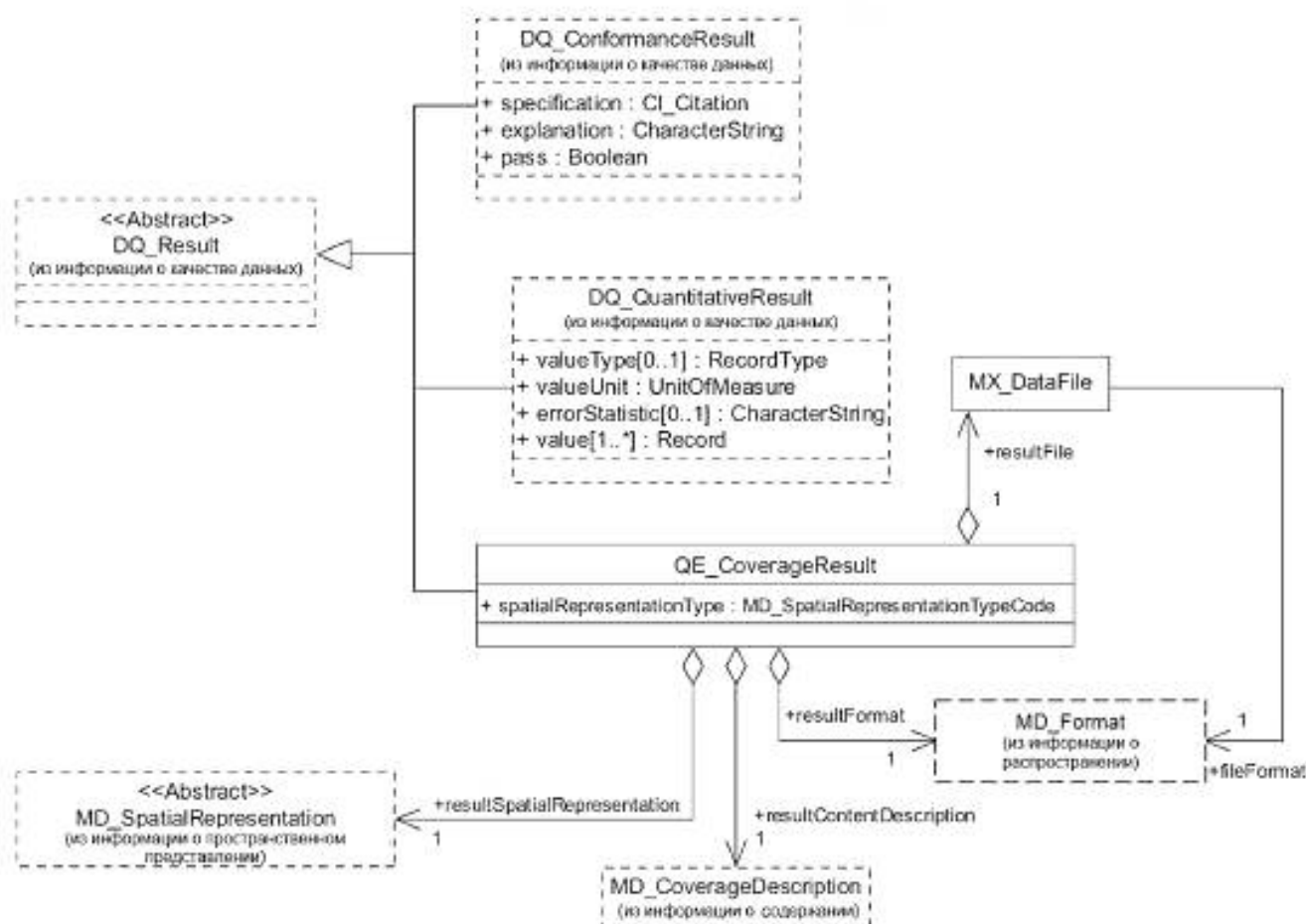
Рисунок А.2 — Результат качества данных
