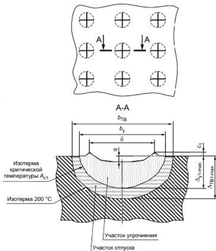
Рисунок 2 — Конструктивные элементы локальной зоны упрочнения при ЗКУ, выполненной неподвижным источником теплоты
