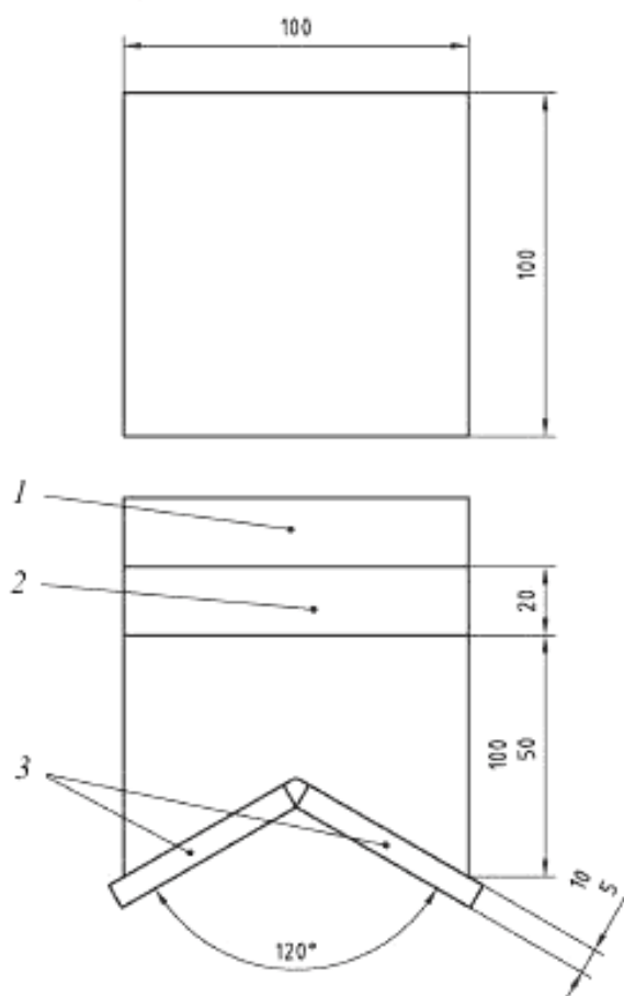
Рисунок 3 – Брусок с V-образным вырезом
