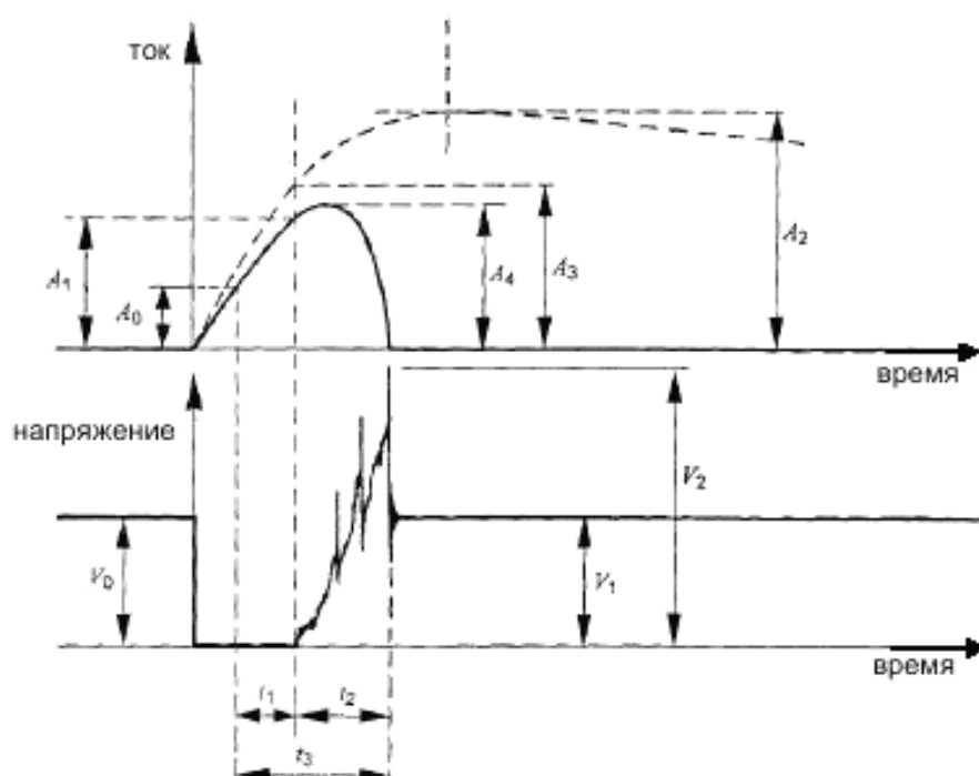
Рисунок В.3 – Осциллограмма, соответствующая выключению до достижения током максимального значения (для токоограничивающего автоматического выключателя)
