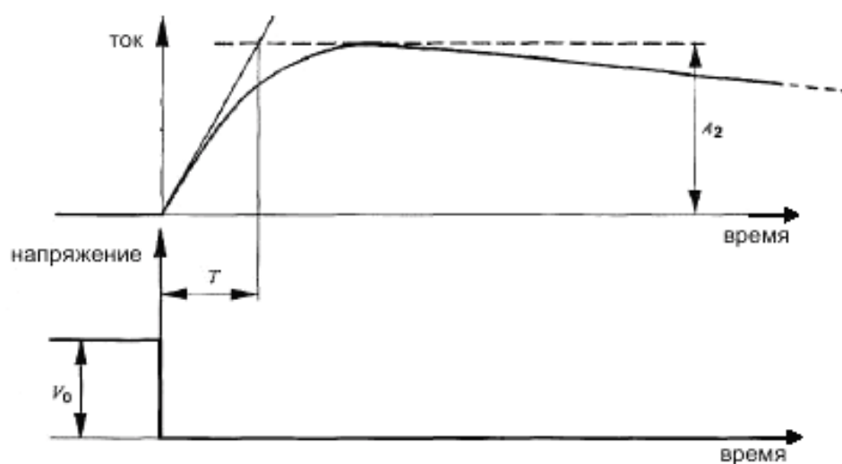
Рисунок В.1 – Калибровка испытательной схемы для получения ожидаемого пикового тока включения
