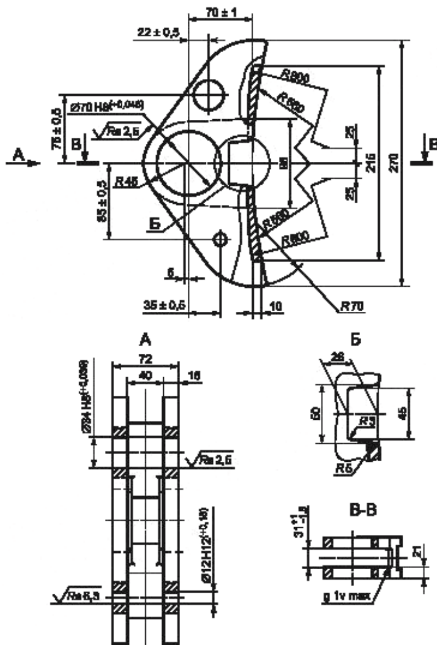
Рисунок 10 — Башмак типа Б
