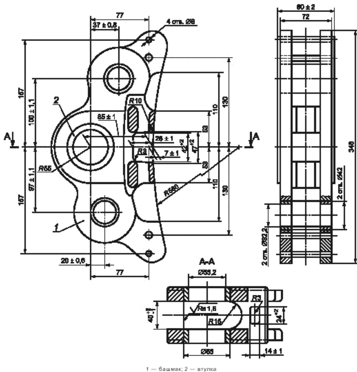
Рисунок 5 — Башмак типа 2 — Исполнение 1
