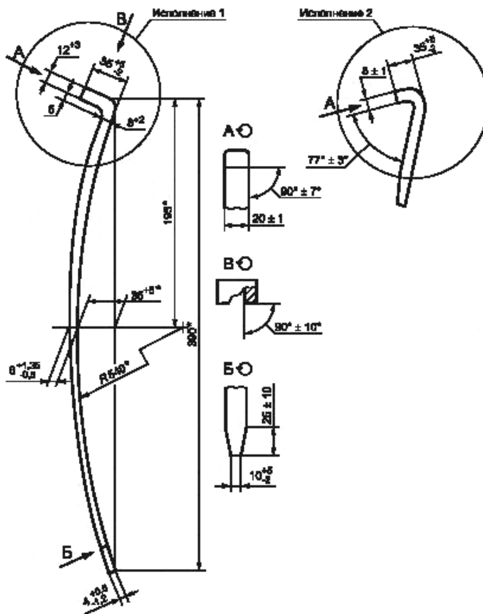
Рисунок 11 — Чека типа 1
