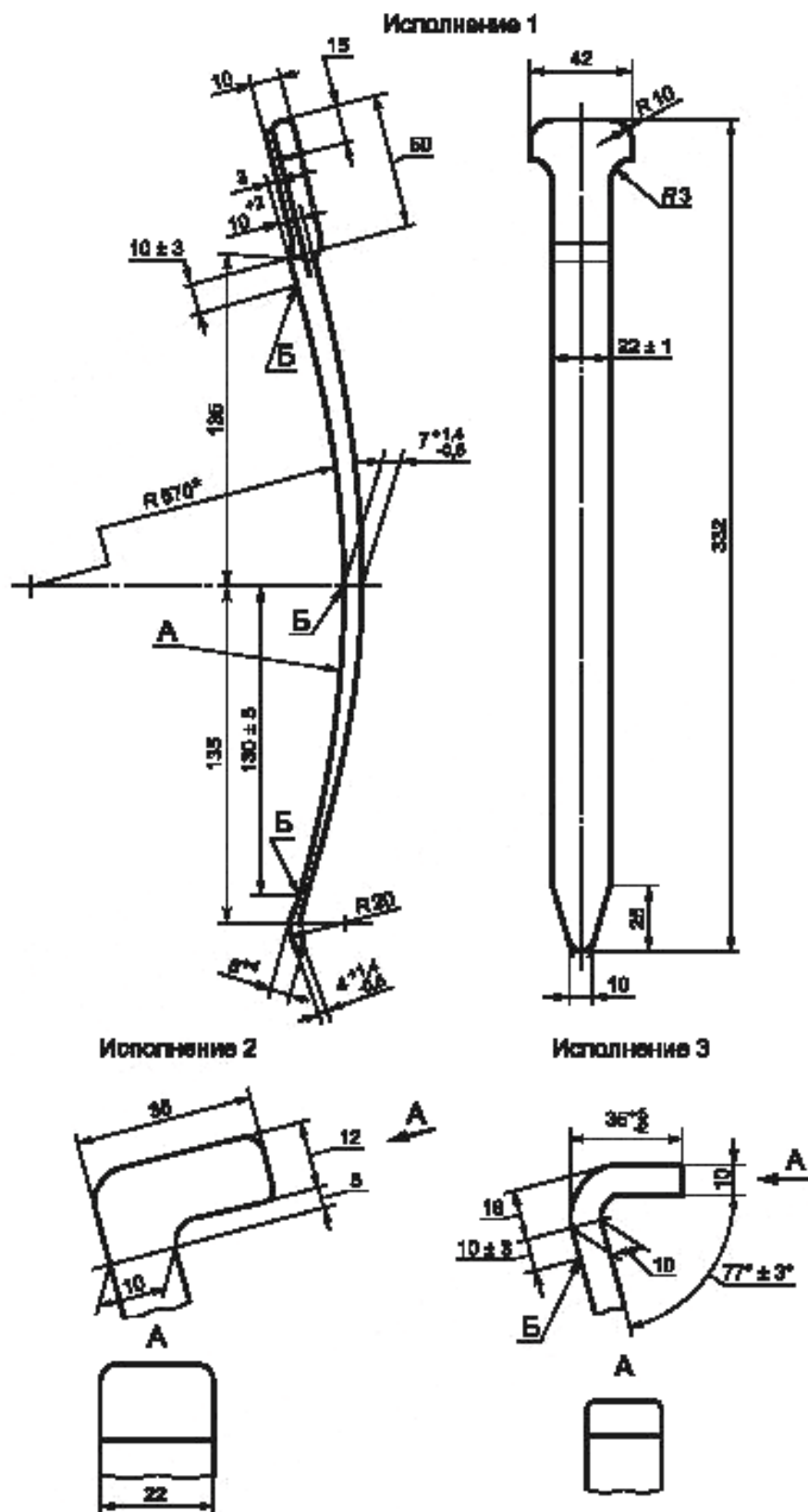
Рисунок 12 — Чека типа 2
