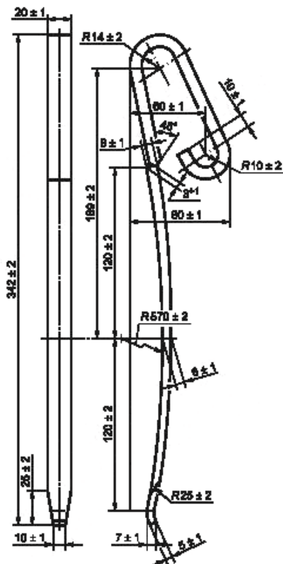
Рисунок 13 — Чека типа 3
