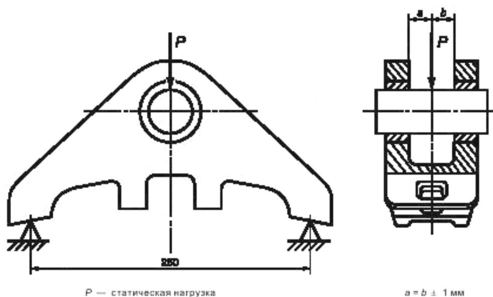
Рисунок В.1 — Схема испытания башмака статической нагрузкой
