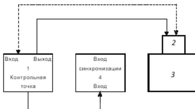
1 – электронный блок дефектоскопа; 2 – преобразователь; 3 – калибровочный образец; 4 – осциллограф
