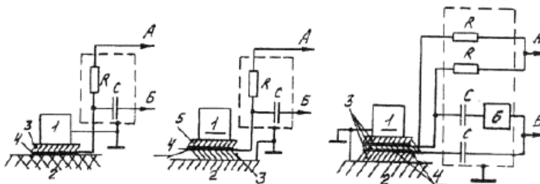
1 — проверяемые ПЭП; 2 — акустическая нагрузка; 3 — конденсаторная бумага СКОН-ОВН толщиной 4 — 15 мкм или целлофановая пленка толщиной не более 22 мкм; 4 — алюминиевая фольга толщиной 5 — 1,2 мкм; 5 — лавсановая пленка ПЭТФ толщиной 10 — 15 мкм; 6 — фазоинвертор; R — резистор МЛТ-0,25 — 1 МОм; C — конденсатор К73-400 В-0,1 мкФ
