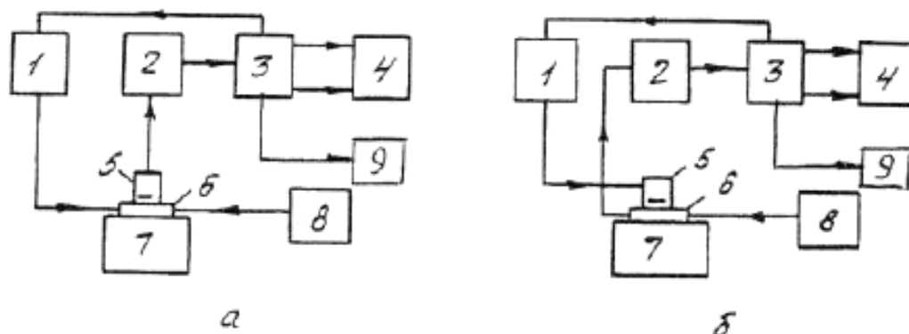
1 — усилитель мощности; 2 — усилитель напряжения (рисунок 40а), усилитель тока (см. рисунок 40 б); 3 — измеритель АЧХ; 4 — графопроектор; 5 — проверяемый ПЭП; 6 — диэлектрический преобразователь; 7 — акустическая нагрузка; 8 — источник напряжения; 9 — частотомер
