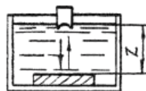
Рисунок 6 — Иммерсионные ПЭП.
