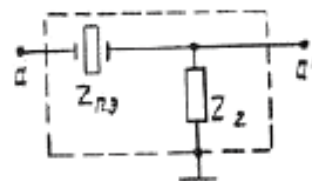
Z_{п.э.} – проверяемый ПЭП; Z_2 – электрическая нагрузка
