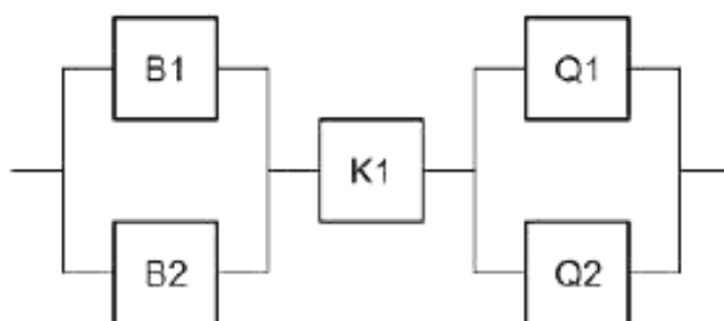
Рисунок 2 – Блок-диаграмма подсистемы, связанной с безопасностью
