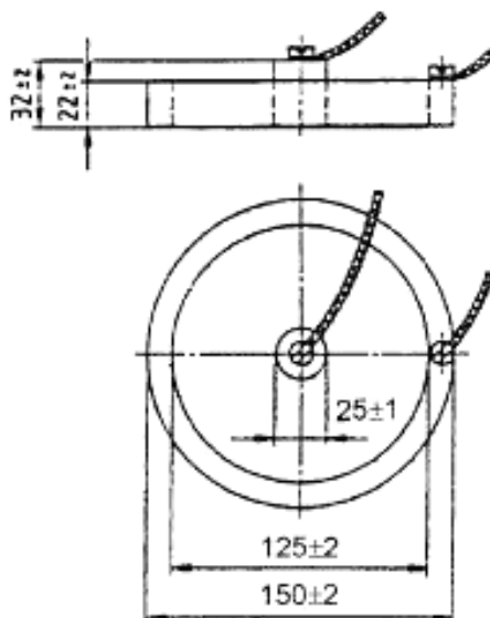
Рисунок Б.1 – Схема размещения электродов при испытании
