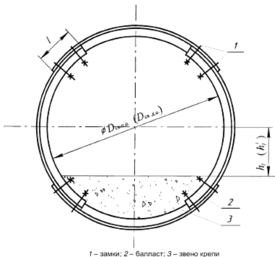
Рисунок 1 – Схема кольцевой крепи
