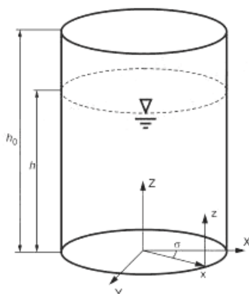
Рисунок 2 — Модель цилиндрического сосуда с жидкостью
