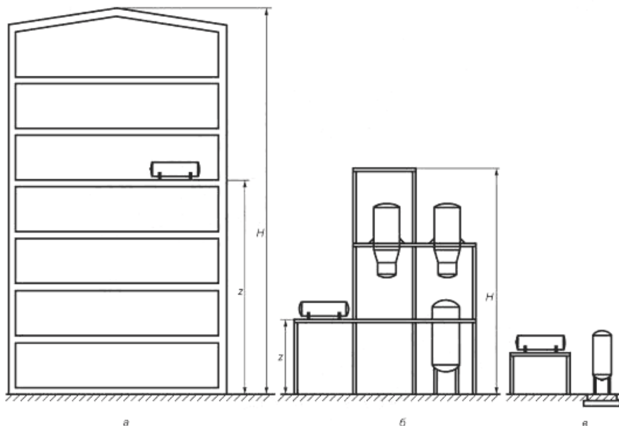
Рисунок 1 — Варианты установки сосуда
