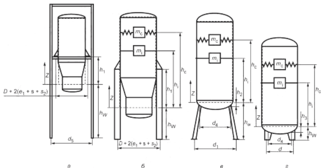
Рисунок 8 — Вертикальный сосуд
