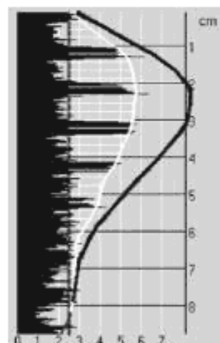
Рисунок А.21б) Ожидаемая огибающая кривая VDR
