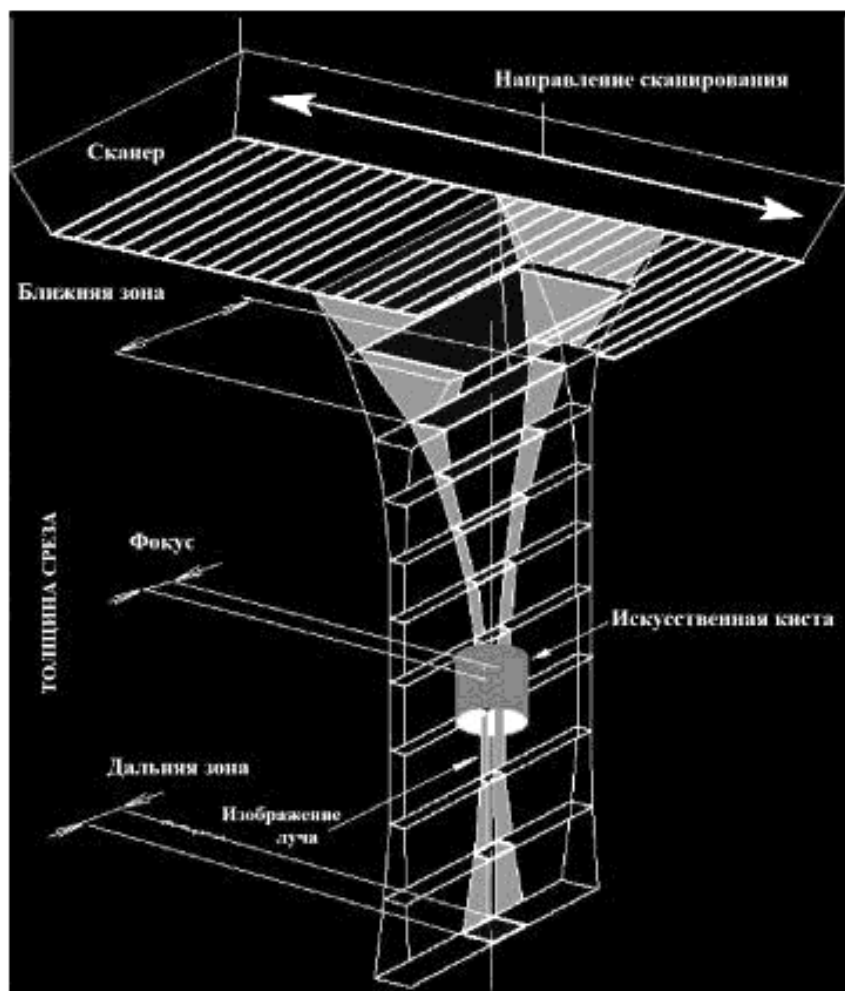
Прохождение ультразвукового пучка через искусственные кисты в фантоме
