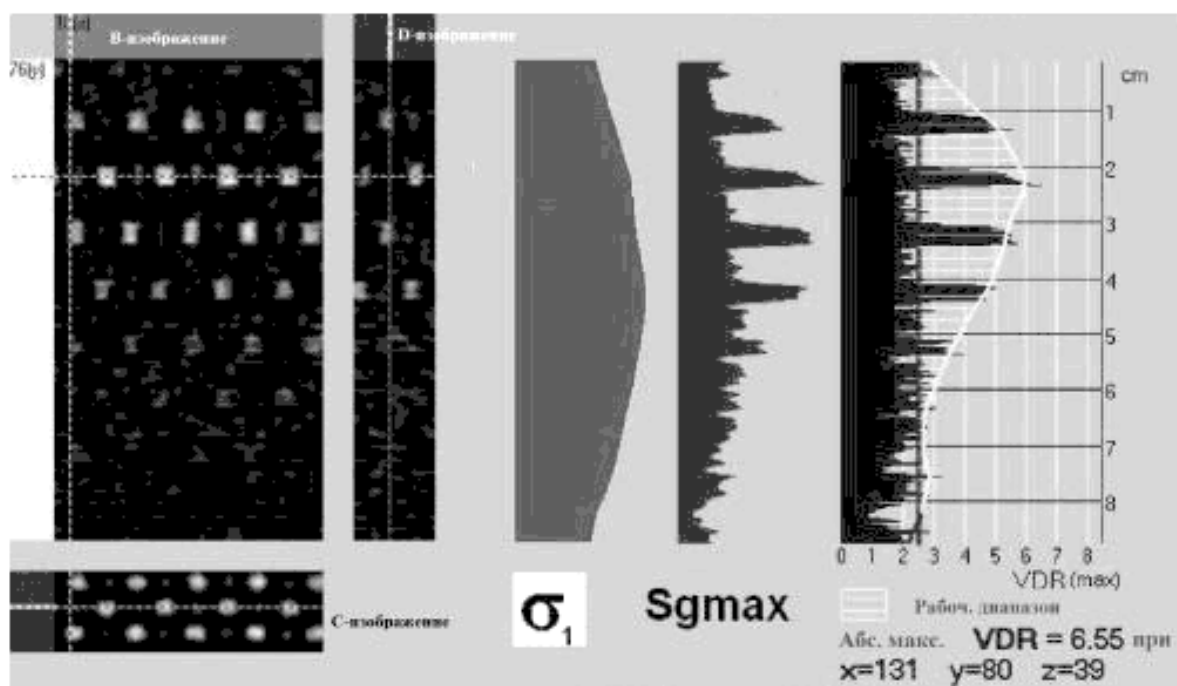
Рисунок А.10 – В-, С-, D- плоскости
