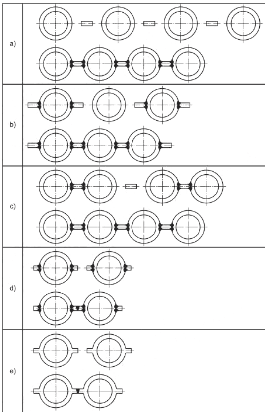
Рисунок С.1 — Примеры конструкций мембранных панелей
