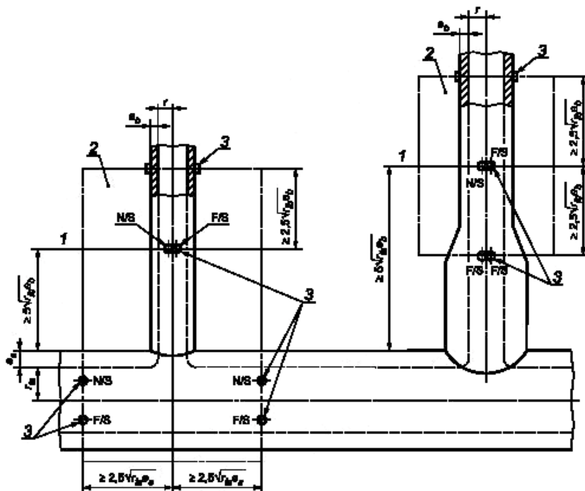
1 — место сварки; 2 — зона нагрева; 3 — термодары
