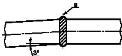
a — Середина сварного шва
