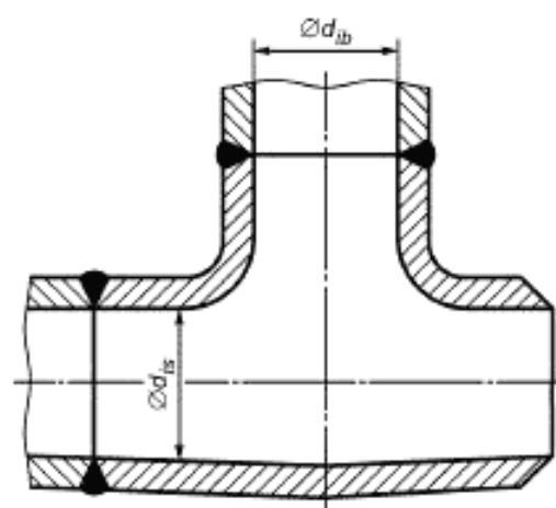
Рисунок 8.1-5 — Ковано-штампованный штуцер
