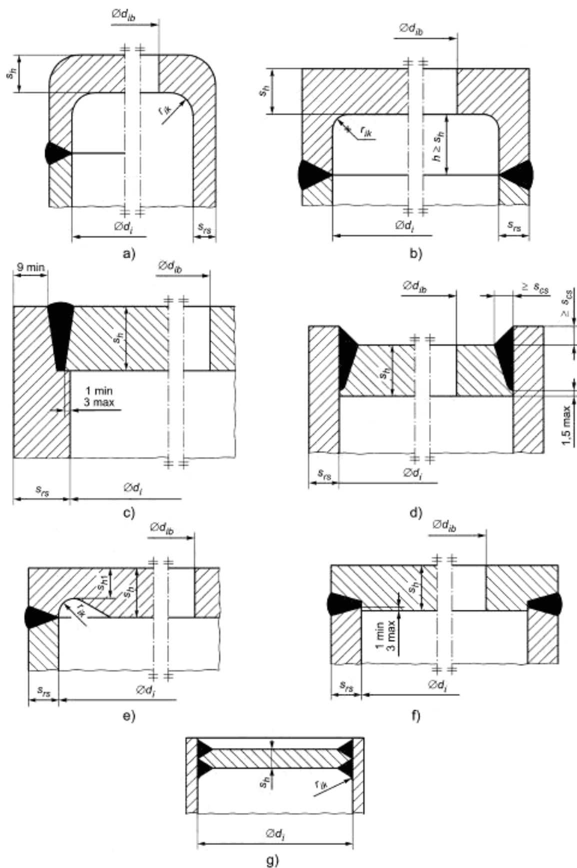
Рисунок 10.3-1 — Плоские торцевые участки без анкерных связей
