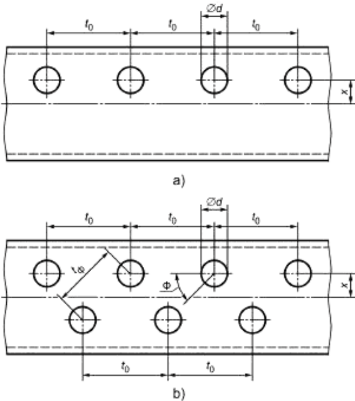
а) отверстия, расположенные на одной линии; б) отверстия, расположенные на двух параллельных линиях
