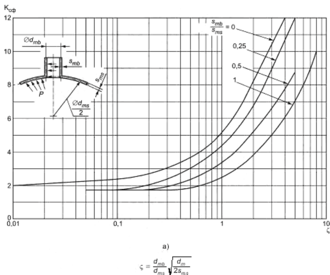
Рисунок 13.4-7 — Коэффициент концентрации напряжений K_{сф} для сферических оболочек, лист 1
