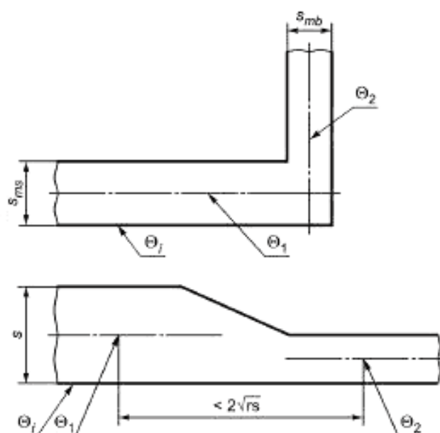
Рисунок 13.3-1 — Определение \Delta\Theta
