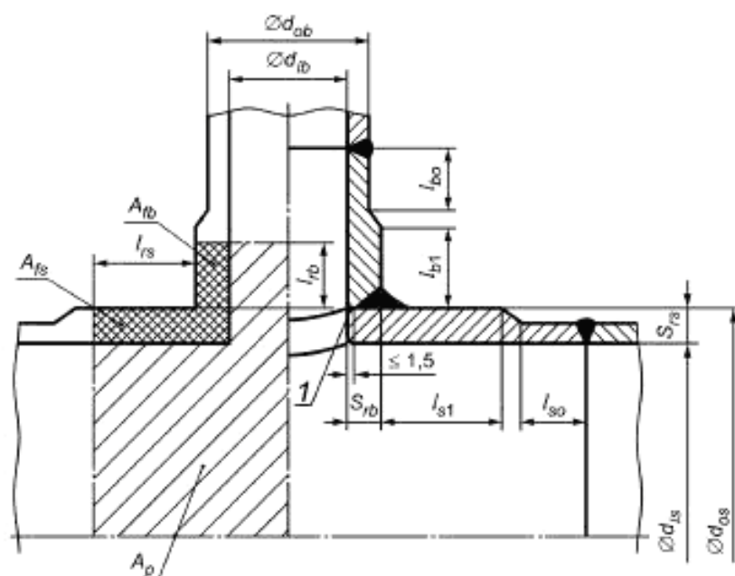
Рисунок 8.1-3 — Усиление приваренным штуцером
