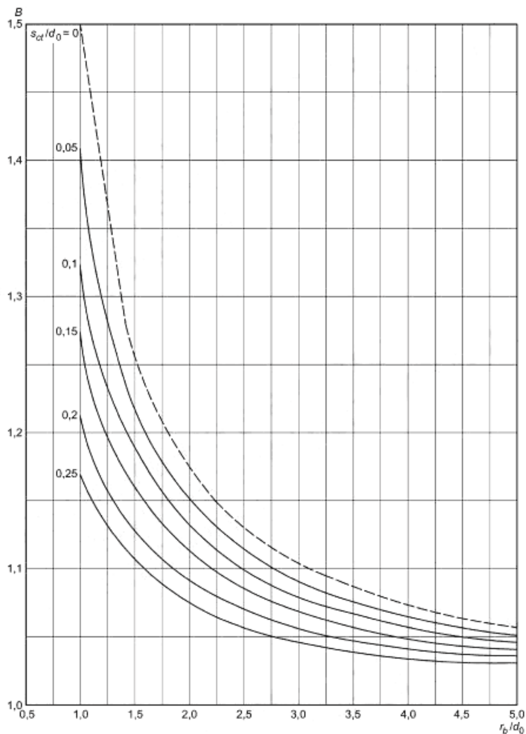
Рисунок А-6 — Расчетный коэффициент B для расчета гибов со стенками равной толщины ( s_n = s_{do} ) труб с номинальным наружным диаметром
