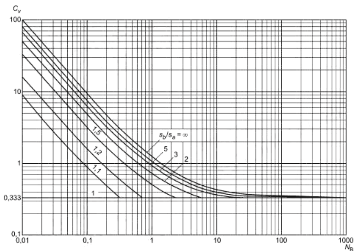
Рисунок 13.3-6 — Коэффициент C_v
