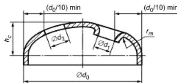
Рисунок 10.2-5 — Отверстия в днищах
