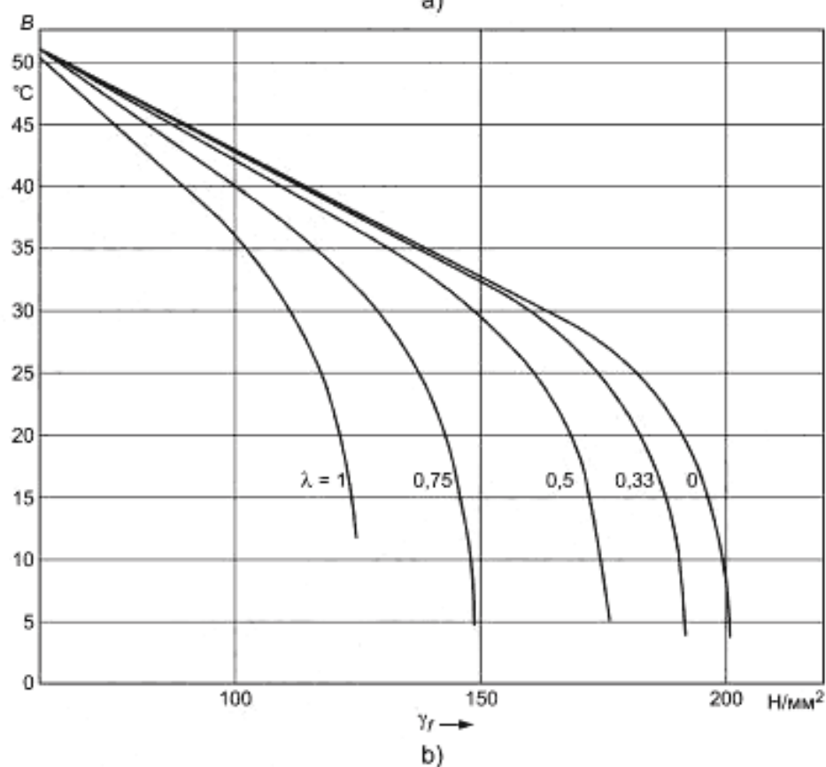
Рисунок 13.3-3 — Значения B для аустенитных нержавеющей сталей
