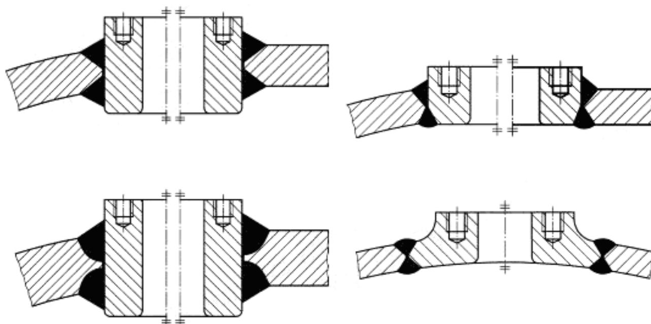
Рисунок 8.4-1 — Типовые примеры приварки усиливающих элементов
