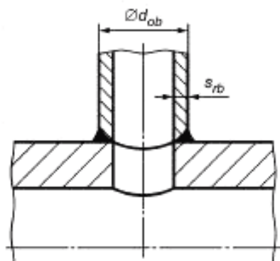
Рисунок 8.2-1 — Соединение трубы с основным корпусом
