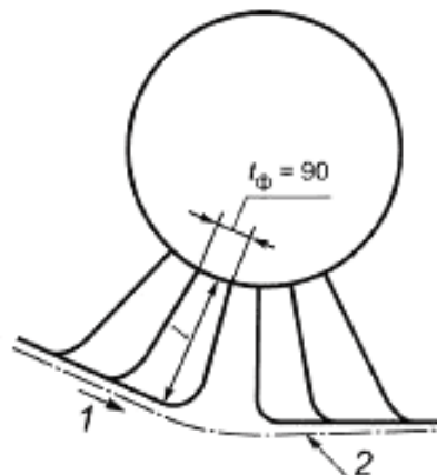
1 — поток дымового газа 2 — граница потока дымового газа Рисунок 6.1-4 — Элементы, защищенные близко расположенными трубами
