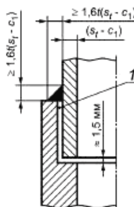
Рисунок 8.5-2 — Соединение на сваренной муфте и резьбовое соединение
