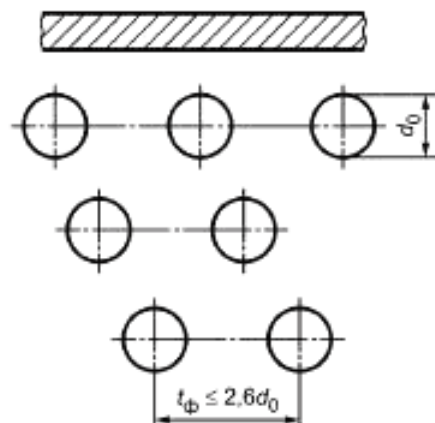
Рисунок 6.1-3 — Элементы, защищенные тремя рядами труб
