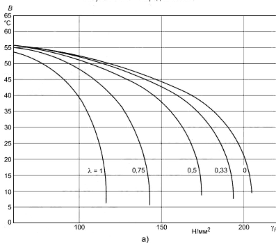
Рисунок 13.3-2 — Значения \Delta\Theta для углеродистых или ферритных легированных сталей, лист 1
