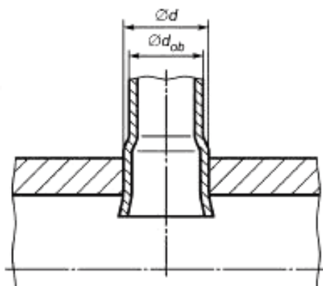
Рисунок 8.2-2 — Развальцованная труба
