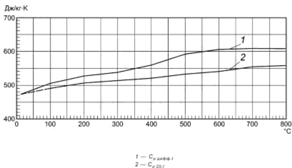
Рисунок D-3c — Теплоемкость сталей групп 8.2 и 215S15
