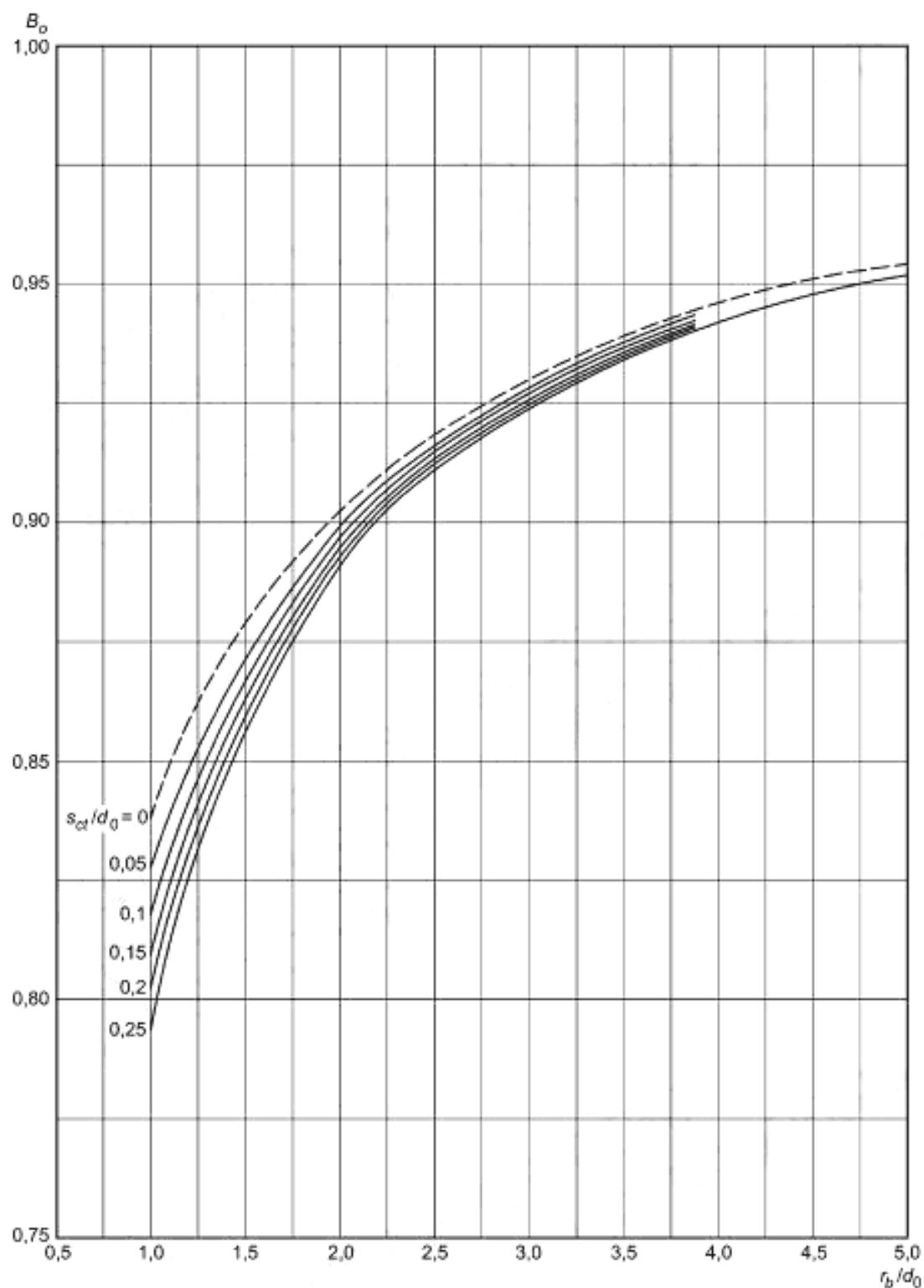
Рисунок А-5 — Расчетный коэффициент B_0 для наружной образующейгиба трубы с номинальным наружным диаметром
