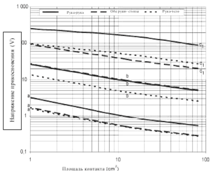
Рисунок 3 - Минимум напряжения прикосновения при переменном токе и влажных, соленых (морских) средах для тока вызывающего реакцию испуга (a), мышечную реакцию (b) и вентрикулярную фибрилляцию (c1)
