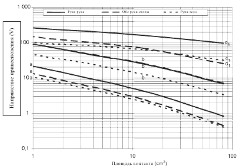
Рисунок 2 - Минимум напряжения прикосновения при переменном токе и влажных средах для тока вызывающего реакцию испуга (a), мышечную реакцию (b) и вентрикулярную фибрилляцию (c1)
