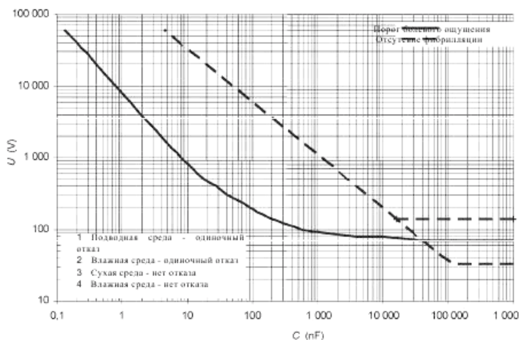
Рисунок А.1 - Параметры заряженных конденсаторов
