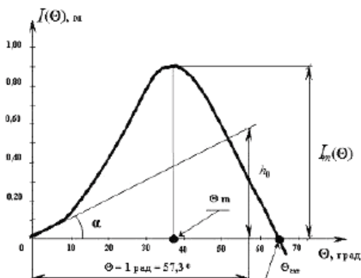
Рисунок К.3 – Диаграмма статической остоичивости
