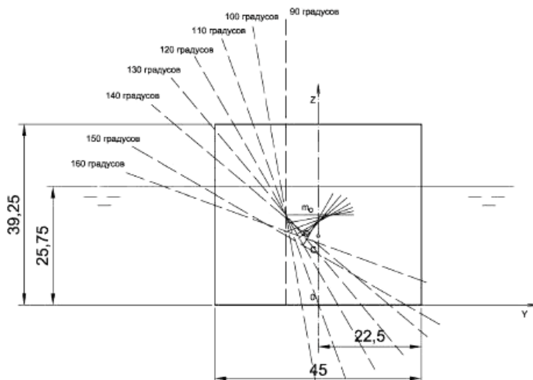
Рисунок К.10 – Положения ватерлиний и соответствующих им перпендикуляров при изменении углов крена от 0^\circ до 160^\circ
