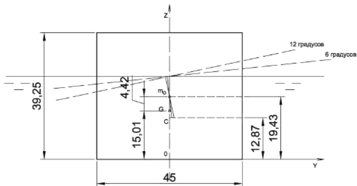
Рисунок К.6 – Общий вид расчетной схемы для положений ватерлинии при углах крена 6 и 12 градусов с заштрихованной трапецией, соответствующей углу крена объекта 12°.
