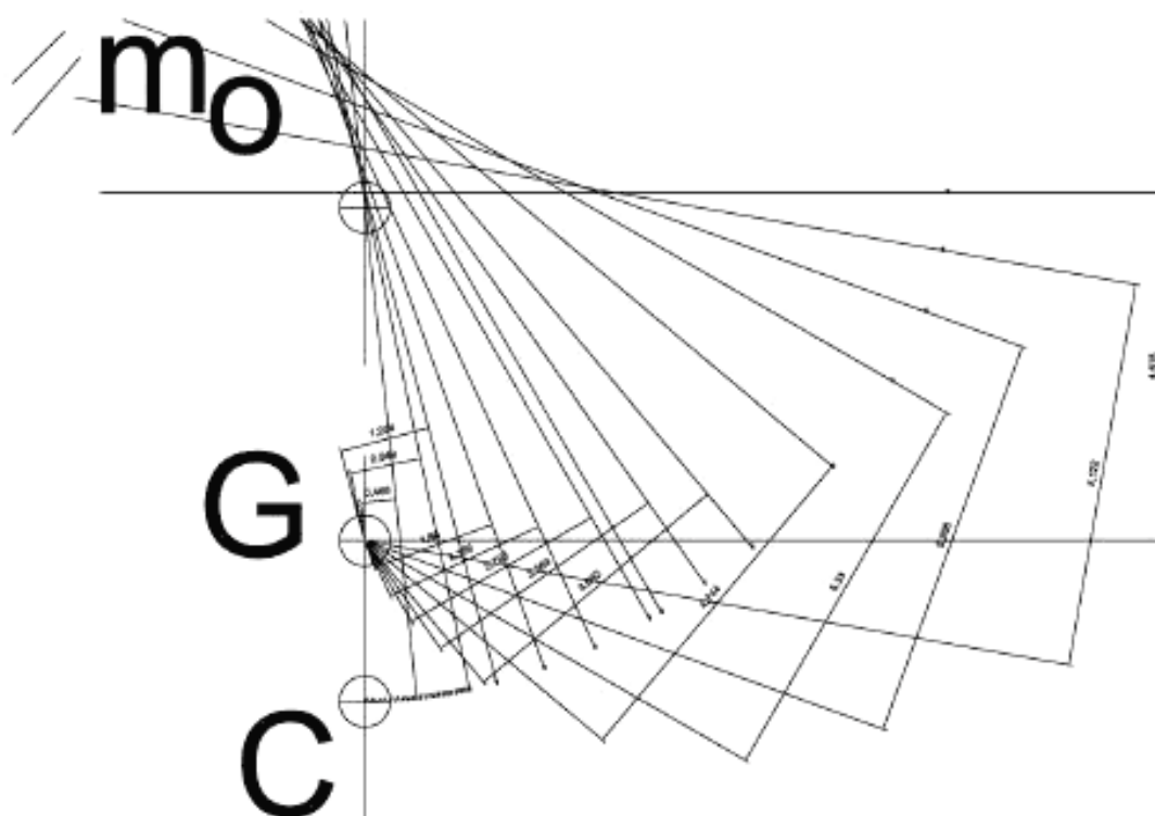
Рисунок К.9 – Измеренные плечи пар сил I(\theta) , при кренах от 0^\circ до 90^\circ
