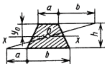
Рисунок К.5 – Определение площади и центра тяжести трапеции
