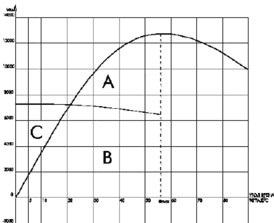
Рисунок 1 – Диаграмма статической остойчивости
