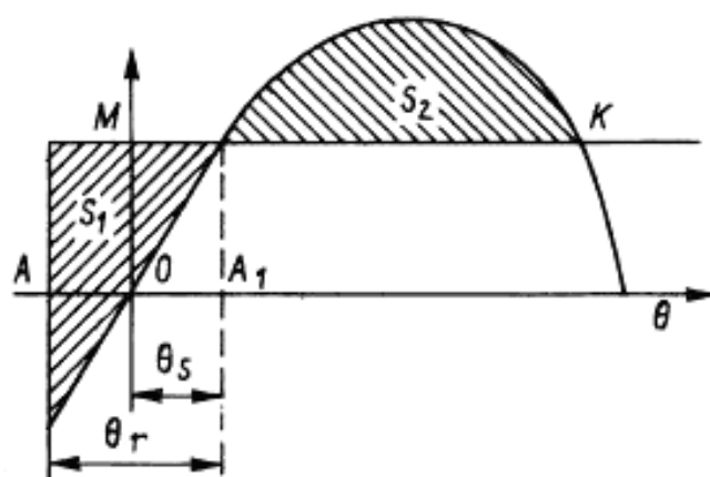
Рисунок 2 – Определение опрокидывающего момента наплавного блока по диаграмме статической остойчивости
