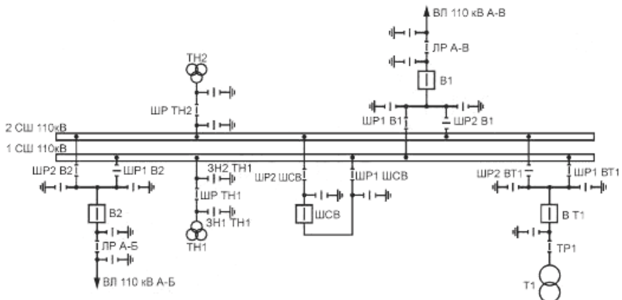
Рисунок Е.1 — Схема РУ с двумя системами шин
