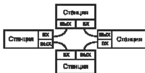
Рисунок 4 — Топология «кольцо»
