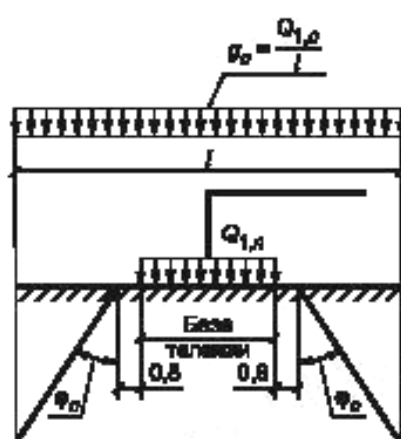
б) Схема распределения нагрузки вдоль грузового причала от ноги крана
