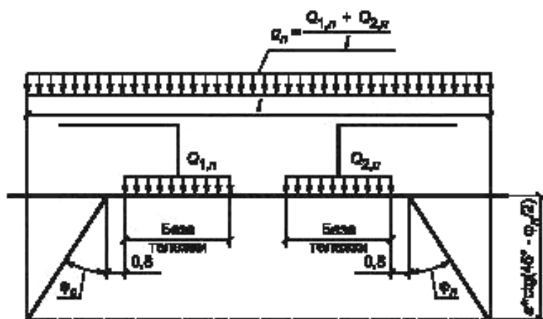
а) Схема нагрузки в направлении ширины грузового причала от ноги крана
