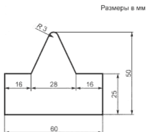
Рисунок 2 — Поперечный профиль и размеры бойка
