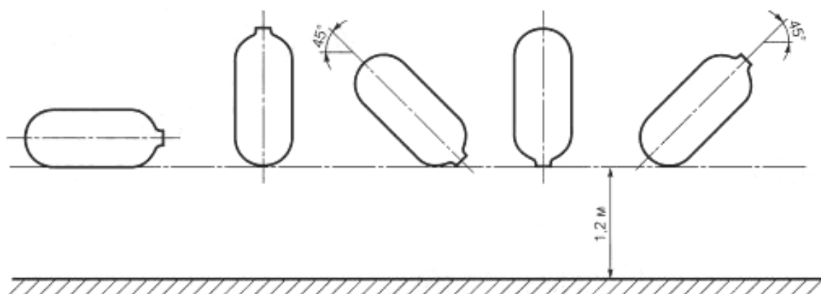
Рисунок 5 — Ориентация баллона при испытании
