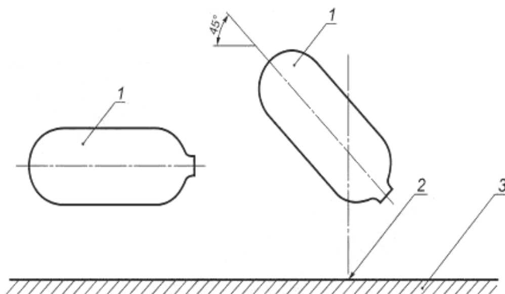
1 — испытываемый баллон; 2 — точка соударения; 3 — испытательная плита
