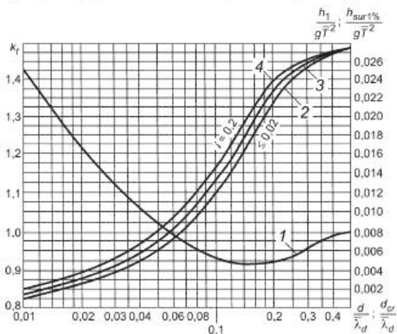
Рисунок А.5 — Графики для определения 1 — коэффициента k_r ; 2, 3 и 4 — величины d_{cr} / \bar{\lambda}_d
