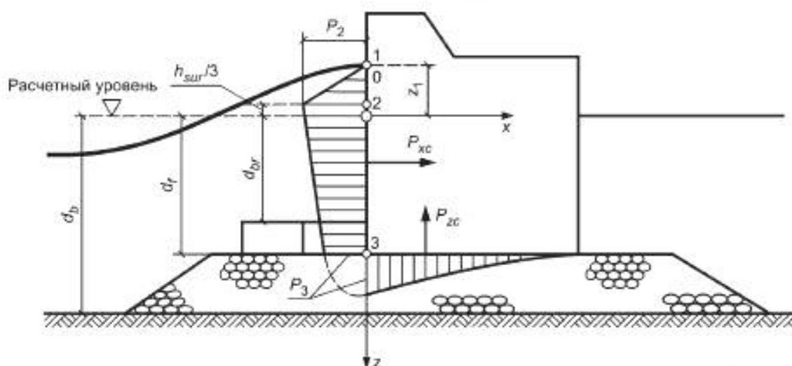
Рисунок 8 — Эпюры давления разбивающихся волн на вертикальную стену
