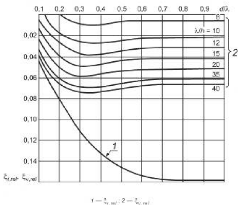
Рисунок 21 — Графики значений относительных ординат
