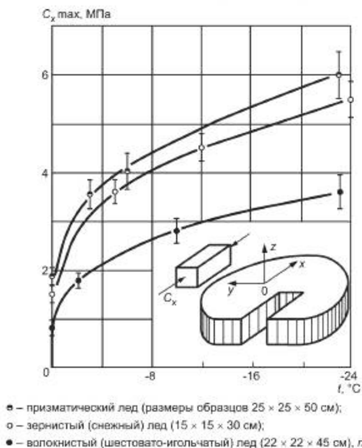
Рисунок Б.2 — Зависимость максимального предела прочности пресноводного льда при одноосном сжатии от температуры
