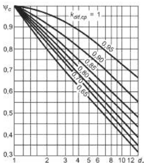
Рисунок A.8 — Графики значений коэффициента \psi_c
