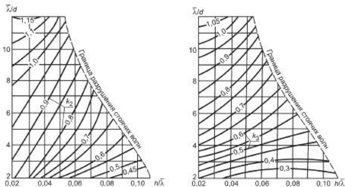
Рисунок 3 — Графики значений коэффициентов k_2 и k_3
