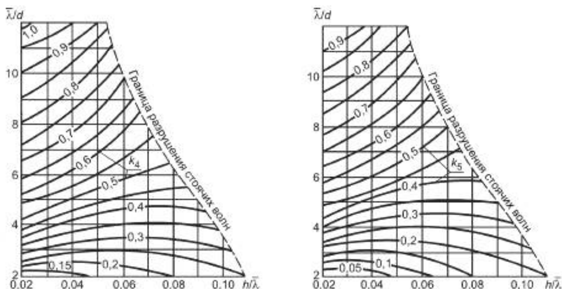
Рисунок 4 — Графики значений коэффициентов k_4 и k_5
