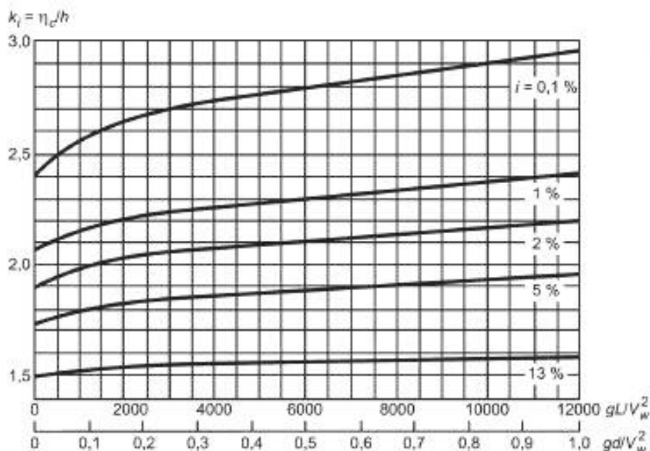
Рисунок А.2 — Графики значений коэффициента k_i
