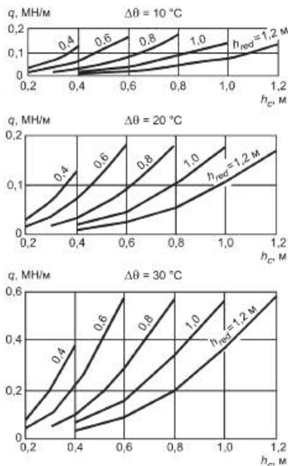
Рисунок 40 — График значений нагрузки q
