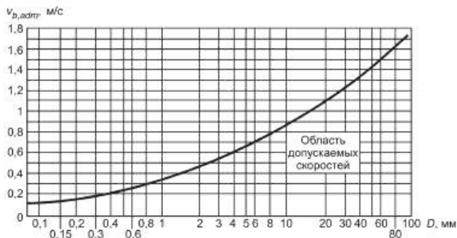
Рисунок 7 — График допустимых значений неразрывающих донных скоростей
