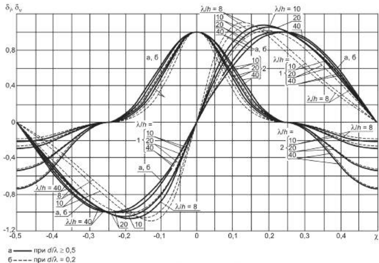
Рисунок 15 — Графики значений коэффициентов сочетания инерционного \delta_i и скоростного \delta_v компонентов силы от воздействия волн
