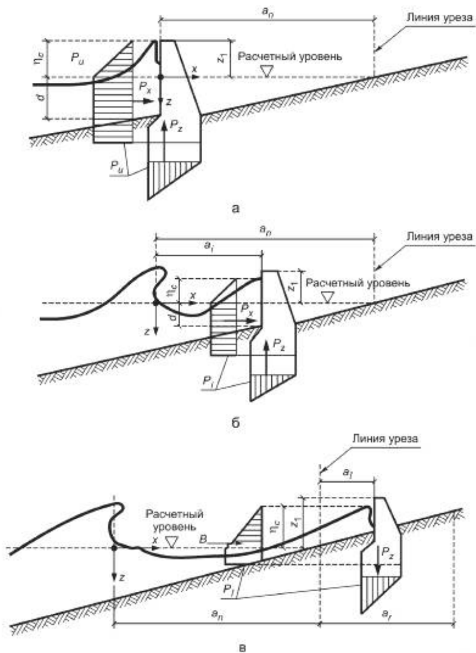
Рисунок 27 — Эпюры волнового давления на вертикальную волнозащитную стену при расположении сооружения
