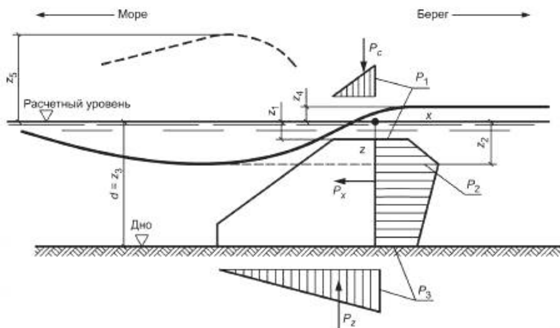
Рисунок 26 — Эпюры волнового давления на подводный волнолом
