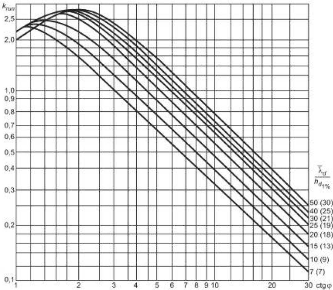
Рисунок 10 — Графики значений коэффициента k_{гип}
