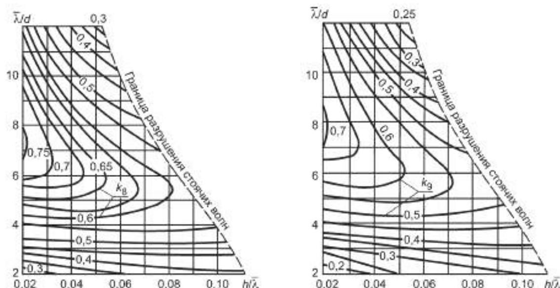
Рисунок 5 — Графики значений коэффициентов k_8 и k_9
