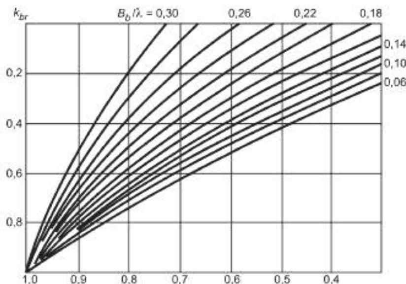
Рисунок 2 — Графики значения коэффициента k_{br}
