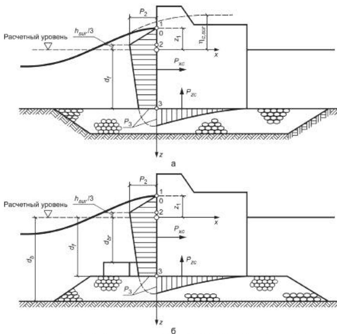
Рисунок 9 — Эпюры давления прибойных волн на вертикальную стену
