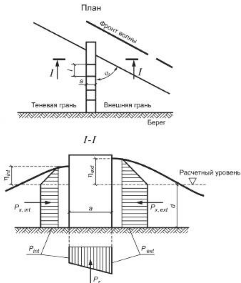
Рисунок 30 — Эпюры волнового давления на буну
