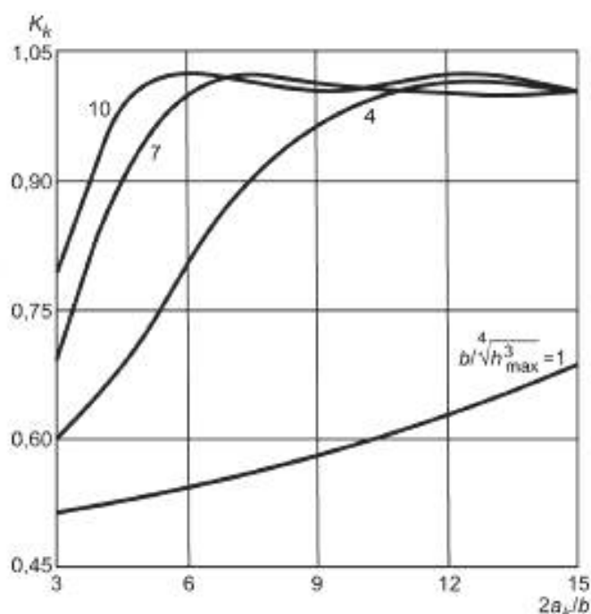
Рисунок 44 — Графики значений коэффициента K_k
