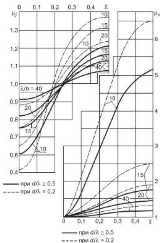
Рисунок 22 — Графики значений инерционного \mu_y и скоростного \mu_v коэффициентов фазы
