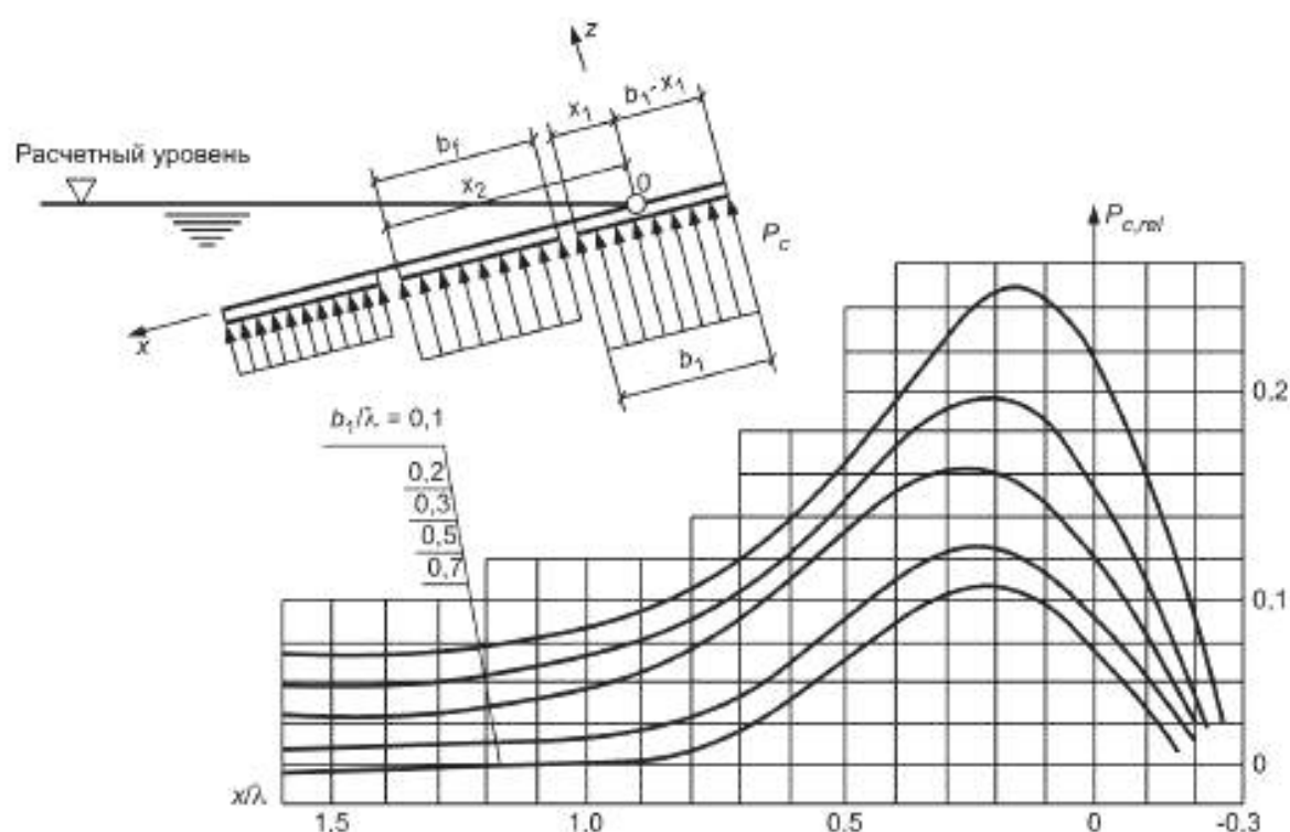
Рисунок 12 — Графики для определения относительного волнового противодействия
