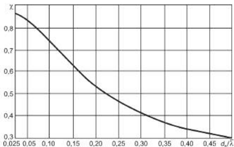
Рисунок 32 — График значений коэффициента \chi
