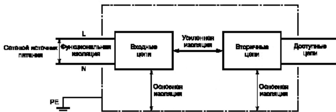
Рисунок 5a — Пример 1 — Упрощенная схема изоляционной системы, содержащей функциональную, основную и усиленную/двойную изоляцию для оборудования класса I
