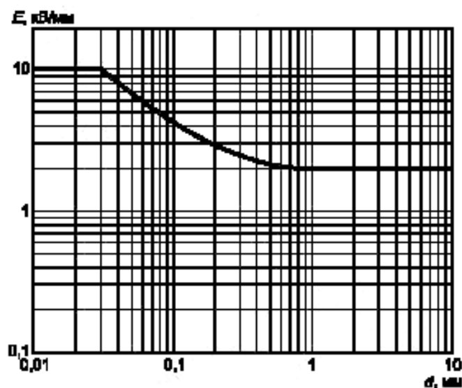
Рисунок 4 — Допустимая напряженность электрического поля для назначения твердой изоляции в соответствии с равенством (7)
