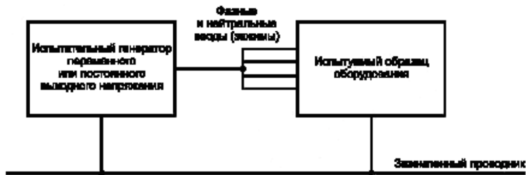
Рисунок 6 — Установка для испытания напряжением переменного (или постоянного) тока
