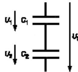
U_0 — напряжение, приложенное к изоляции; U_1 — напряжение, приложенное к изоляционному промежутку; U_2 — напряжение, приложенное к твердой изоляции; C_1 — емкость изоляционного промежутка; C_2 — емкость твердой изоляции
