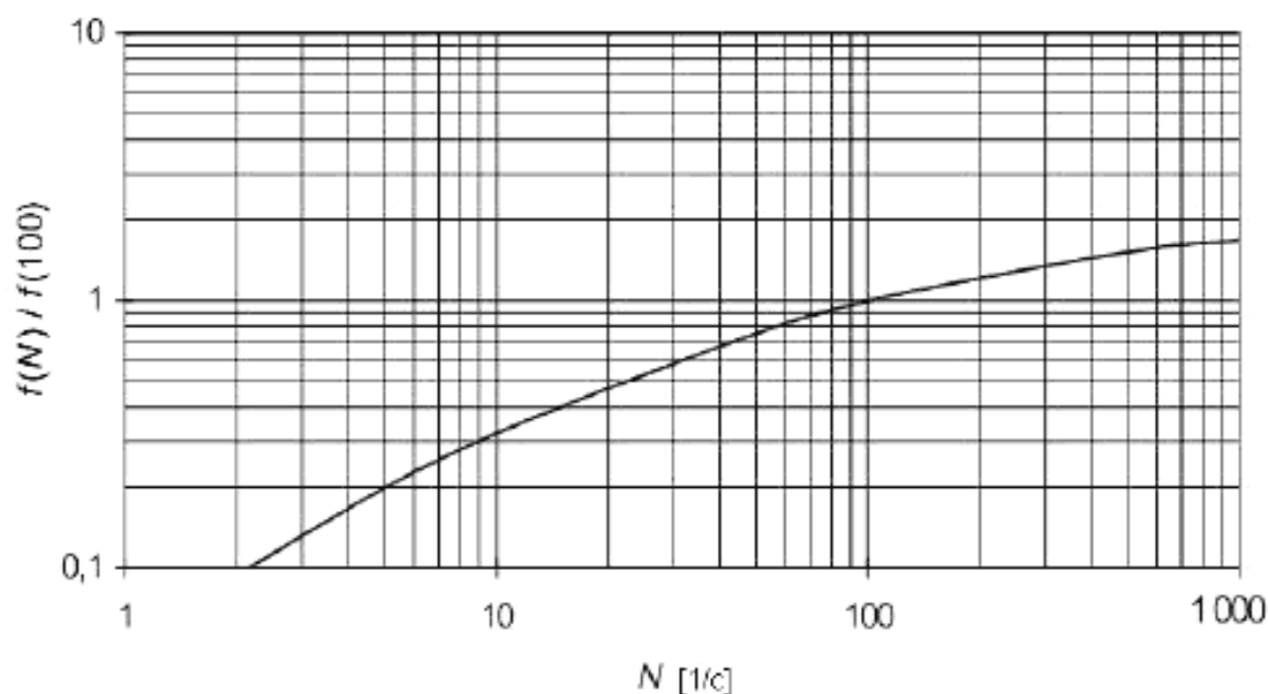
Рисунок Г.1 – Изменение показания f(N) измерителя радиопомех СИСПР в зависимости от частоты повторения импульсов N для постоянных импульсов.
