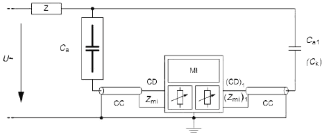
в – Балансная схема
