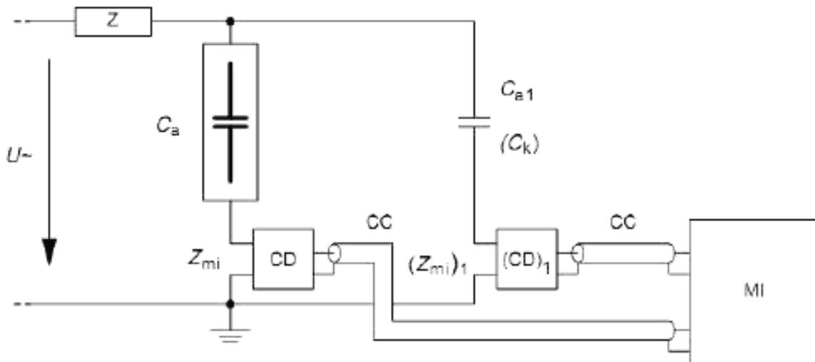
г – Схема дискриминатора полярности
