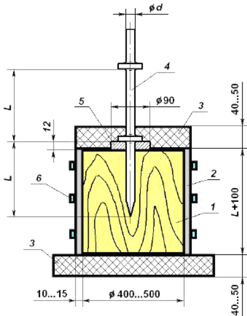
1 – цилиндрическая деревянная колода; 2 – войлочная изоляция; 3 – резиновые пластины; 4 – испытательная двухбуртная пила; 5 – стальная шайба, 6 – обечайка
