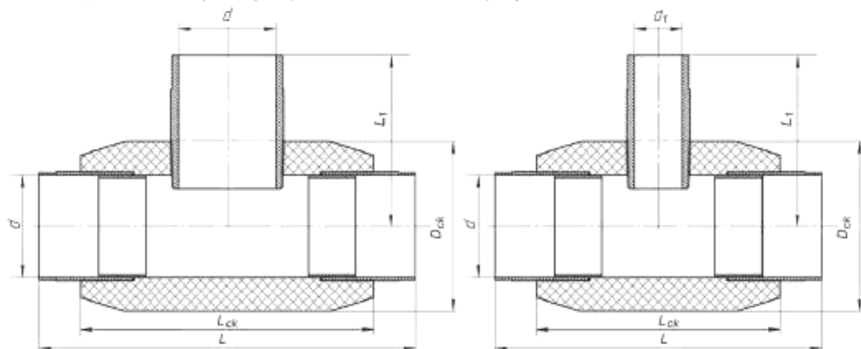
а) Тройник равнопроходной
