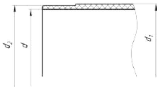
d – внутренний диаметр трубы; d_1 – наружный диаметр трубы; d_2 – диаметр ниппеля Рисунок 2 – Ниппель под соединение «К» без утолщения
