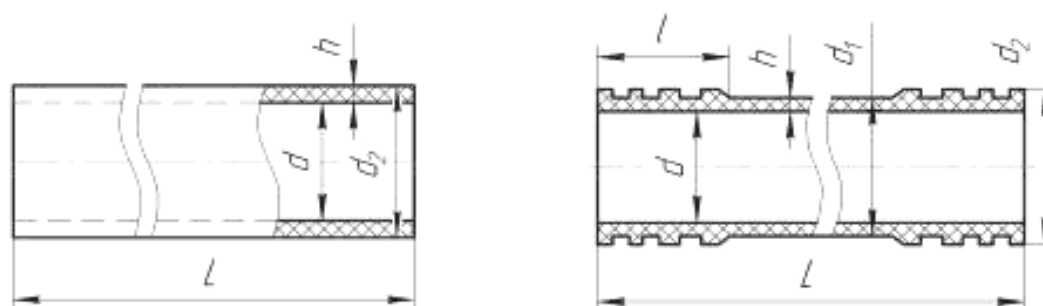
а) труба с присоединительными частями без утолщений
