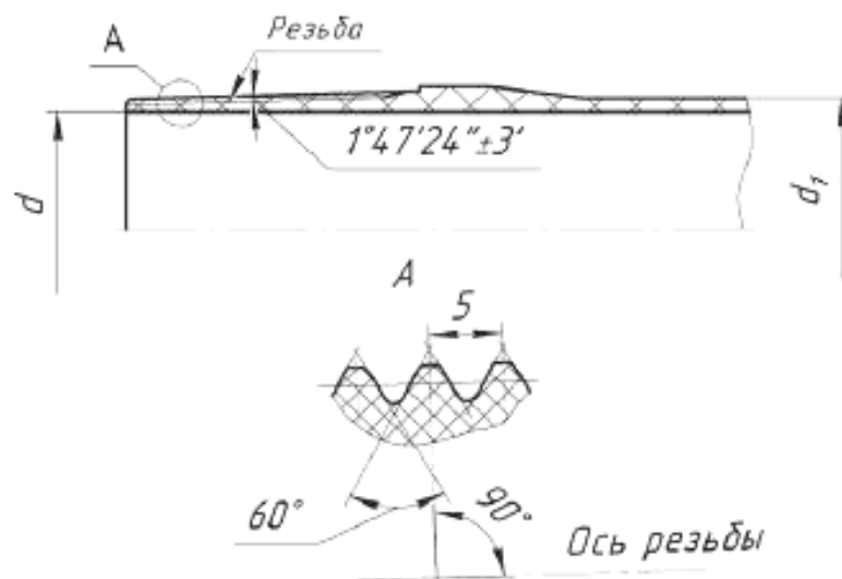
Рисунок 5 – Резьбовая концевая часть под соединение «РКН»
