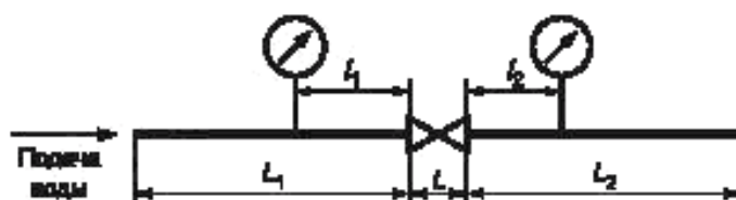
Рисунок 1 — Принципиальная схема участка расходного испытательного стенда
