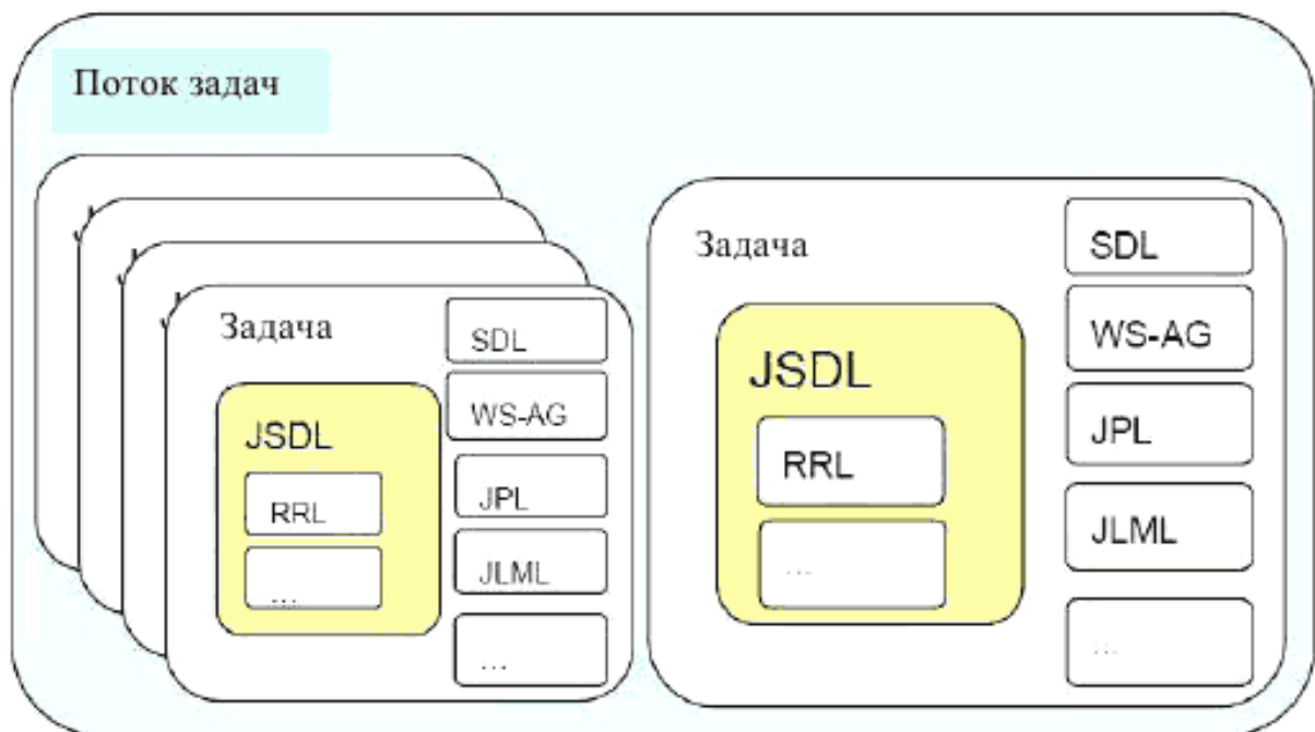
Рисунок 2 – Взаимодействие между JSDL и другими спецификациями
