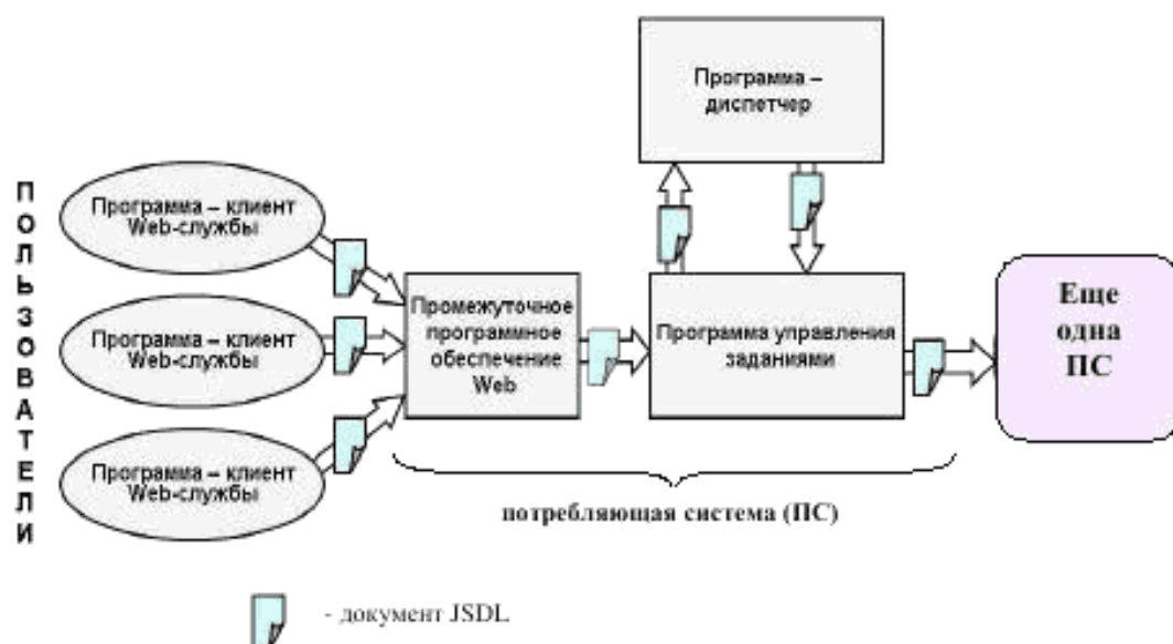
Рисунок 1 - Пользователи JSDL в Грид-среде
