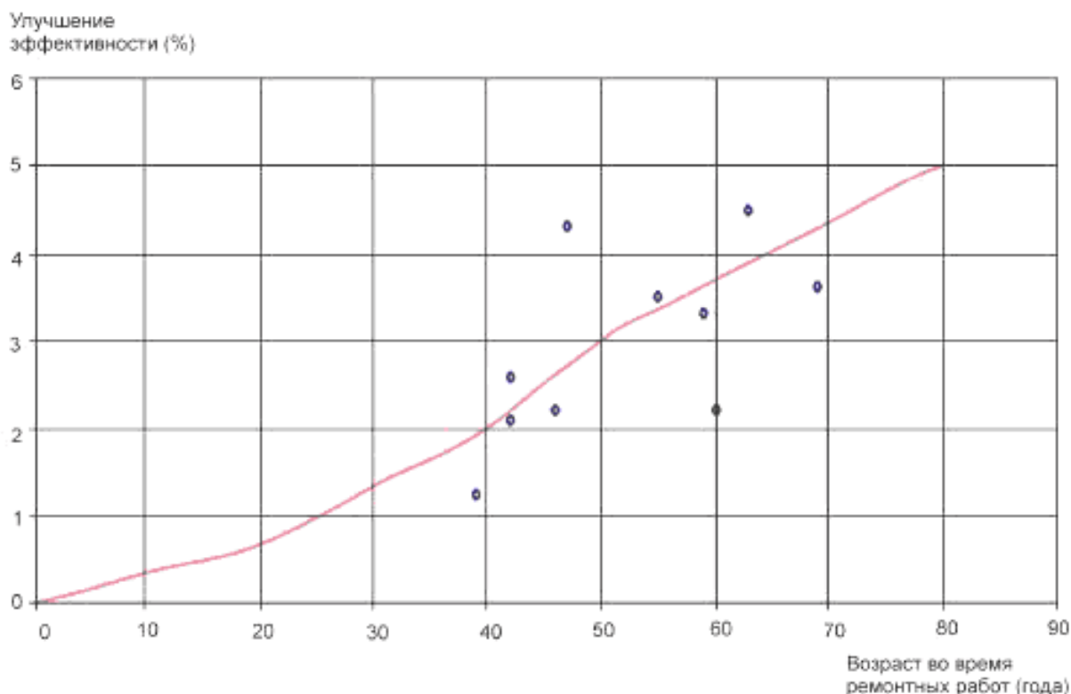
Рисунок 7b — Потенциальные усовершенствования для ремонта турбины Каплана
