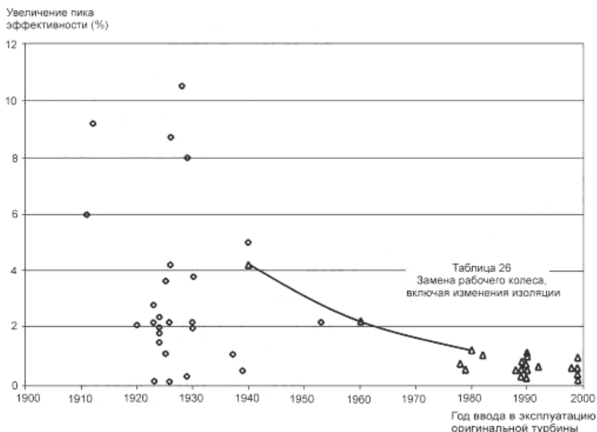
Рисунок 7а — Потенциальные усовершенствования для ремонта радиально-осевой турбины
