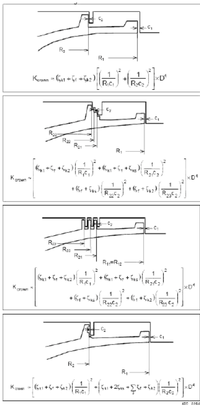
Рисунок Е.1 – Примеры типичной конструкции уплотнения рабочего колеса (сторона ступицы)
