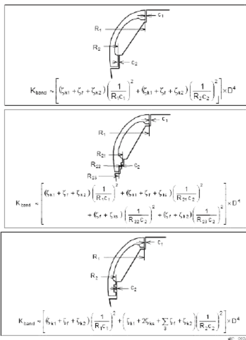
Рисунок Е.2 – Примеры типичной конструкции уплотнения рабочего колеса (сторона обода)
