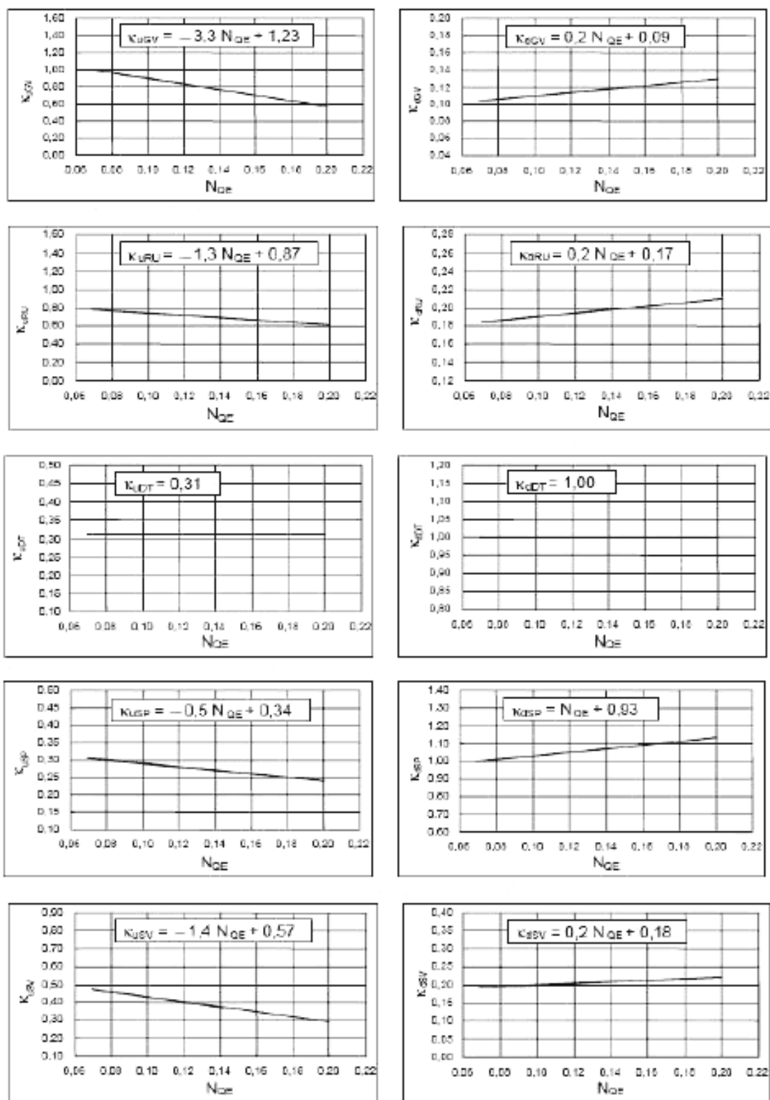
Рисунок В.8 – \kappa_{vco} и \kappa_{dco} для каждого компонента турбонасоса при работе в режиме турбины
