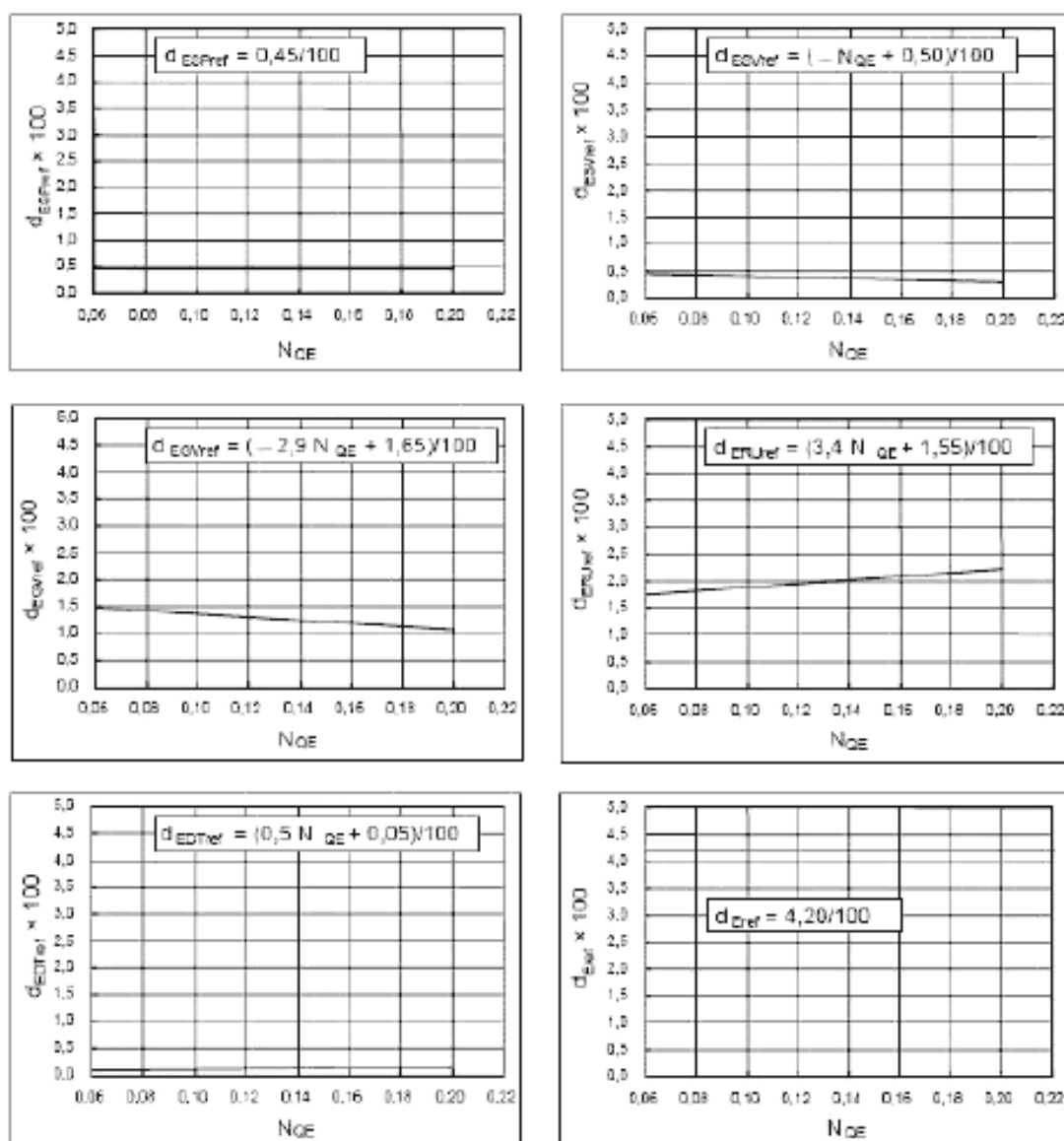
Рисунок В.12 – d_{ECOref} и d_{Eref} для турбонасоса при работе в режиме насоса
