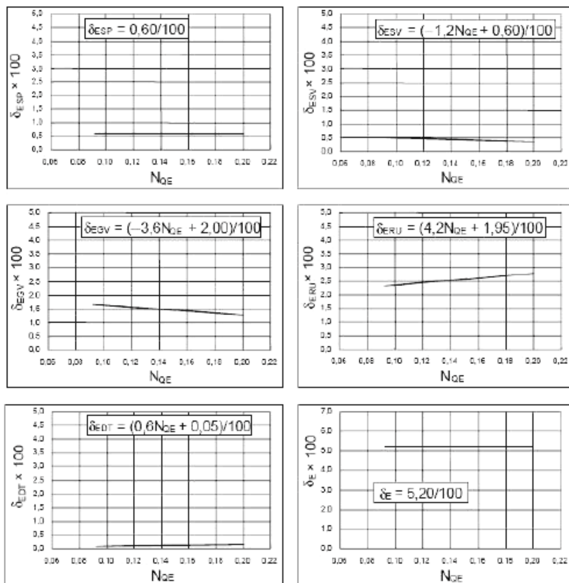
Рисунок В.6 – Относительные масштабируемые потери гидравлической энергии в каждом компоненте турбонасоса при работе в режиме насоса
