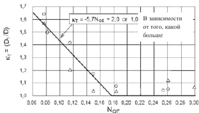
а) Фактор размеров диска \kappa_T для турбины Френсиса
