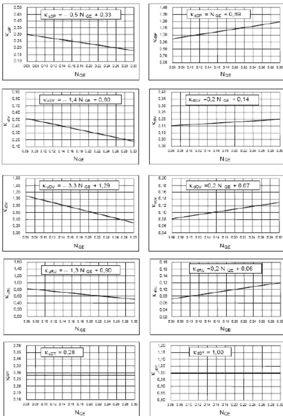
Рисунок В.7 – \kappa_{aCO} и \kappa_{dCO} для каждого компонента турбины Френсиса
