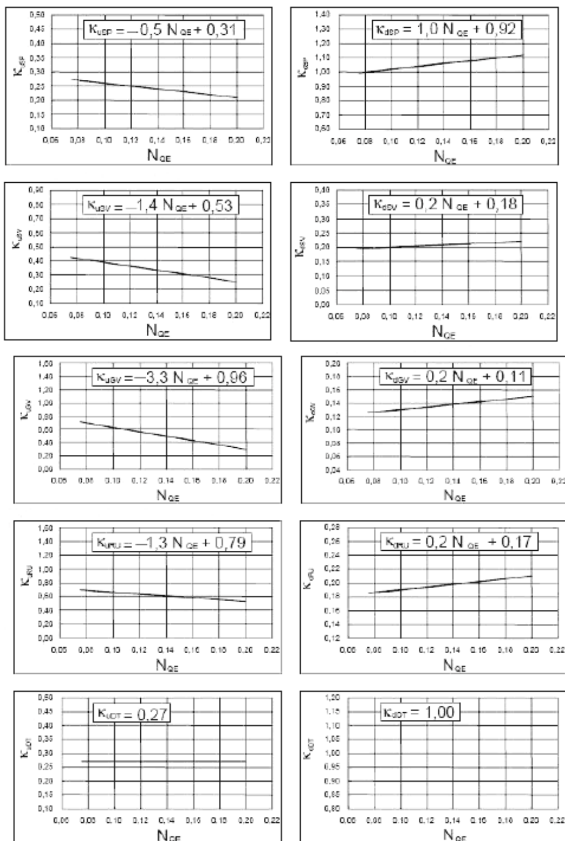
Рисунок В.9 – \kappa_{всп} и \kappa_{дсп} для каждого компонента турбонасоса при работе в режиме насоса
