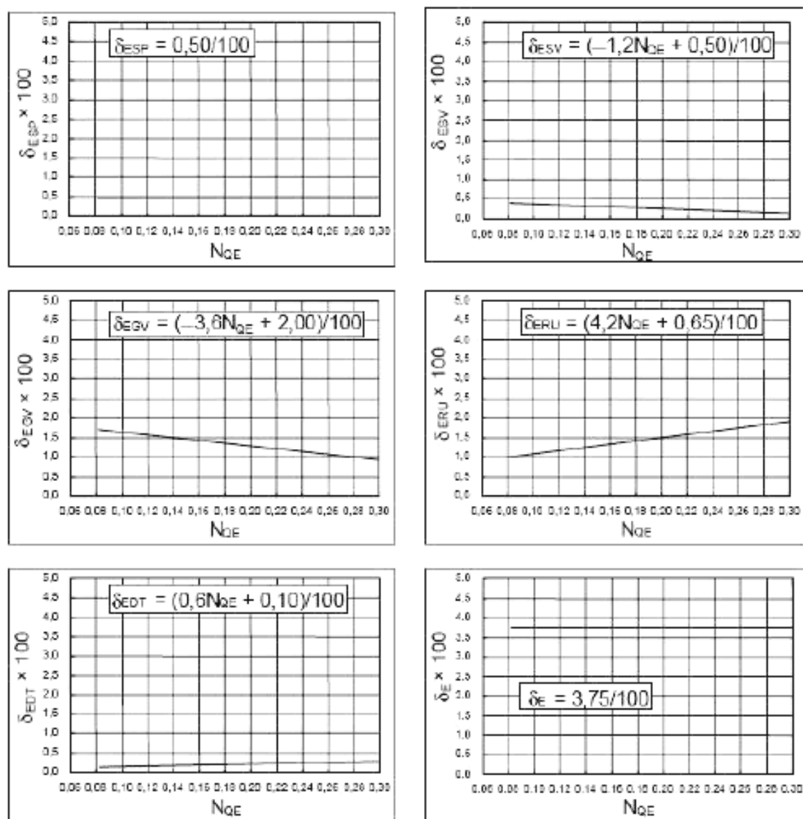
Рисунок В.4 – Относительные масштабируемые потери гидравлической энергии в каждом компоненте турбины Френсиса
