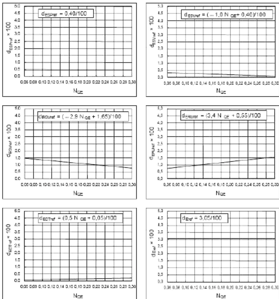
Рисунок В.10 – d_{ECOref} и d_{Eref} для турбины Френсиса
