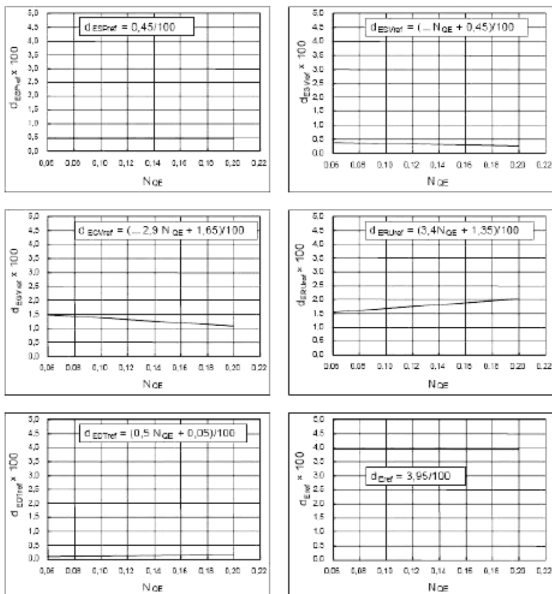
Рисунок В.11 – d_{ECOref} и d_{Eref} для турбонасоса при работе в режиме турбины
