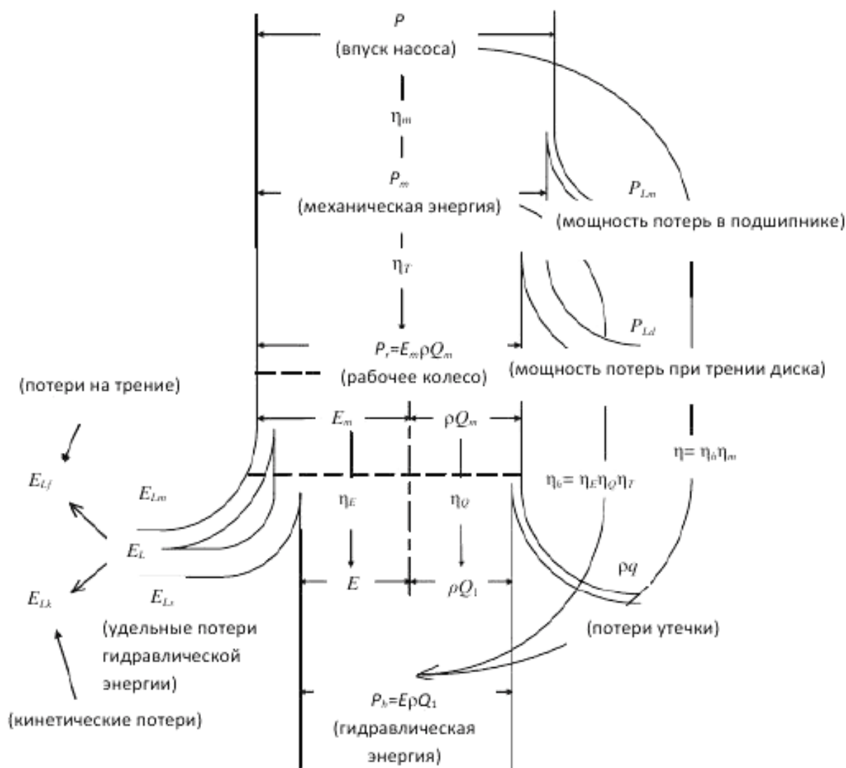
Рисунок А.2 – Диаграмма движения потока насоса
