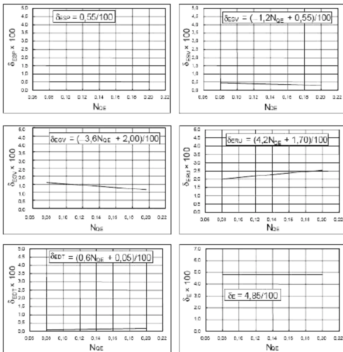
Рисунок В.5 – Относительные масштабируемые потери гидравлической энергии в каждом элементе турбонасоса при работе в режиме турбины
