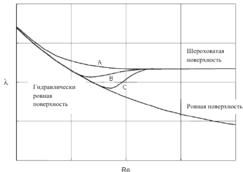
Рисунок В.2 – Различные характеристики \lambda в переходной зоне
