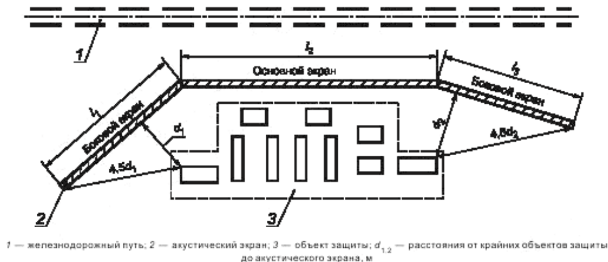
Рисунок 3 — Схема определения длины боковых акустических экранов
