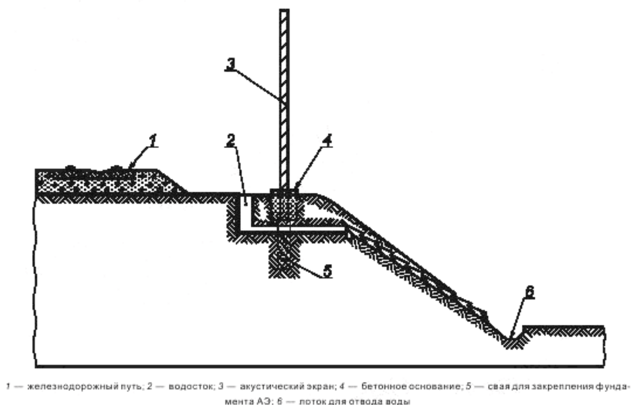
Рисунок 4 — Схема водоотводного сооружения
