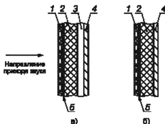
Рисунок 5 — Схема многослойной панели со звукопоглощением с воздушным промежутком (а) и без него (б)
