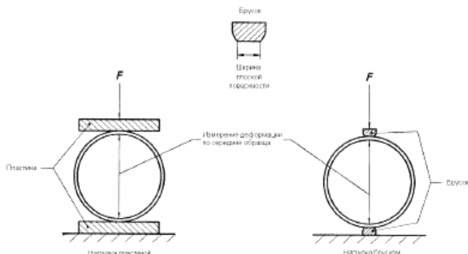
Рисунок 2 — Схема установки испытываемого образца в опорных площадках
