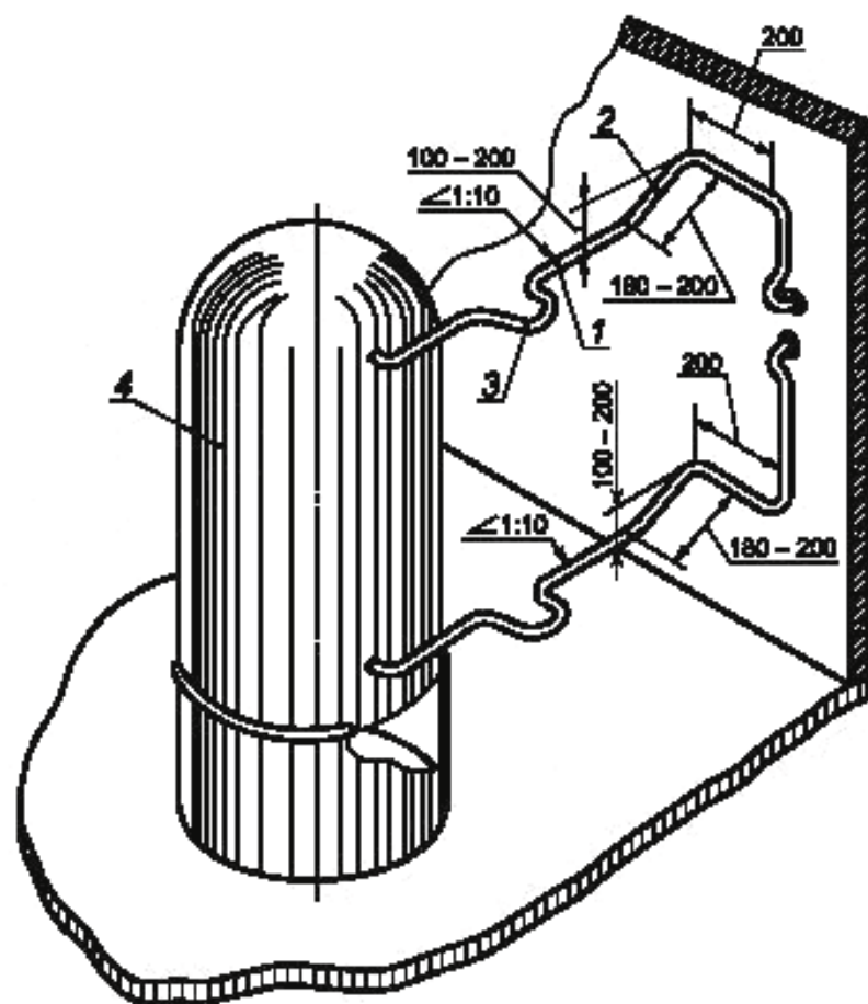
1 — трубопровод; 2 — участок подъема трубы; 3 — компенсационная петля; 4 — аппарат
