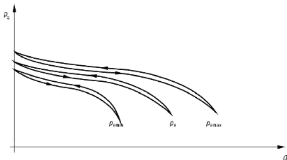
Рисунок 2 — Кривая ( p_{ас} — постоянная, p_в — постоянная)
