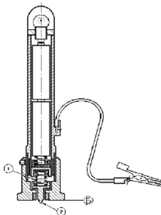
1 — Пружина с усилием 10 Н; 2 — Наконечник, которым проводят испытание цаппаньем (стальная сфера диаметром 1 мм)
