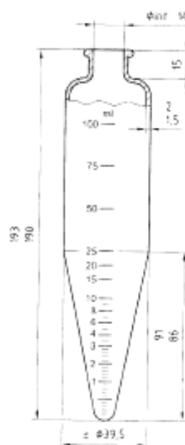
Рисунок Б.2 – Коническая центрифужная пробирка
