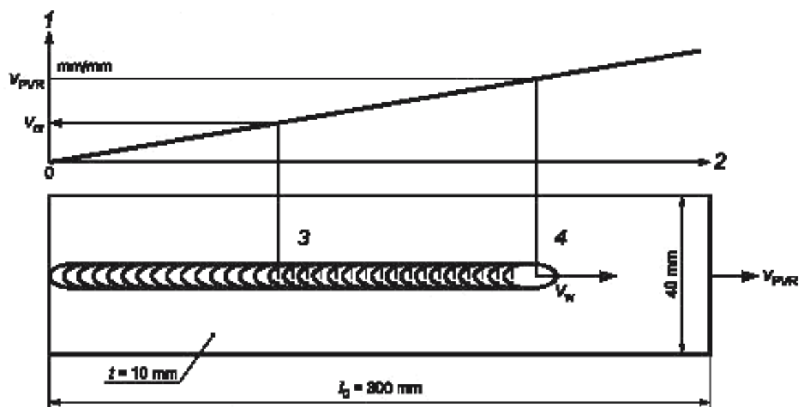
Рисунок 6 — Процедура испытания на сопротивляемость образованию горячих трещин программируемым деформированием (PVR-испытание)
