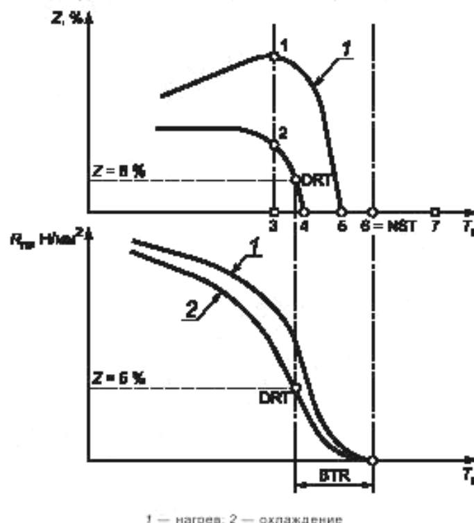
Рисунок 2 — Графики, построенные по результатам испытания
