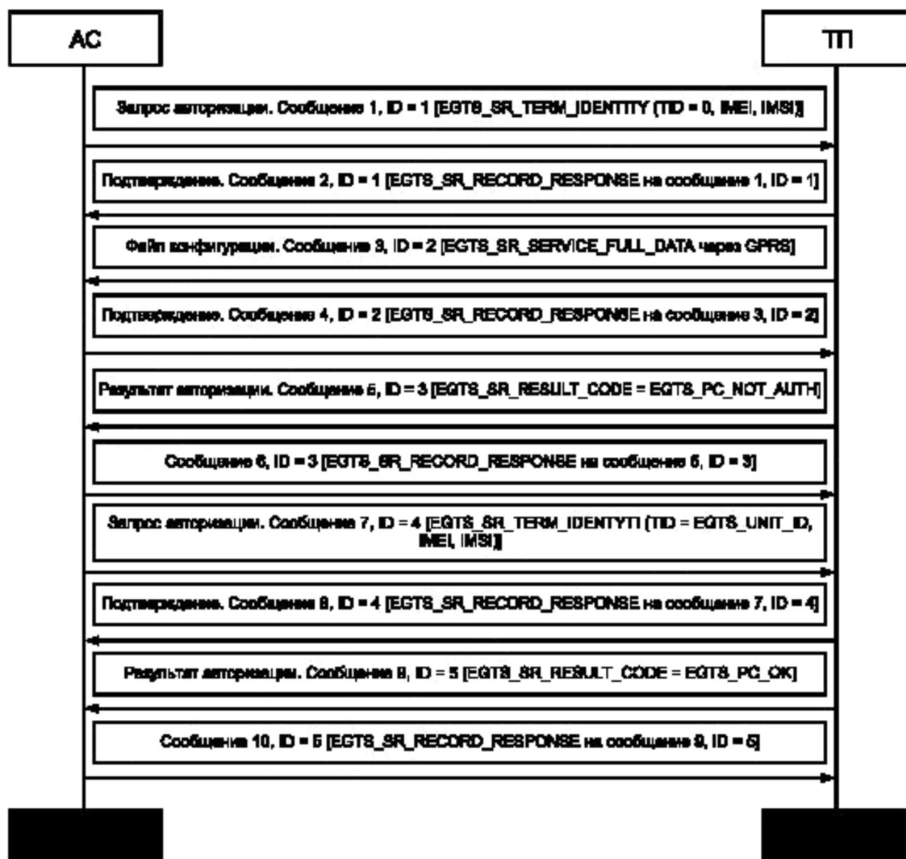
Рисунок 5 — Алгоритм конфигурации AC с использованием GPRS
