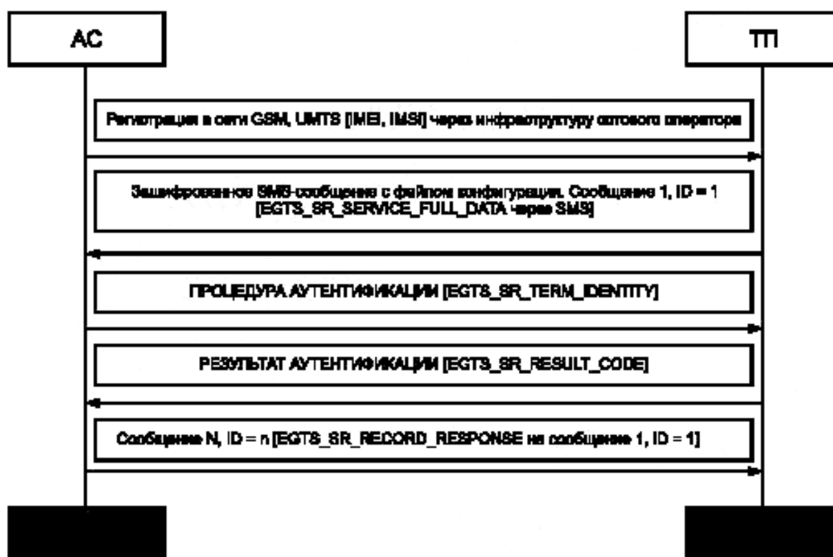
Рисунок 4 — Алгоритм конфигурации АС с использованием SM
