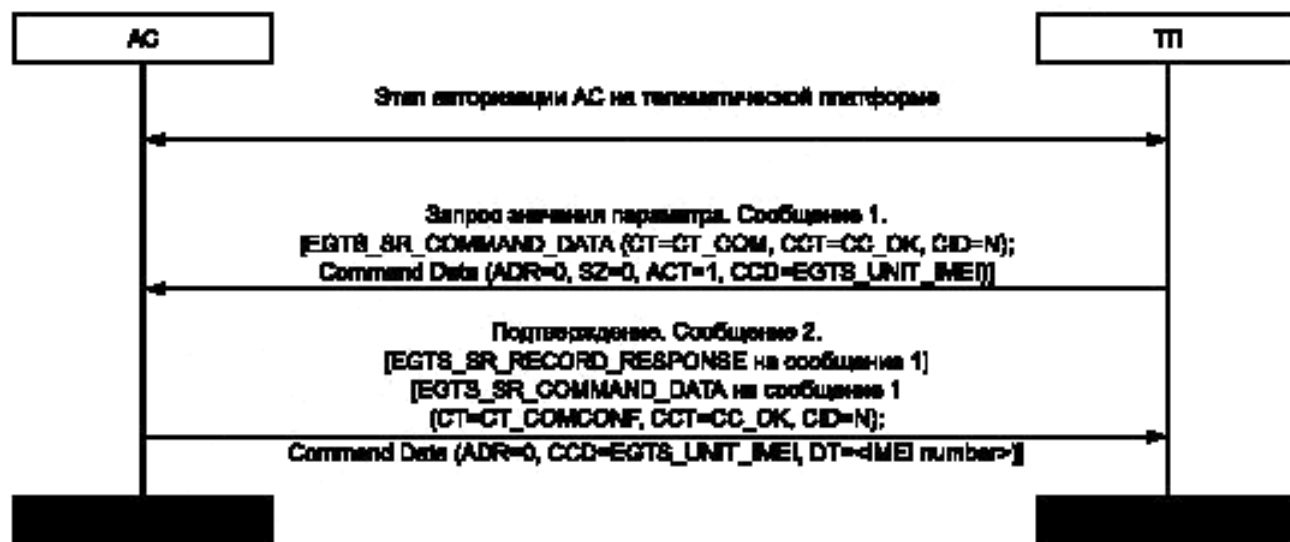
Рисунок 7б — Запрос значения параметра.
