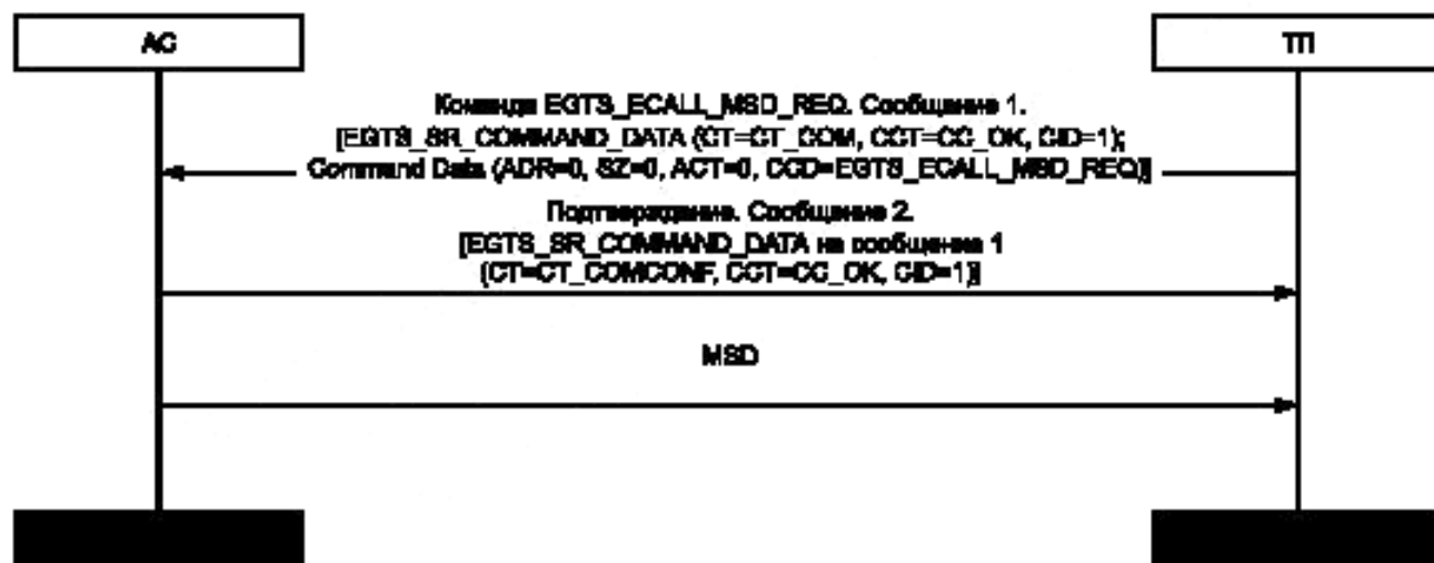
Рисунок 7а — Отправка команды EGT8_ECALL_MSD_REQ по SMS
