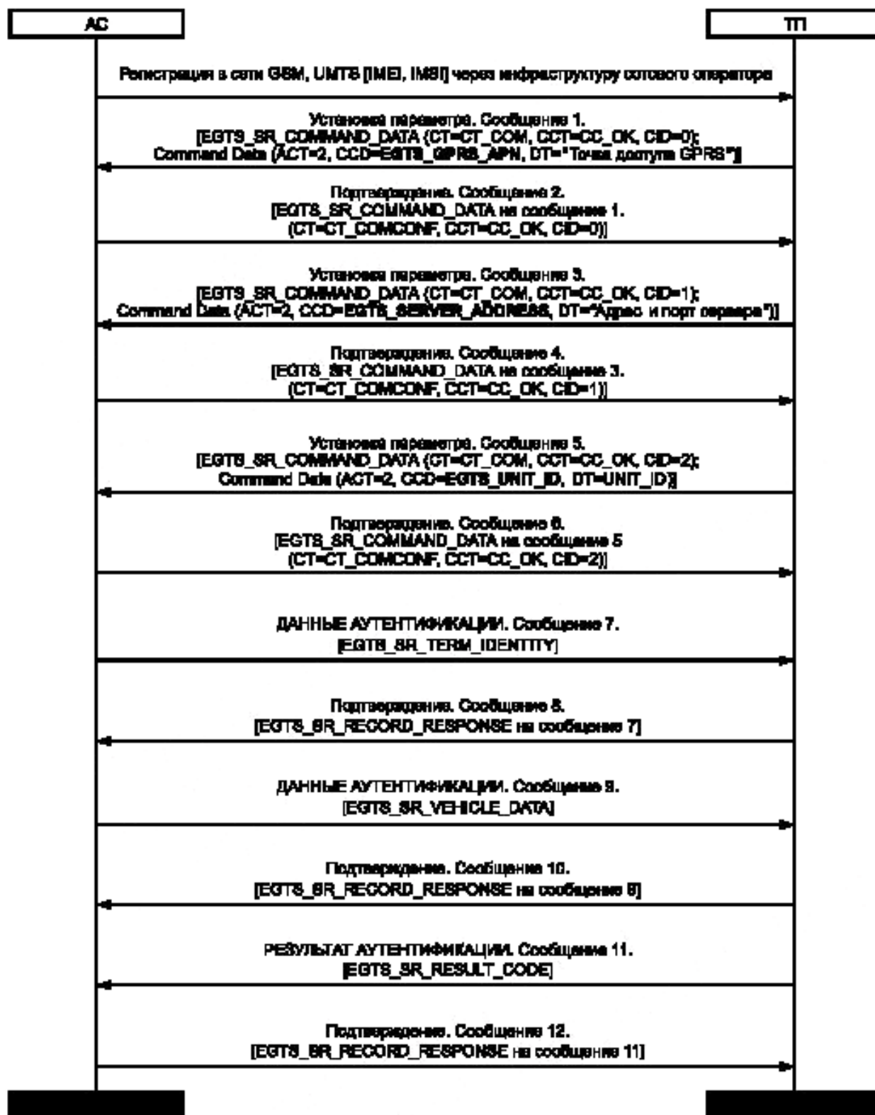
Рисунок 4 — Алгоритм конфигурации AC с использованием SMS
