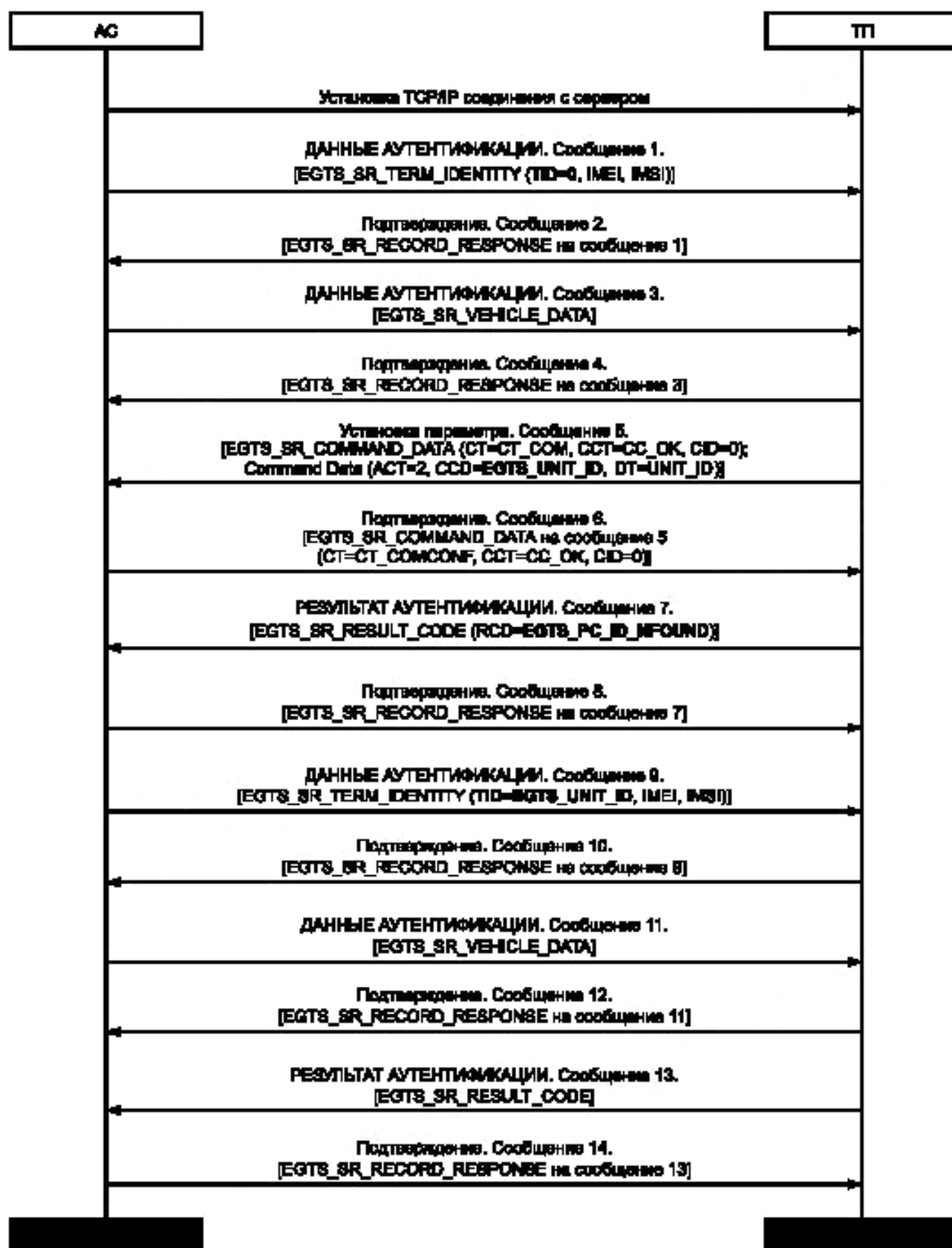
Рисунок 5 — Алгоритм конфигурации AC с использованием GPRS».
