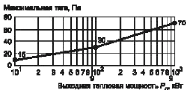
Рисунок 3 — Требования к тяге для котлов, работающих на естественной тяге при отрицательном давлении в топке
