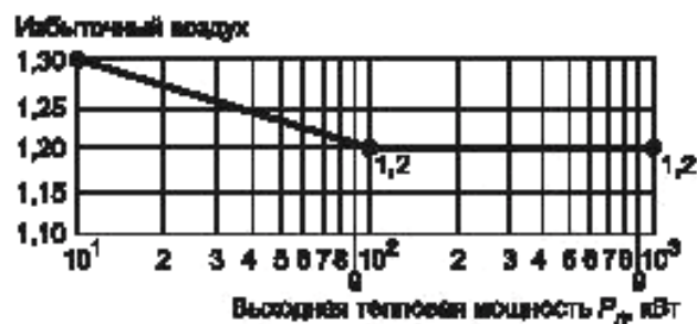
Рисунок 2 — Требования к коэффициенту избытка воздуха
