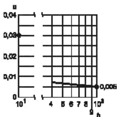
Рисунок 5 — Потери на холостом ходу
