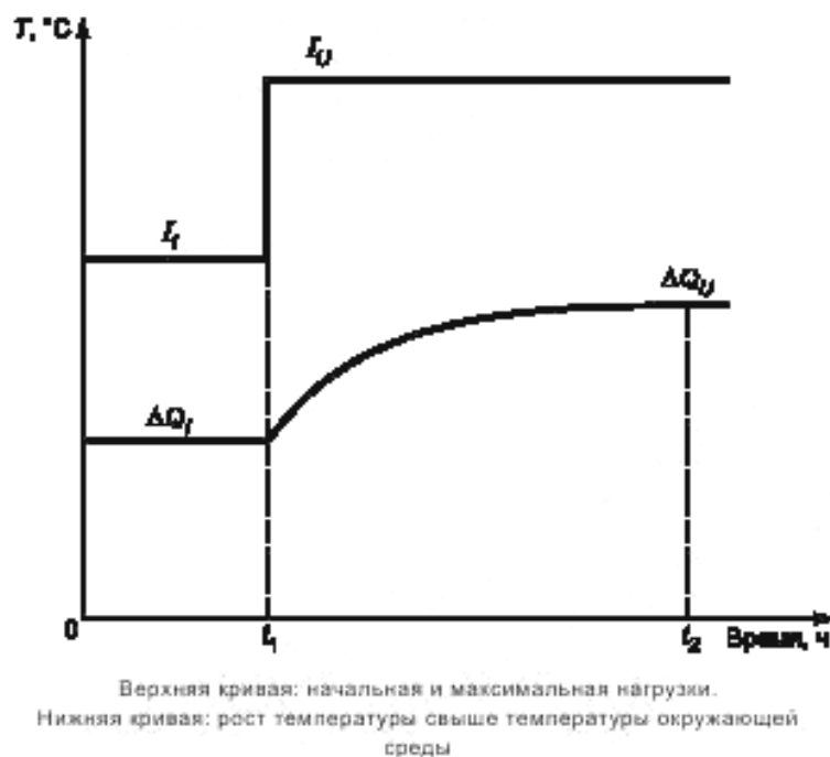
Рисунок Б.1 — Ступенчатое изменение кривой нагрузки
