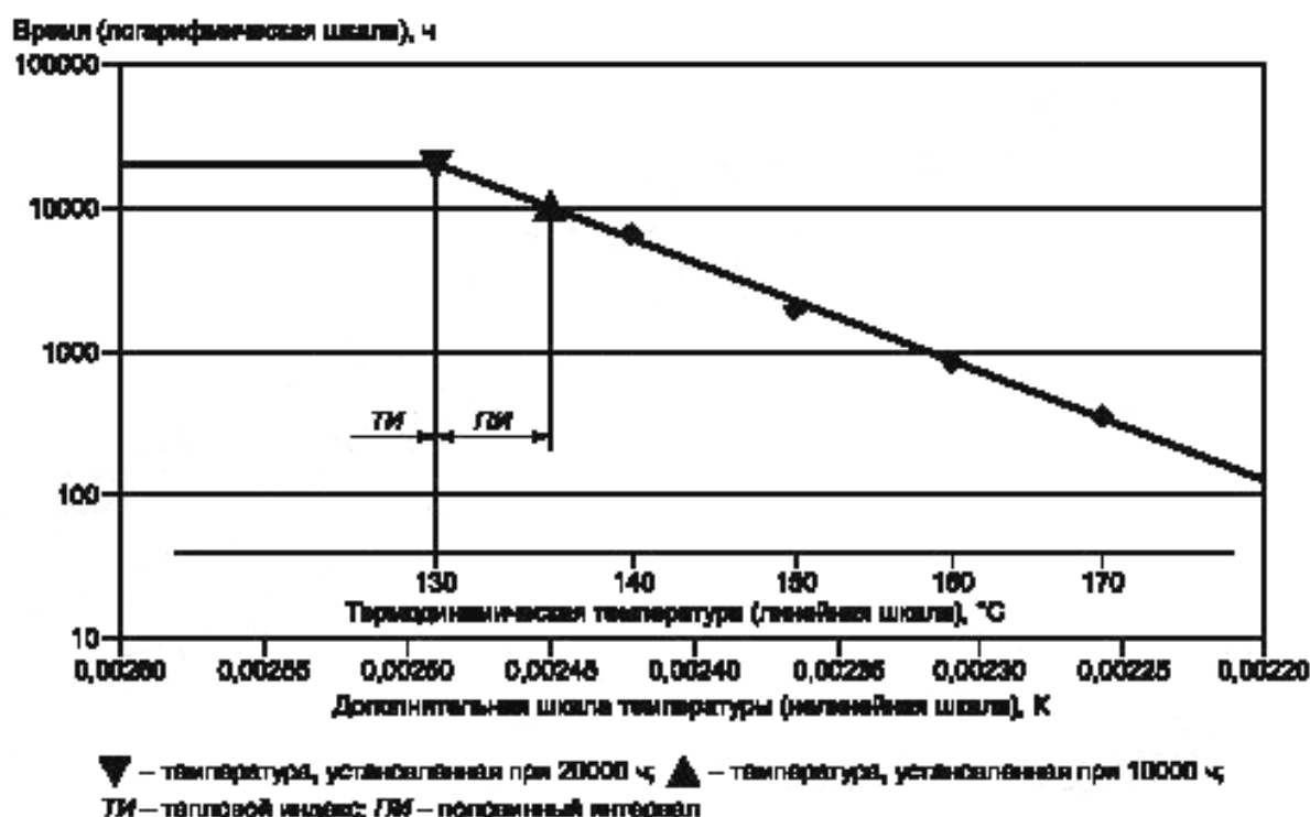
Рисунок А.2 — График теплостойкости
