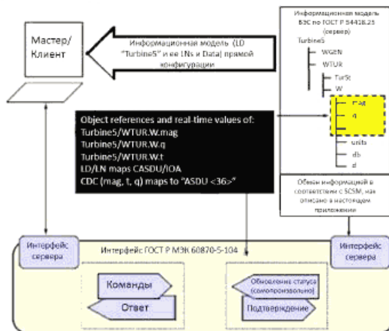
Рисунок Г.1 – Архитектура отображения (концептуальная)
