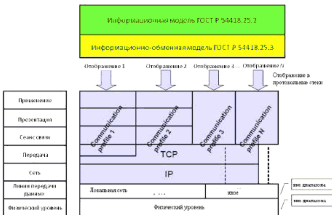
Рисунок 2 – Коммуникационные профили
