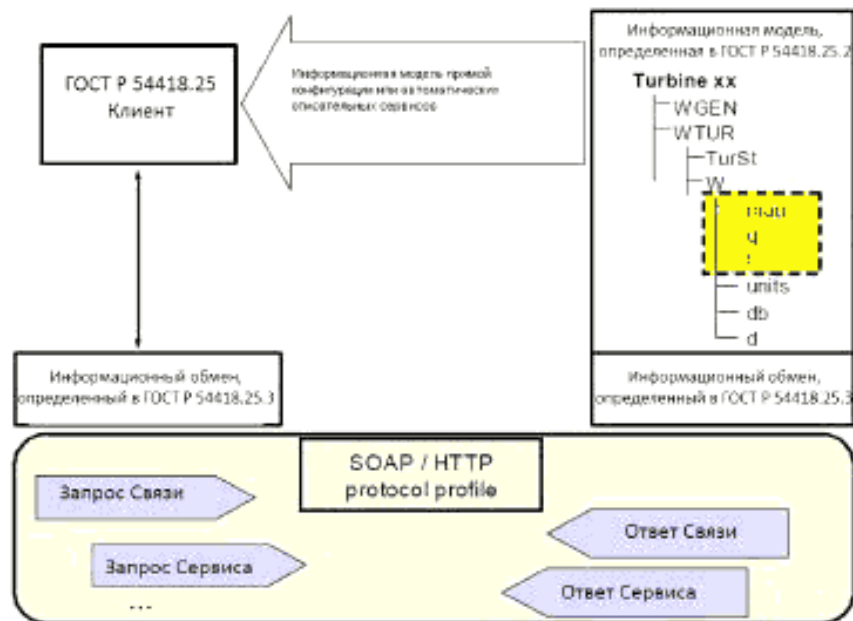
Рисунок А.1 – Структура отображения (концепция)
