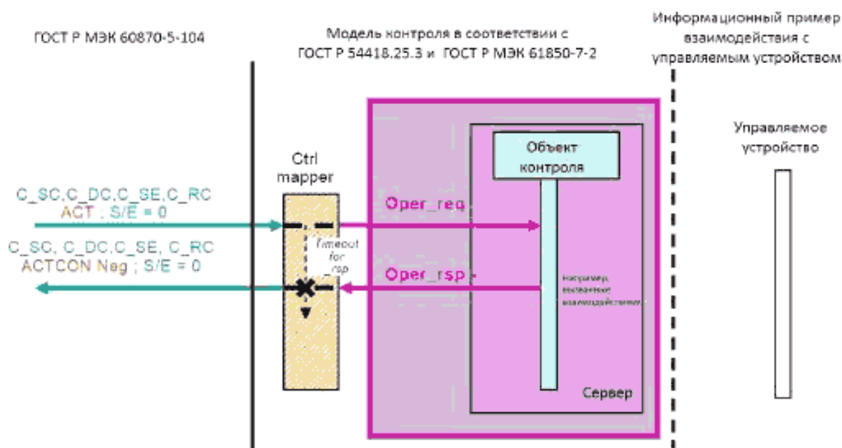
Рисунок Г.4 – Прямое Управление с общей Нормальной Безопасностью – отрицательный случай б)
