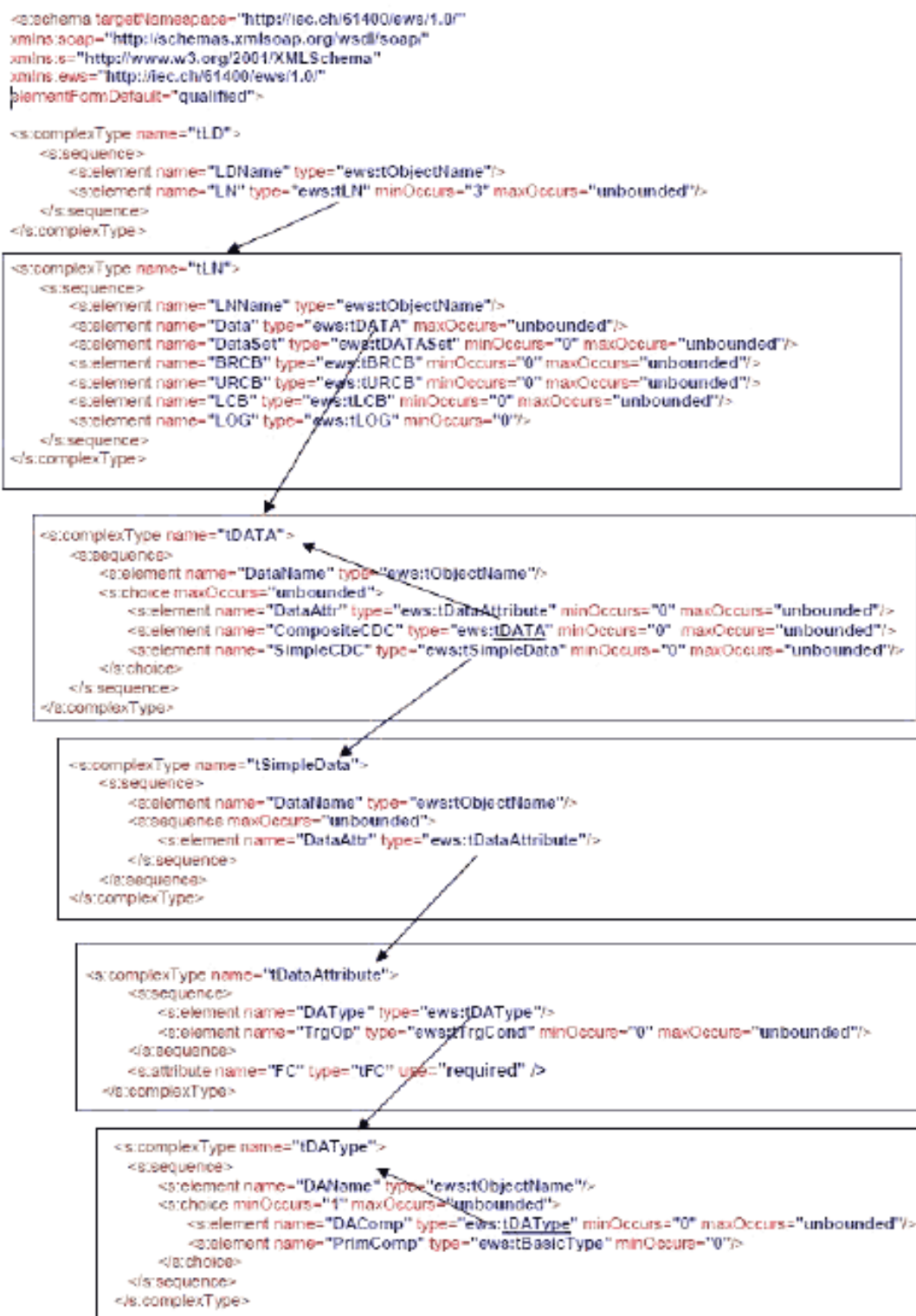
Рисунок А.2.1 – XML схема для информационной модели ВЭС
