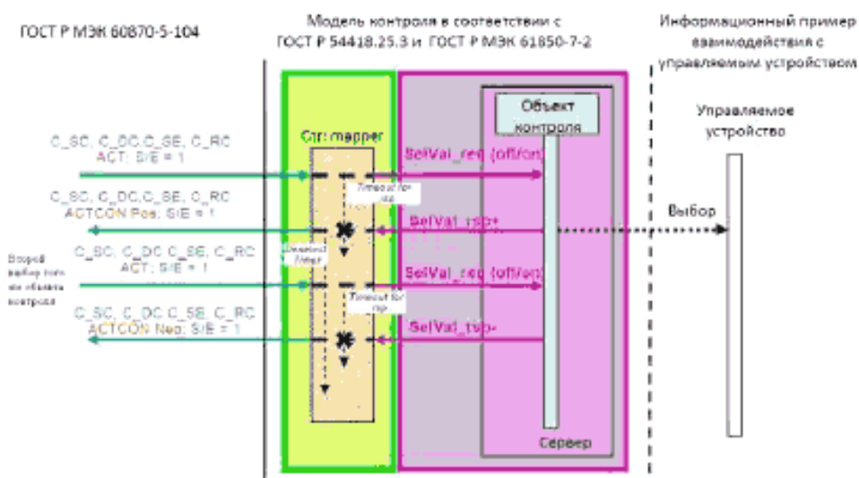
Рисунок Г.13 – SBO-Управление – отрицательный случай в)
