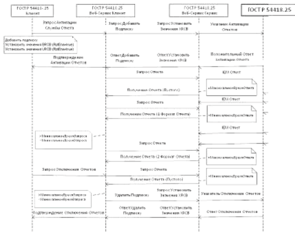
Рисунок А.5 – Механизм сервисов реализации отчетов (концепция)
