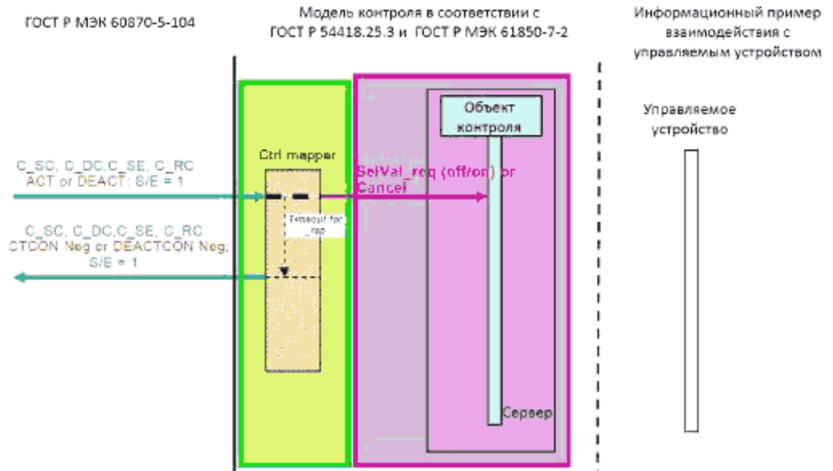
Рисунок Г.11 – SBO-Управление – отрицательный случай а)
