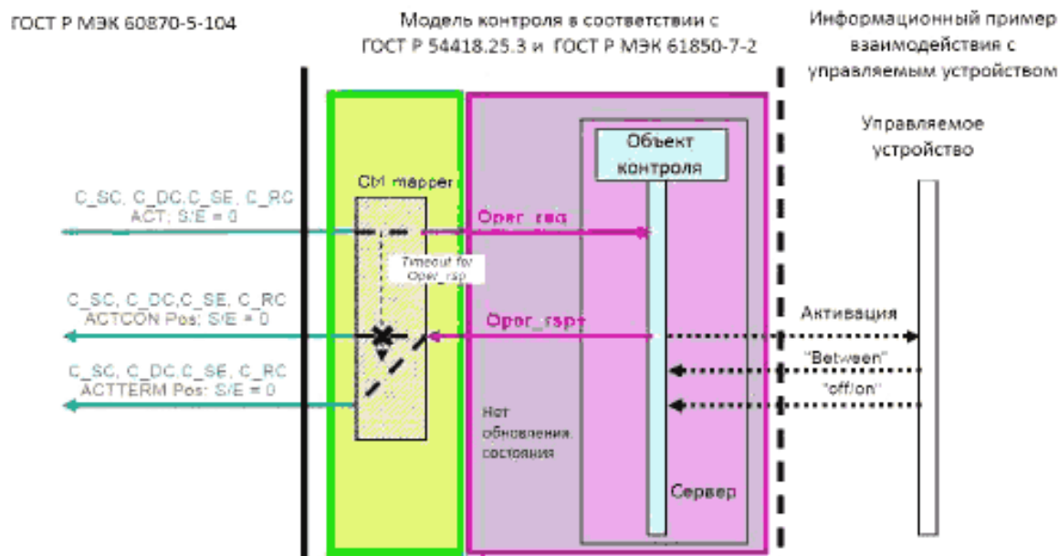
Рисунок Г.6 – Прямое Управление с общей Нормальной Безопасностью без обновления состояния – положительный случай
