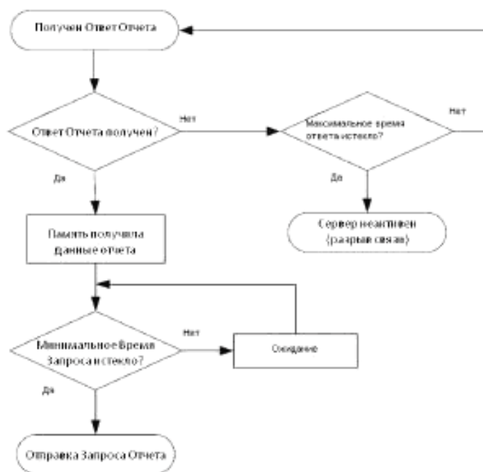
Рисунок А.3 – Поведение клиента в отчетном сервисе (концепция)
