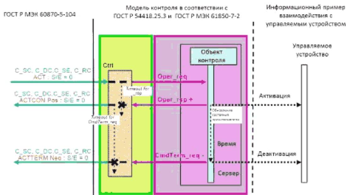
Рисунок Г.8 – Прямое Управление с Улучшенной Безопасностью – отрицательный случай в)
