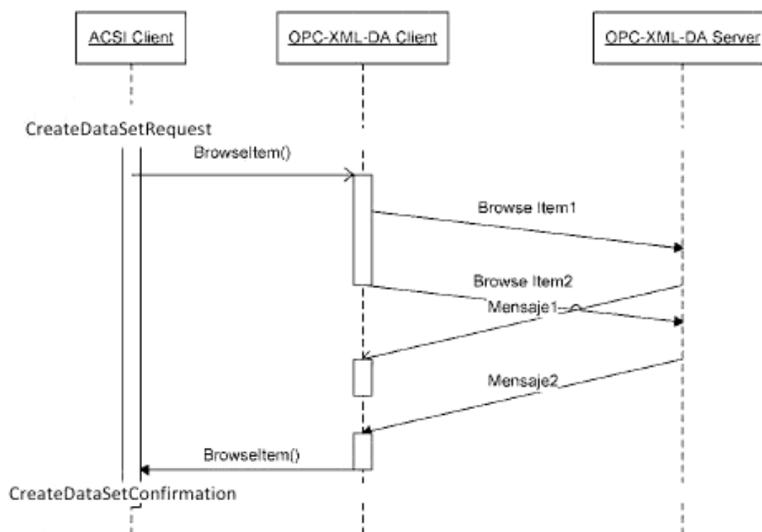
Рисунок Б.3 – последовательность сервисов CreateDataSet
