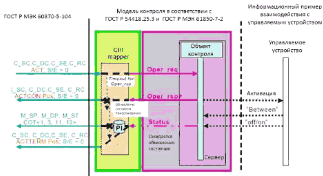
Рисунок Г.2 – Прямое Управление с Нормальной Безопасностью с корректировкой данных – положительный случай
