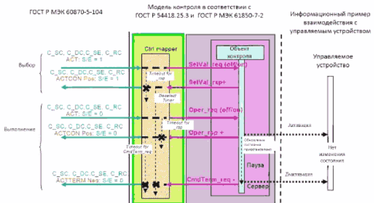
Рисунок Г.15 – SBO-Управление с Улучшенной Безопасностью – отрицательный случай а)
