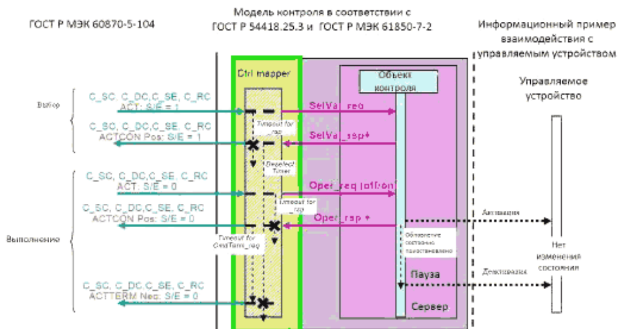
Рисунок Г.16 – SBO-Управление с Улучшенной Безопасностью – отрицательный случай б)
