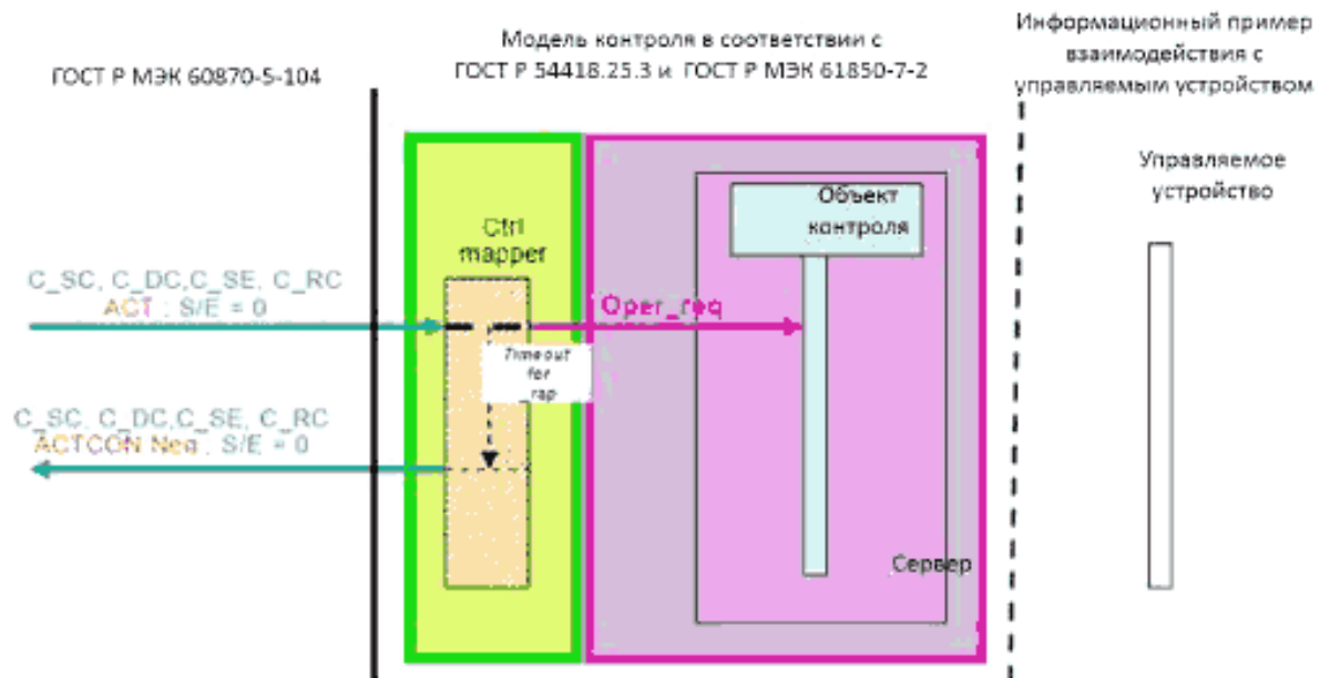
Рисунок Г.3 – Прямое Управление с общей Нормальной Безопасностью – отрицательный случай а)
