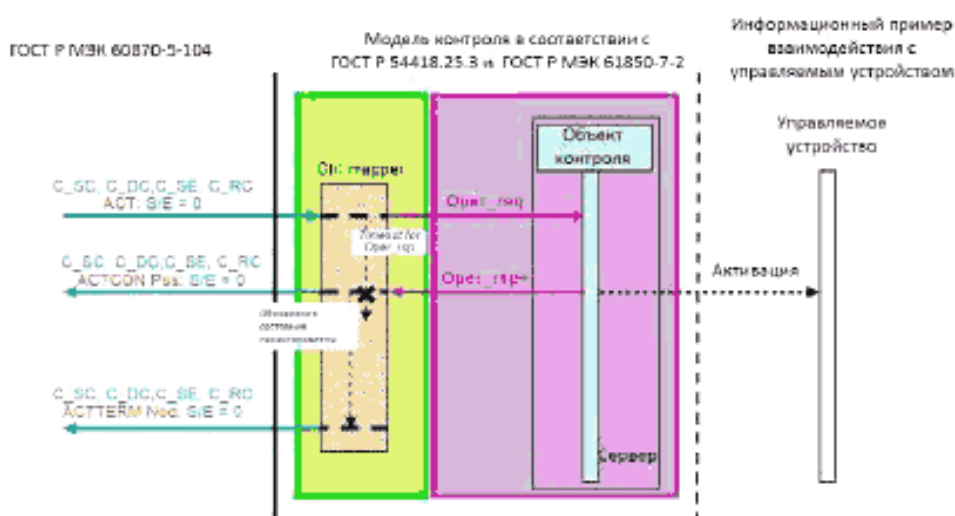
Рисунок Г.5 – Прямое Управление с общей Нормальной Безопасностью с обновлением состояния – отрицательный случай в)
