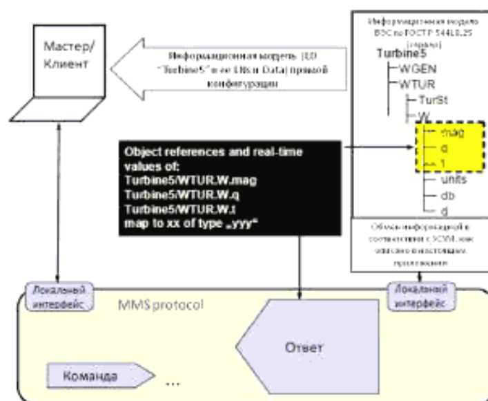
Рисунок В.1 – Архитектура отображения (схематичная)
