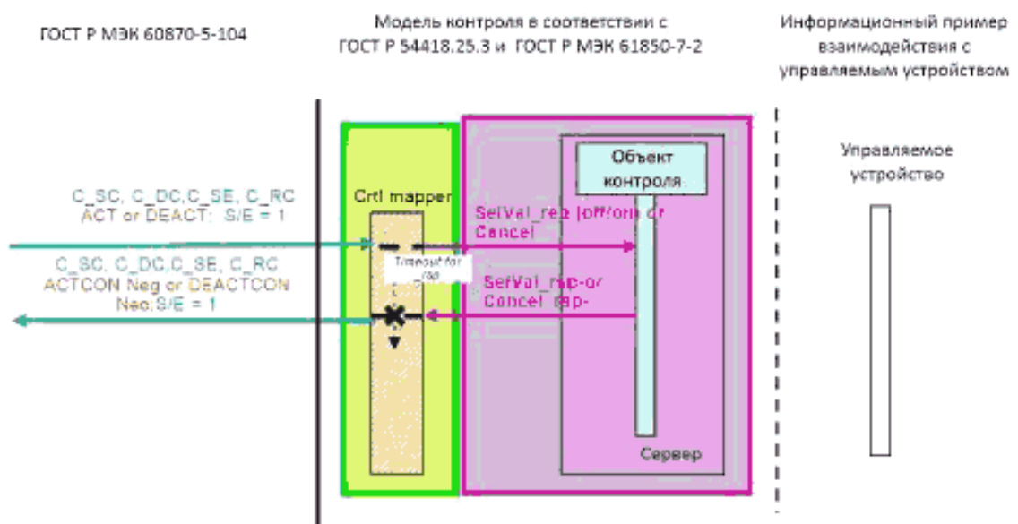
Рисунок Г.12 – SBO-Управление – отрицательный случай б)
