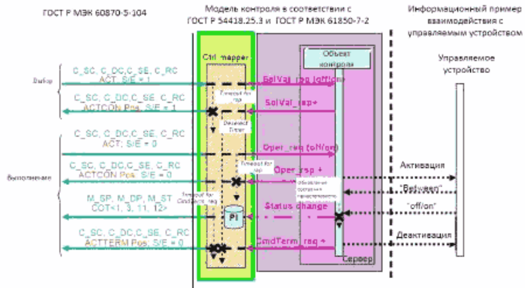
Рисунок Г.14 – SBO-Управление с Улучшенной Безопасностью – положительный случай
