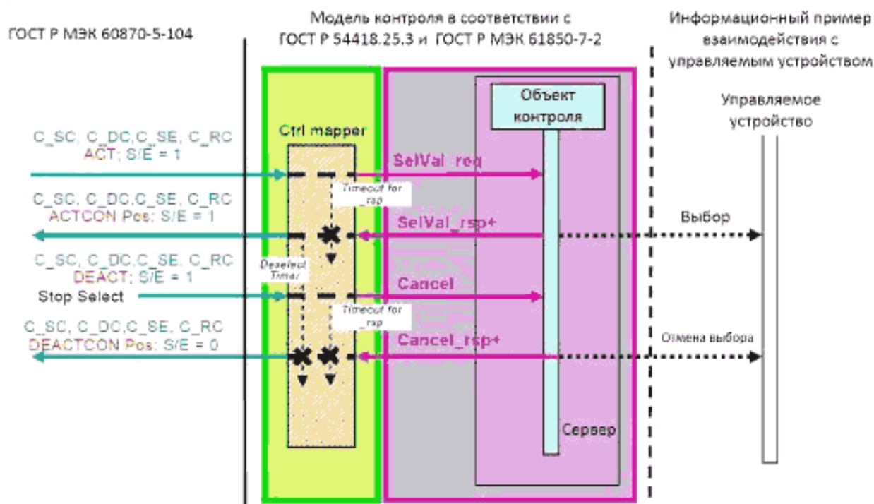
Рисунок Г.10 – SBO-Управление – положительный случай
