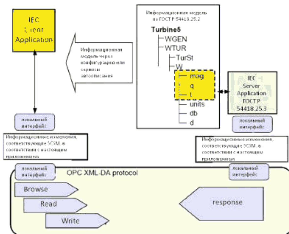
Рисунок Б.1 – Отображение (концептуальное) архитектуры
