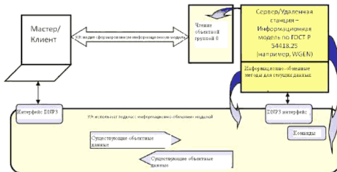
Рисунок Д.1 – Структура отображения (концепция)
