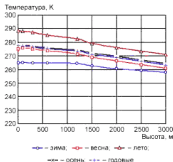
Рисунок В2 — Сезонные отличия высотных профилей температуры Т
