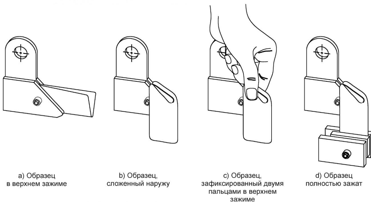
Рисунок 4 — Установка испытуемой пробы
