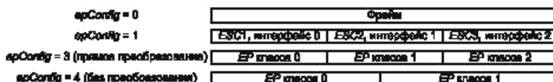
Рисунок 3 – Классы EP для различных значений epConfig
