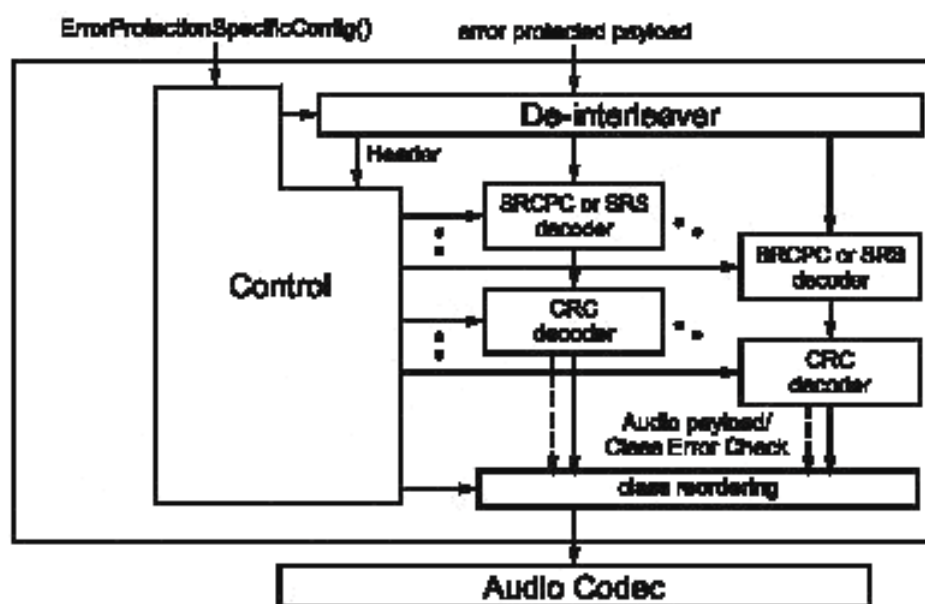
Рисунок 5 - Схема декодера EP
