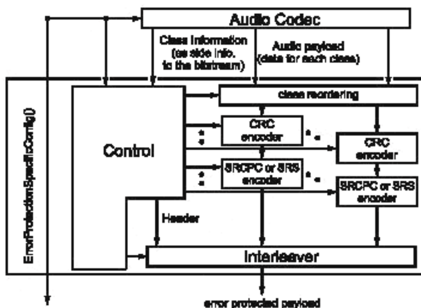
Рисунок 4 - Схема кодера EP
