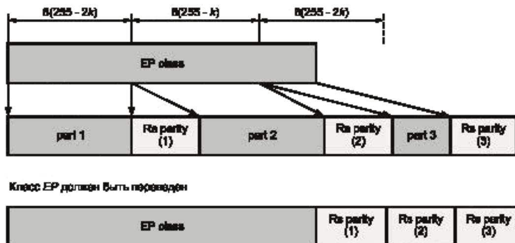
Рисунок 7 – Кодирование RS фрейма EP
