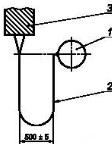
1 — контрольный груз; 2 — свободная петля испытываемого образца; 3 — опора
