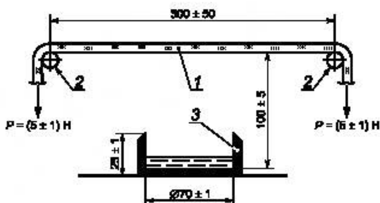
1 — образец веревки; 2 — опоры; 3 — емкость для горючего
