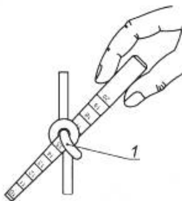
Рисунок 2 — Схема измерения внутреннего диаметра узла
