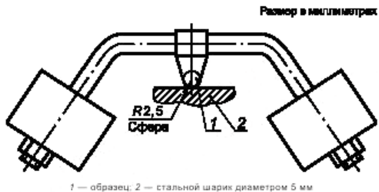
Рисунок 25 — Установка для испытания прочности материалов
