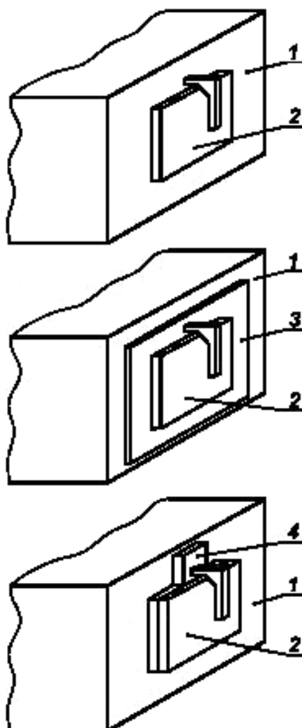
Рисунок 20 — Калибр (толщина около 2 мм) для проверки габаритов крышек для закрывающих пластин
