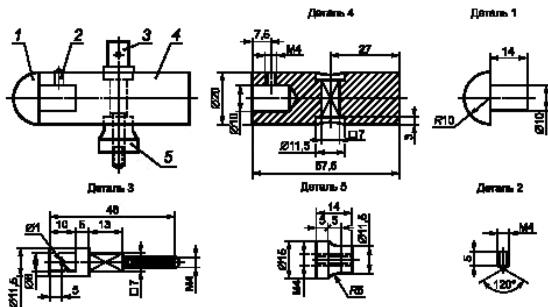
Рисунок 16 — Устройство маятника для испытания на удар
