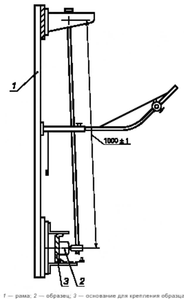
Рисунок 15 — Устройство для испытания на удар
