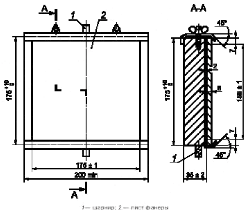
Рисунок 17 — Основание для крепления образца
