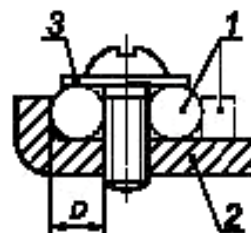
Зажимы, требующие применения прокладок, прижимной пластины или специальной прижимной детали
