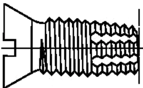
Рисунок 7 — Самонарезающий режущий винт
