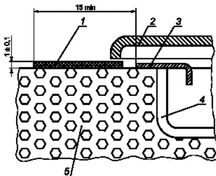
Рисунок 19 — Устройство для испытания крышек и закрывающих пластин
