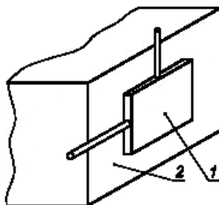
Рисунок 23 — Калибр для проверки пазов, отверстий и обратных конусов
