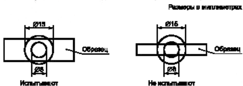
Рисунок 26 — Схема испытания по 24.1.1
