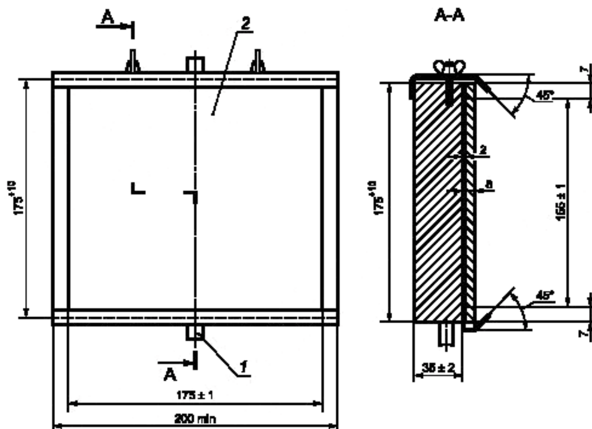
Рисунок 24 — Монтажная опора
