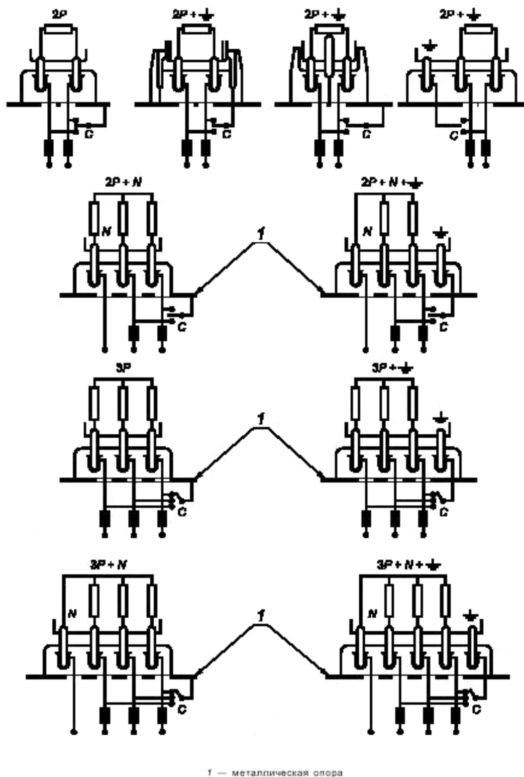
Рисунок 17 — Схема соединения для испытания соединителей на нормальную работу
