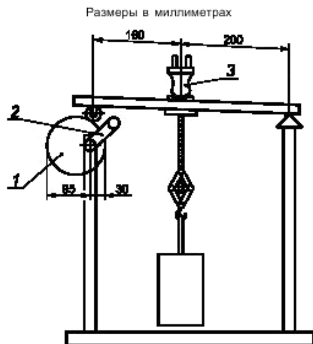
Рисунок 20 — Установка для испытания узла крепления шнура
