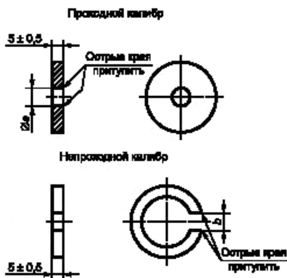
Проверка диаметров штырей вилок
