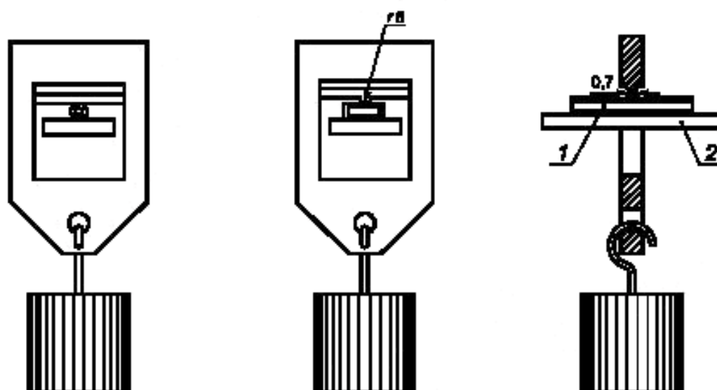
Рисунок 41 — Установка для испытания давлением при высокой температуре
