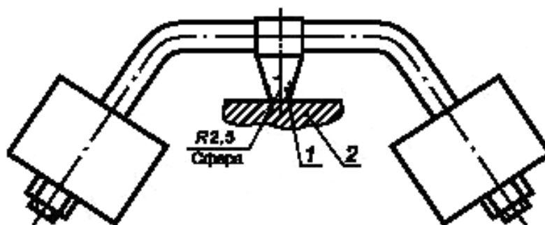
Рисунок 36 — Схема, показывающая направление приложения калибра, изображенного на рисунке 35
