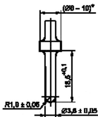
Рисунок ДА.6 — Калибр для проверки контактного нажатия розеток
