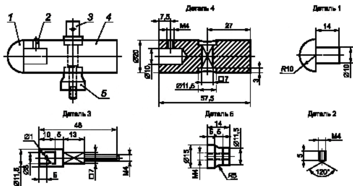
Рисунок 23 — Ударный элемент
