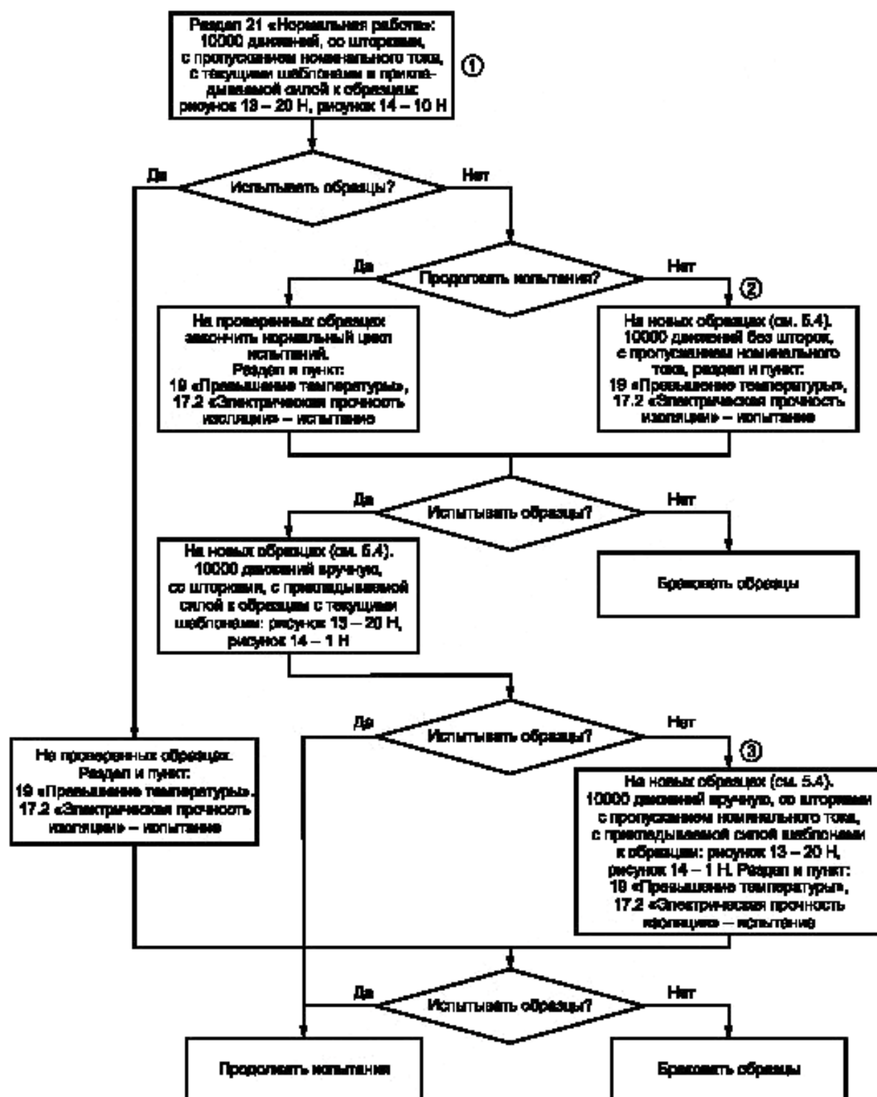
Рисунок 43 — Методика испытаний по разделу 21 «Нормальная работа»
