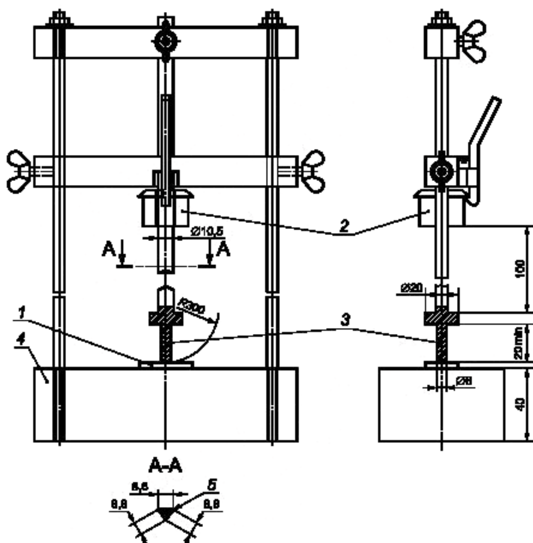
Рисунок 42 — Установка для испытания ударом при низкой температуре
