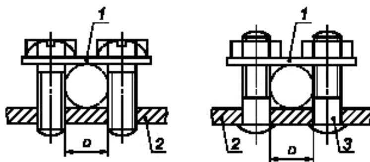
1 — прижимная пластина; 2 — неподвижная деталь; 3 — шпилька; D — место расположения проводника
