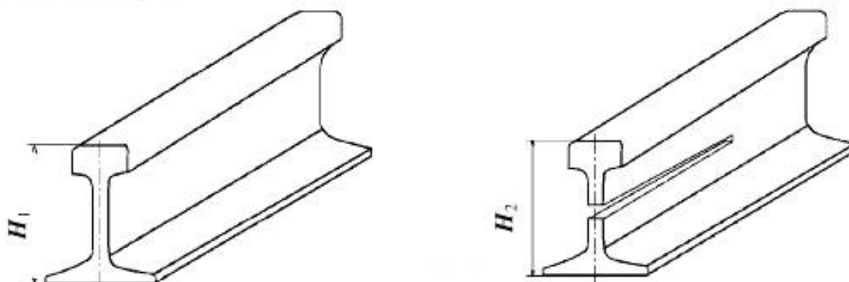
Рисунок 4 – Схема определения остаточных напряжений в шейке рельсов
