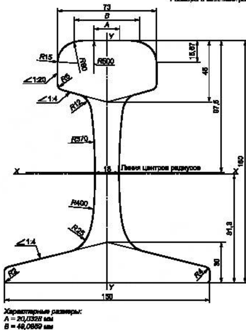
Рисунок А.3 — Рельс типа РП65
