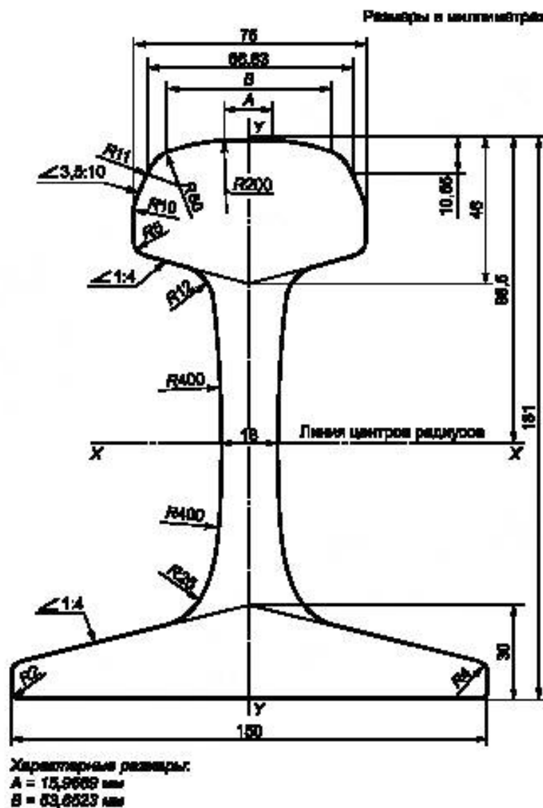
Рисунок А.4 — Рельс типа РП65К
