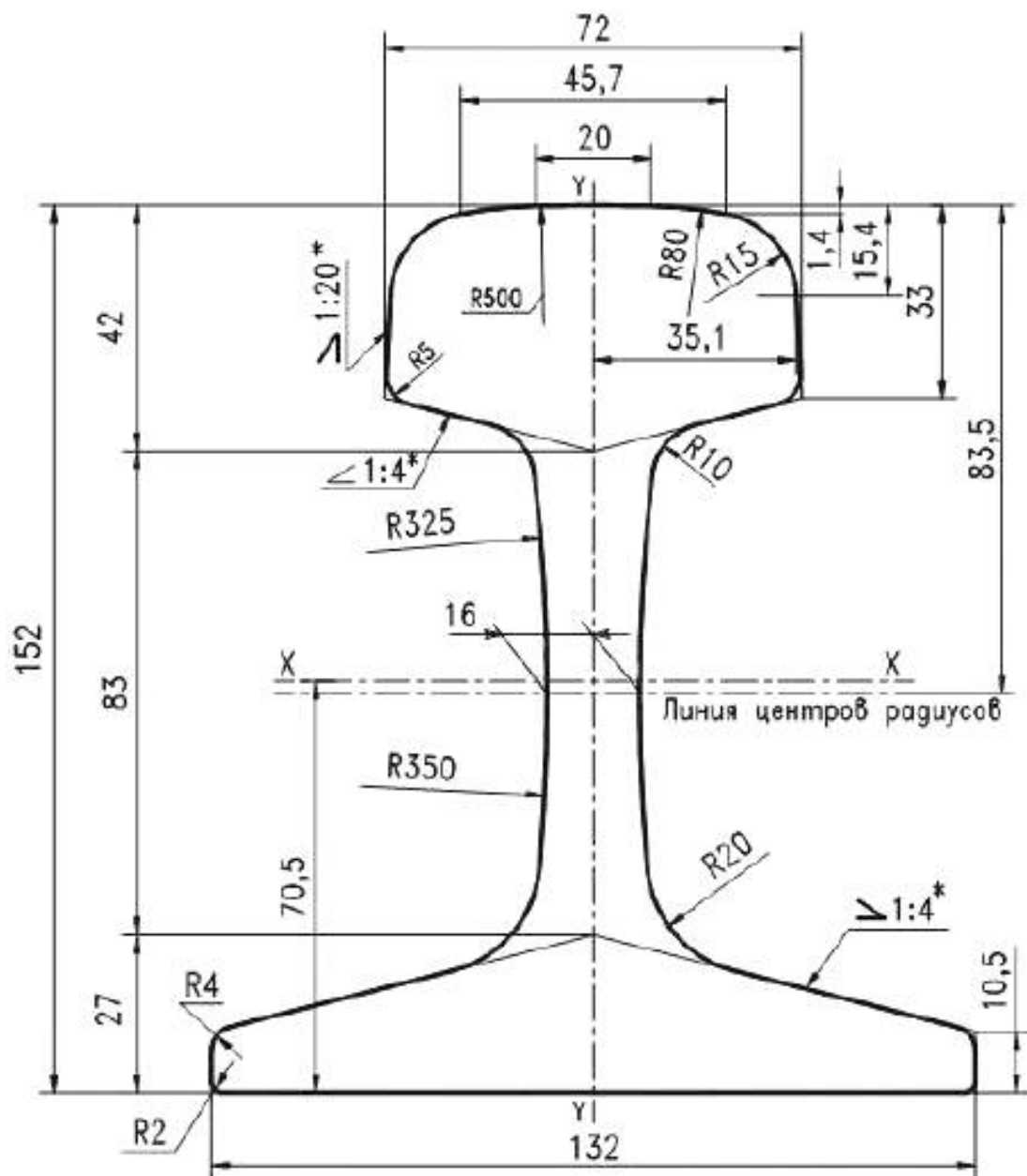
Рисунок А.1 – Рельс типа РП150
