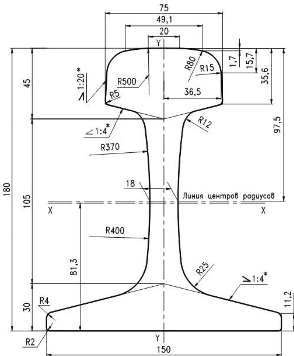
Рисунок А.3 – Рельс типа РП65
