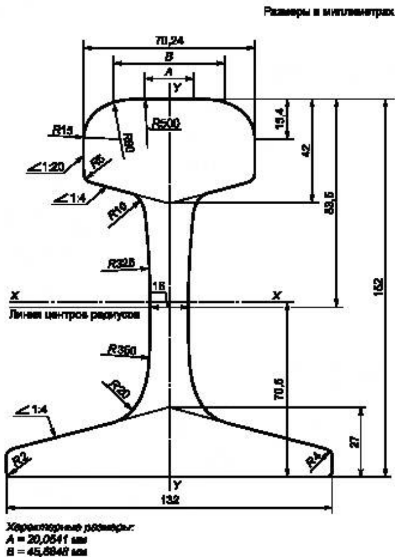
Рисунок А.1 — Рельс типа РГ50
