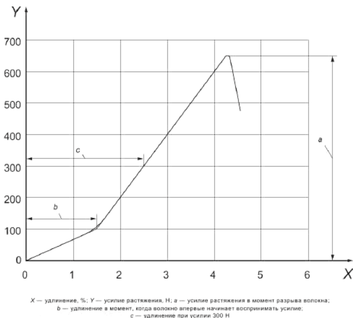
Рисунок 1 — Пример кривой усилие/удлинение
