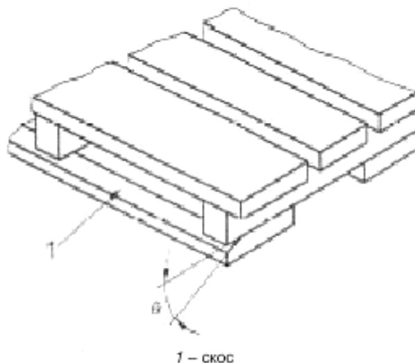
Рисунок 48 – Сплошной скос
