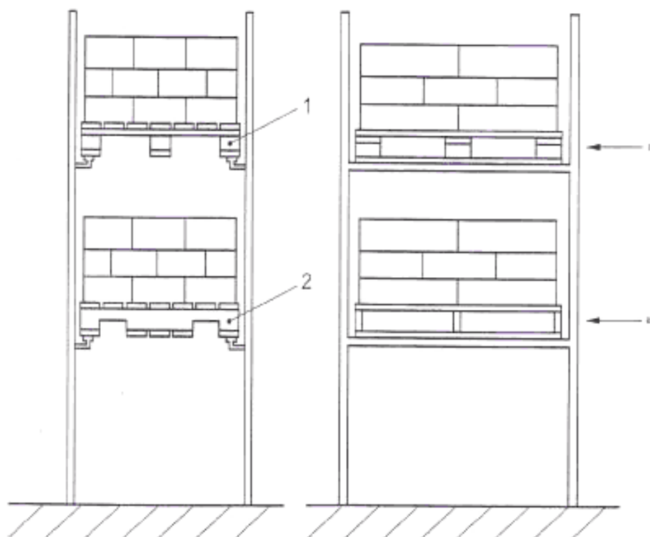
1 – четырехзаходный поддон со свободным заходом; 2 – поддон с продольной выемкой; а – сторона загрузки
