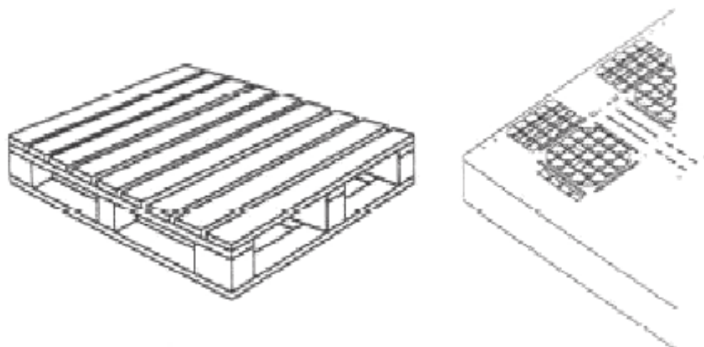
Рисунок 9 – Поддоны четырехзаходные
