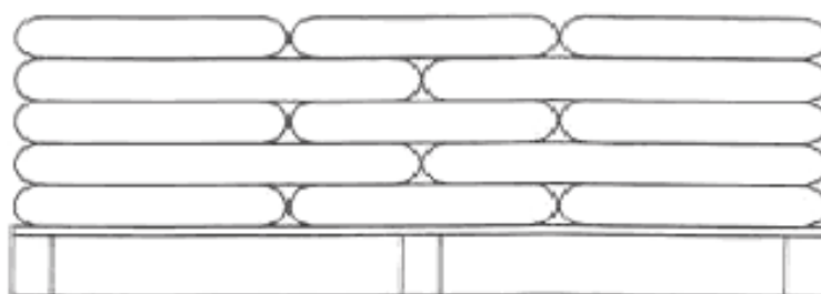
Рисунок 2 — Равномерно распределенный закрепленный груз
