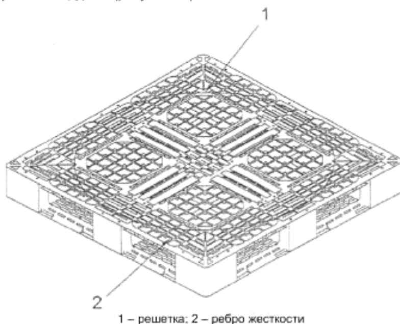
Рисунок 62 – Дополнительные элементы: решетка и ребра жесткости
