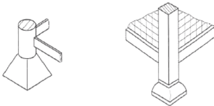
Рисунок 59 – Чашечная опора
