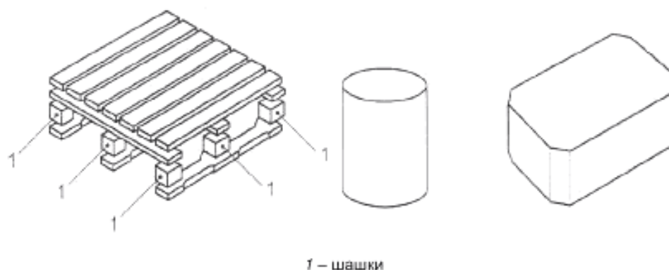
Рисунок 55 – Шашки
