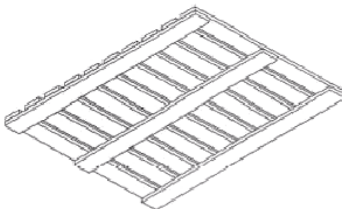
Рисунок 35 – Верхний настил поддона с нижними деталями (мат)
