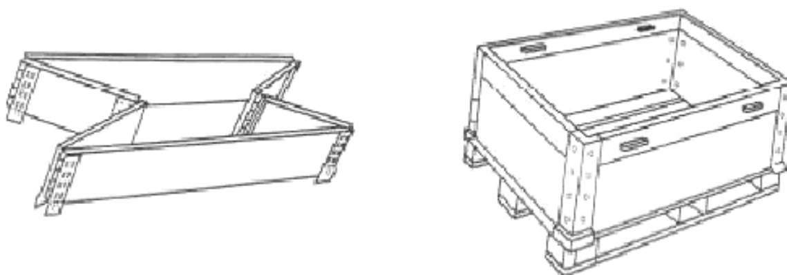
Рисунок 31 – Съемный бортик
