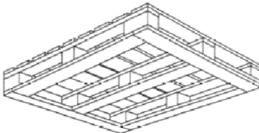
Рисунок 13 — Поддон с нижним настилом по периметру
