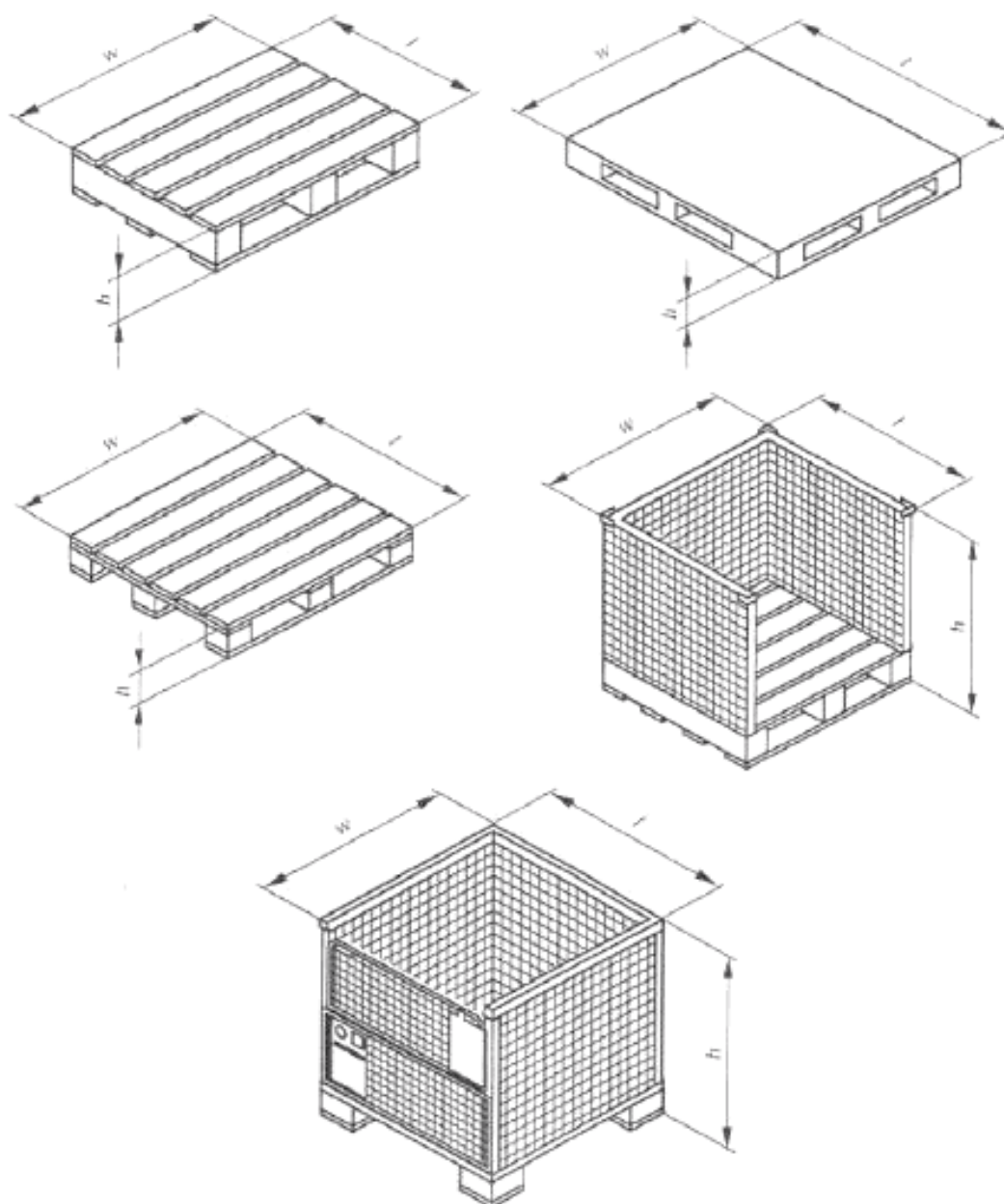
Рисунок 72 – Условные обозначения размеров поддонов
