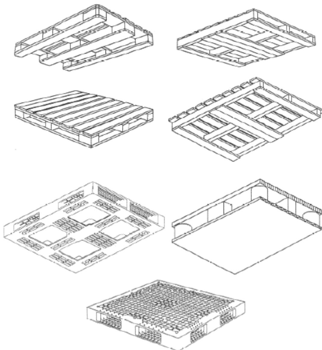
Рисунок 5 – Двухнастильные поддоны
