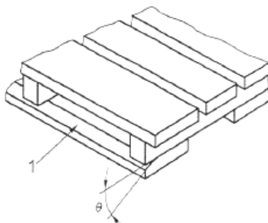
Рисунок 49 – Частичный скос
