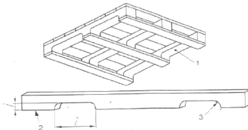
1 – выемка; 2 – опорная часть продольного бруса; 3 – радиус закругления; а – глубина выемки; б – длина выемки.
