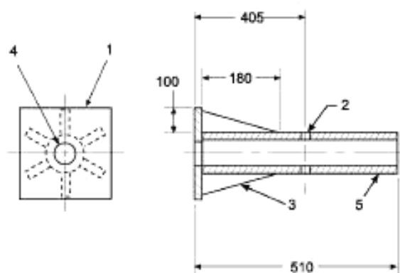
1 — квадратная стальная плита со стороной 300 мм и толщиной 12,7 мм; 2 — сквозное отверстие диаметром 12 мм; 3 — шесть стальных накладок толщиной 10 мм, приваренных к плите и трубе; 4 — отверстие диаметром (54 \pm 3) мм; 5 — стальная труба диаметром 63 мм, приваренная к плите.
