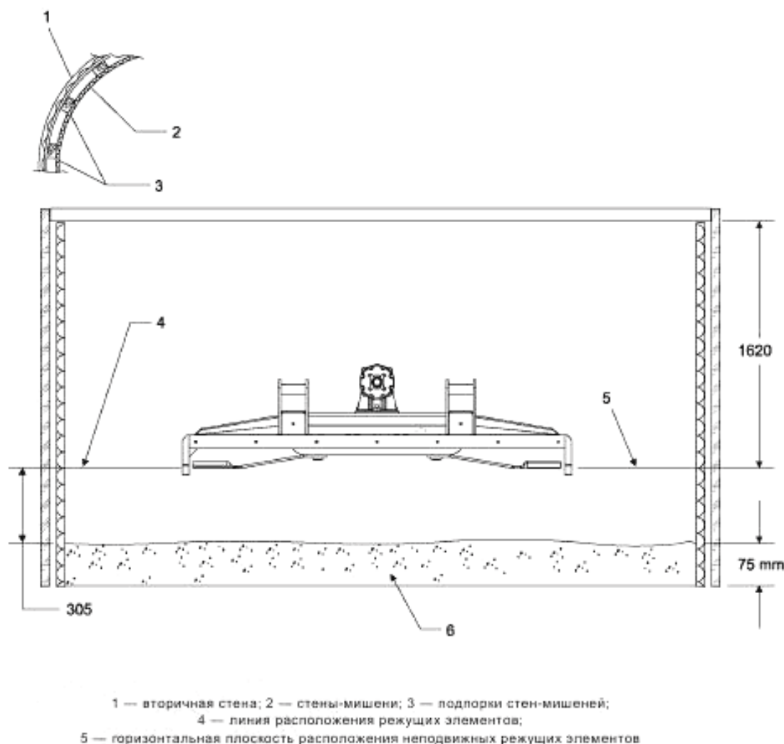
Рисунок 9 — Конструкция стен-мишеней и поперечное сечение
